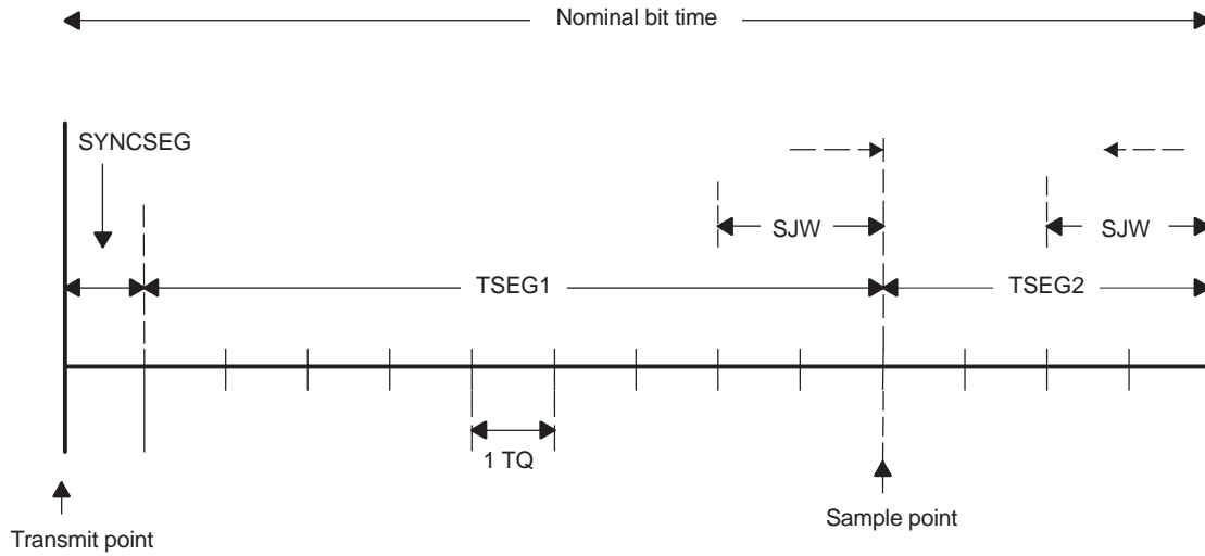
图 42. CAN 位时序
