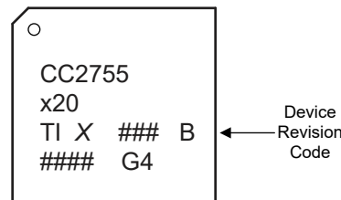
图 2-1. 封装符号
