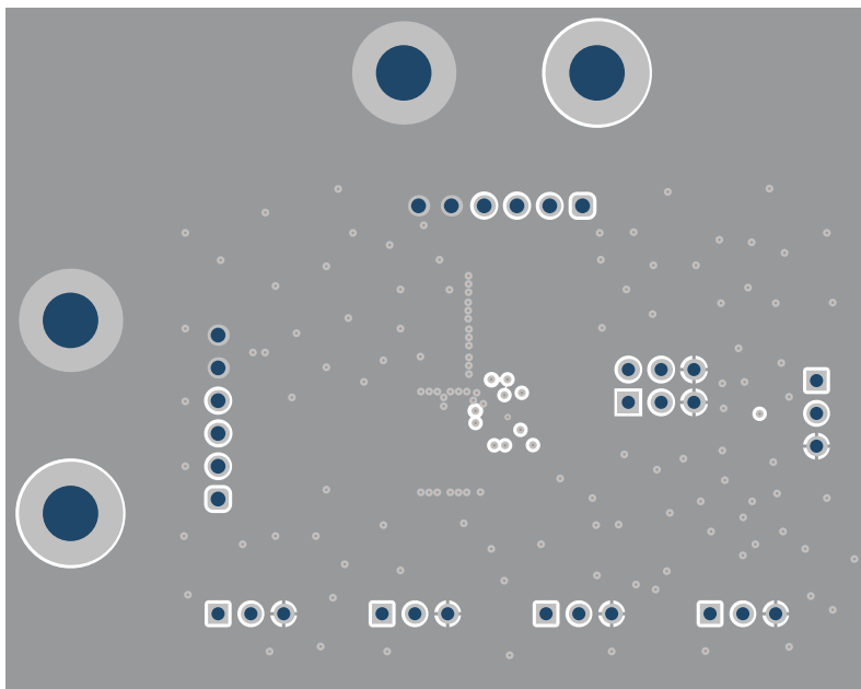
图 3-4. 信号层 1
