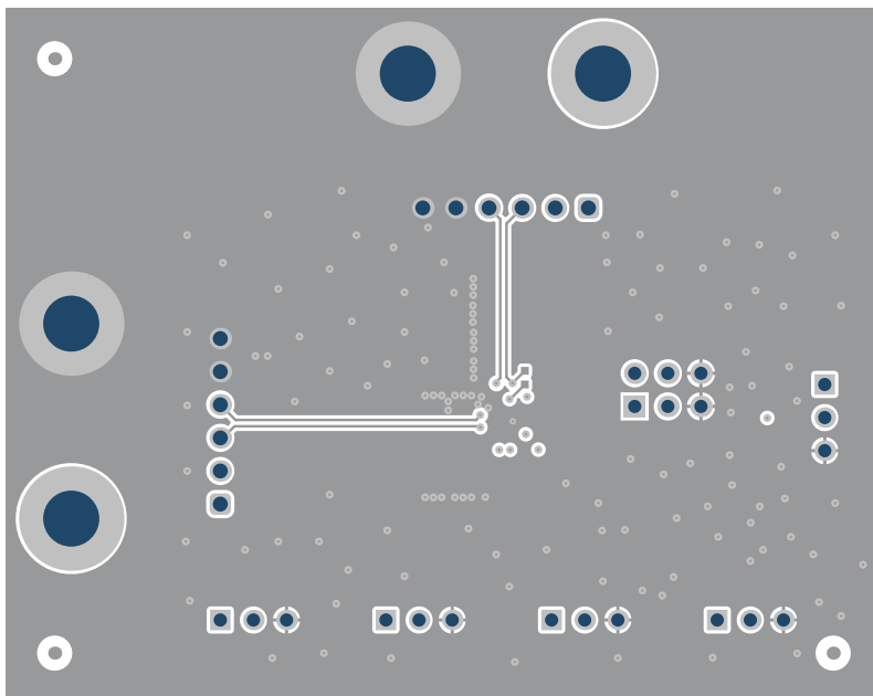
图 3-6. 底层
