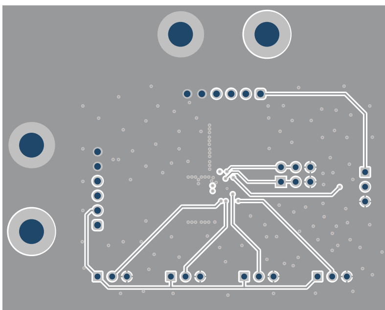
图 3-5. 信号层 2
