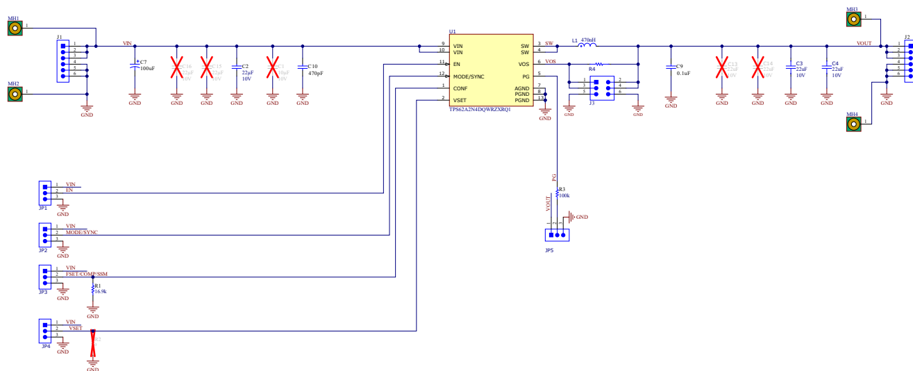
图 3-1. TPS62A204QEVM-116 原理图
