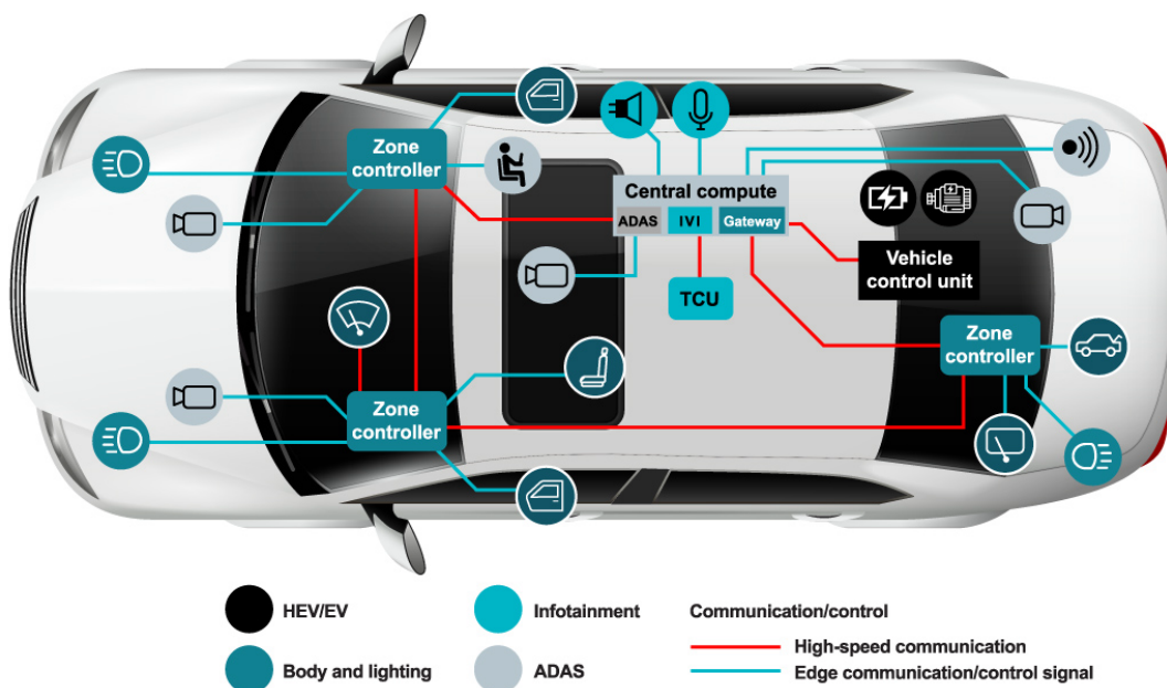
图 2. 软件定义车辆内中央计算架构和互联系统的简化概述
