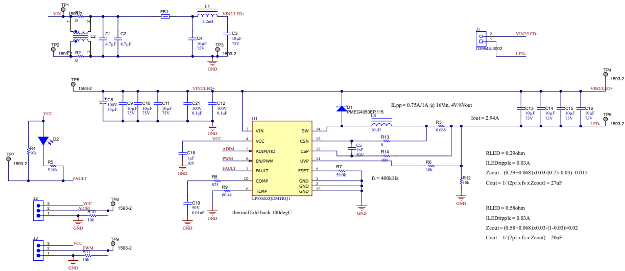
图 3-1. LP8868ZQ1EVM 原理图
