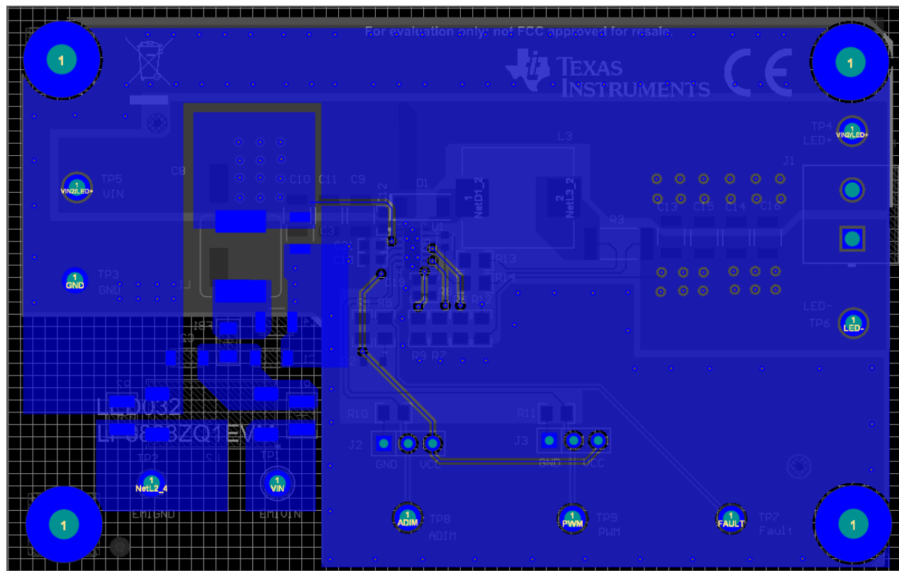
图 3-5. LP8868ZQ1EVM 底层
