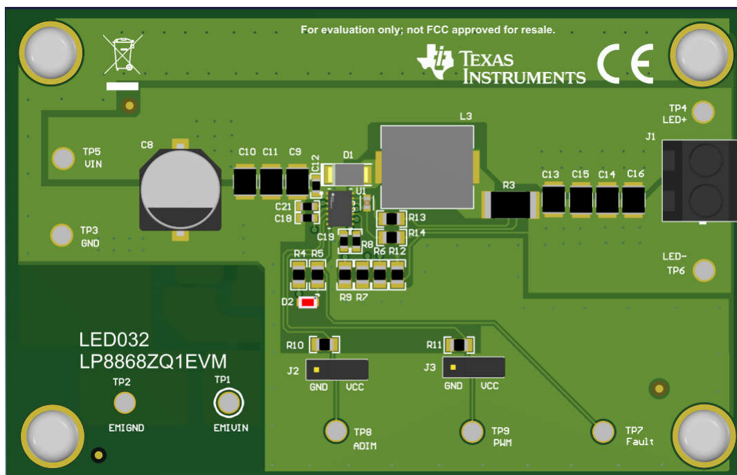
图 1-1. LP8868ZQ1EVM 套件
