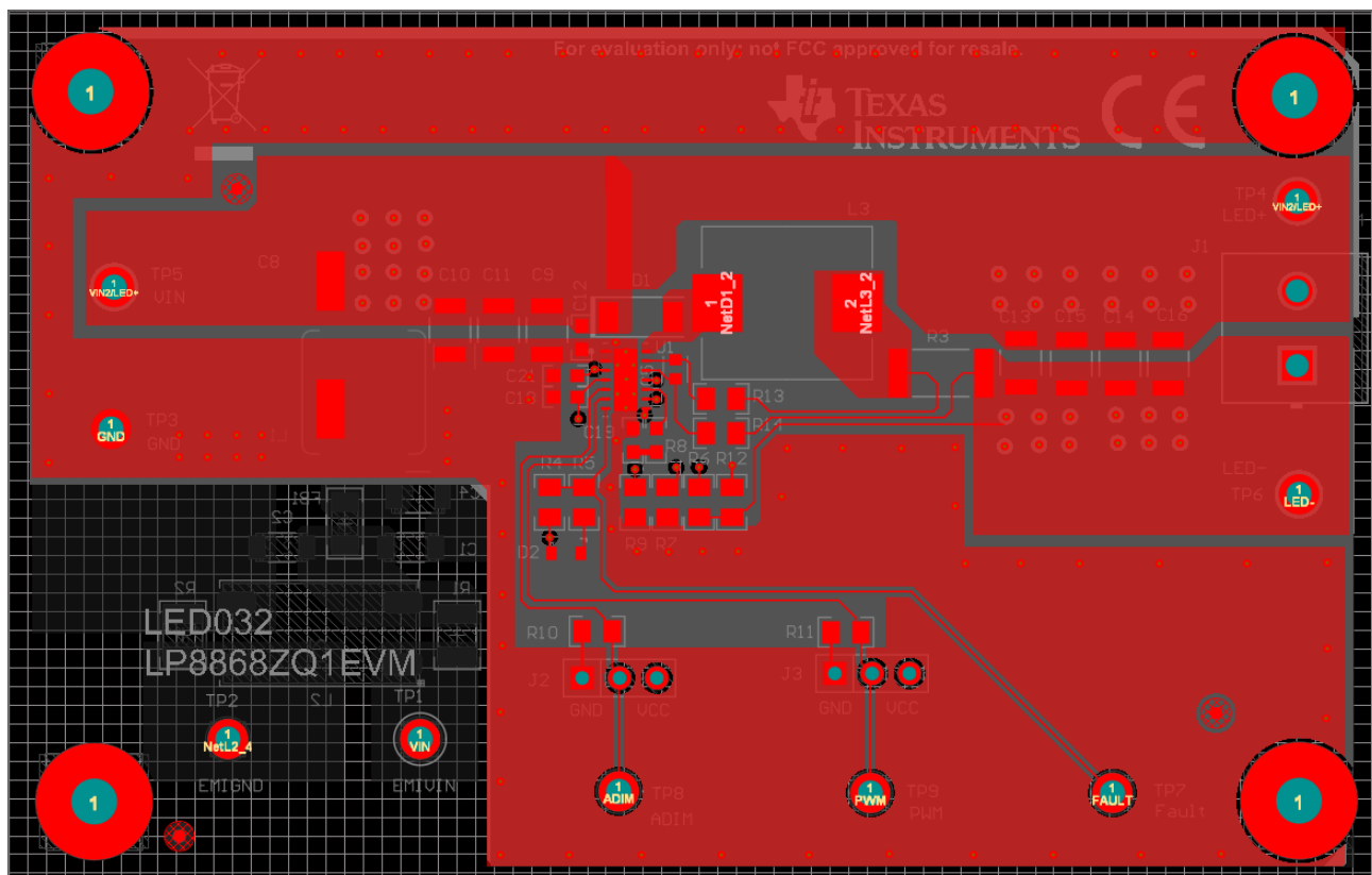
图 3-2. LP8868ZQ1EVM 顶层
