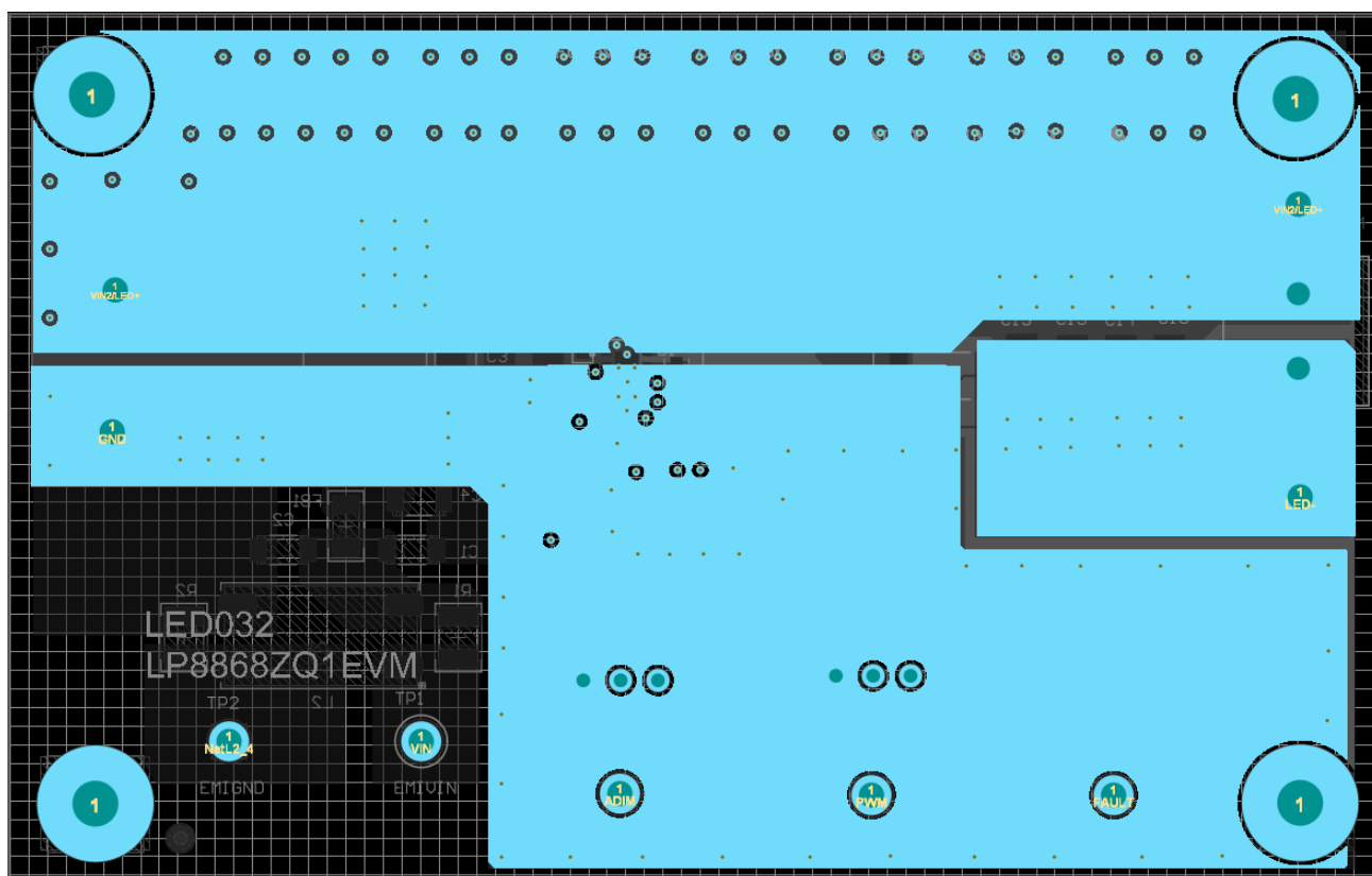
图 3-4. LP8868ZQ1EVM 内层 2
