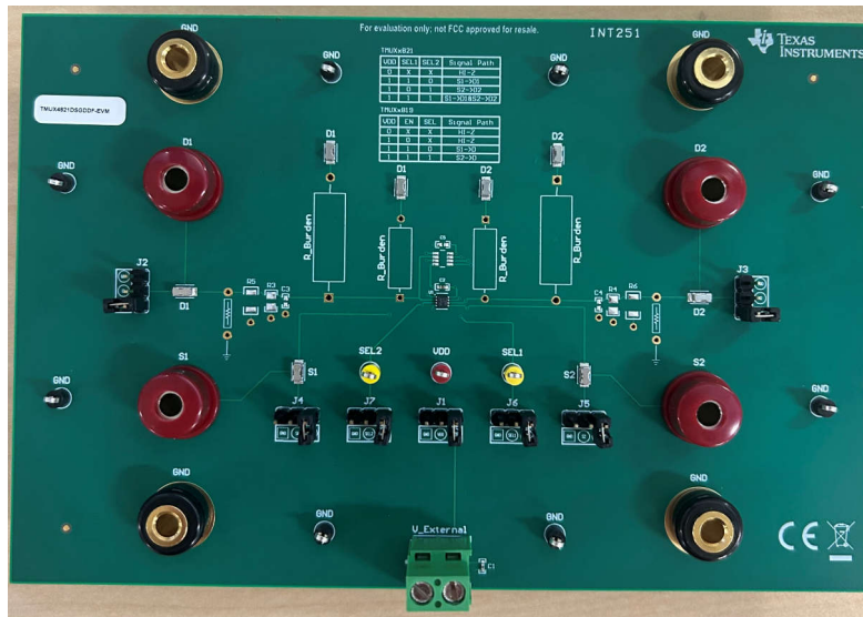
TMUX28XX-DSG-DDF-EVM (顶视图)
