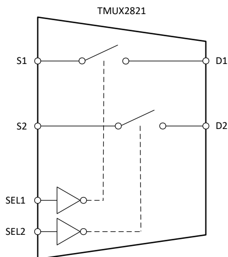
图 1-1. TMUX2821 简化电路
