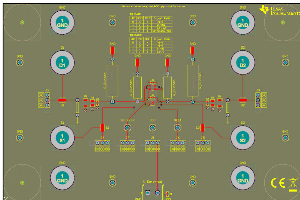
图 3-2. TMUX28XX-DSG-DDF-EVM 顶层布局
