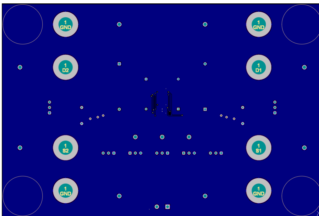
图 3-3. TMUX28XX-DSG-DDF-EVM 底层布局
