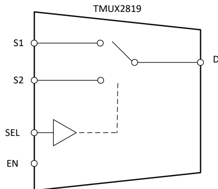
图 1-2. TMUX2819 简化电路
