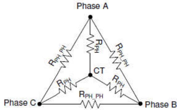
图 6-3. 电阻测量
