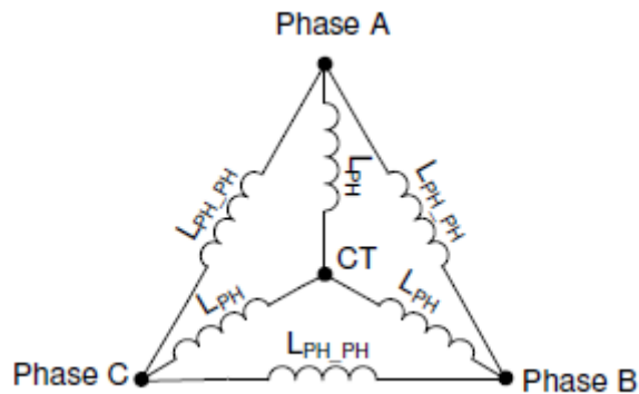
图 6-4. 电感测量
