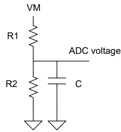
图 2-3. ADC 分压器
