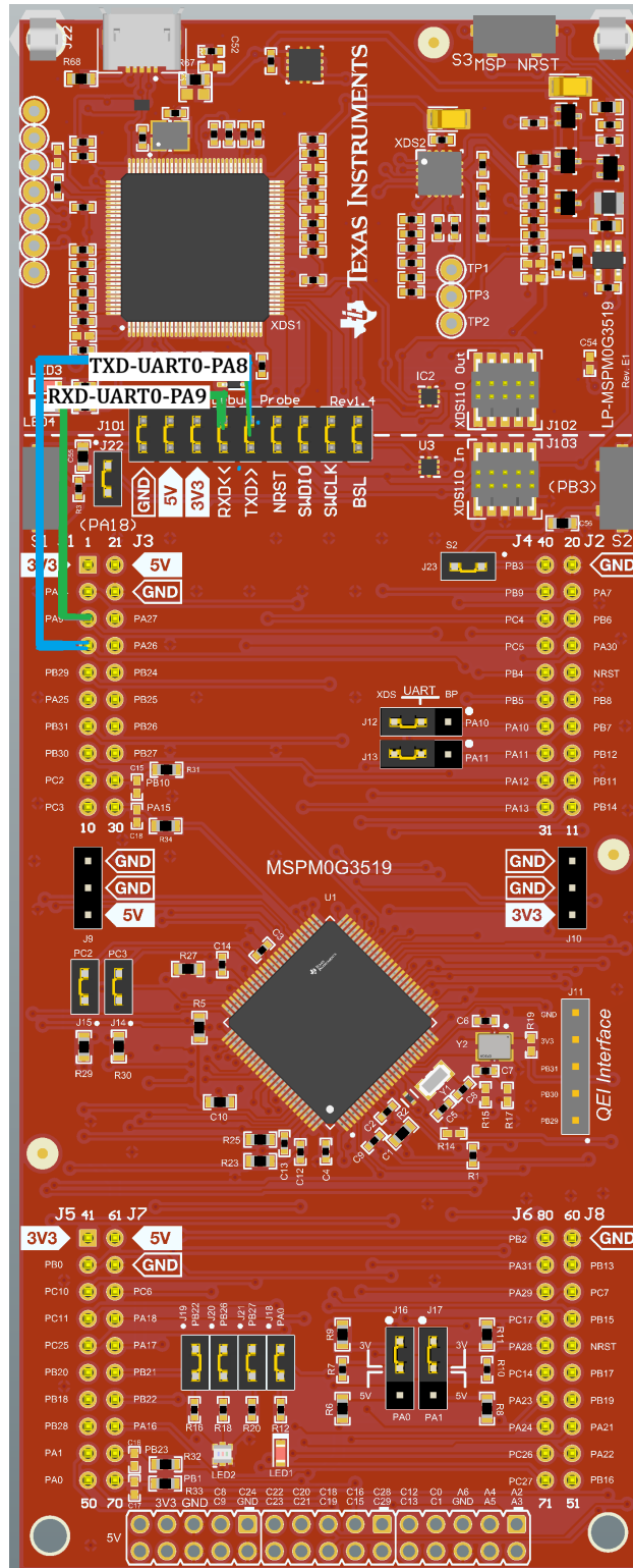
图 2-6. LP-MSPM0G3519 反向通道连接到 UART0
