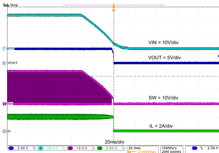
图 3-5. TPS542021EVM 相对于 V_{IN} 的关断
