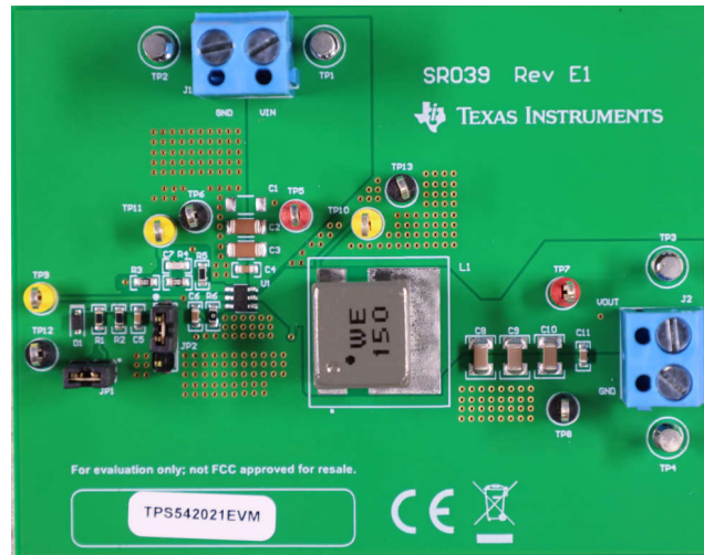
TPS542021EVM ( 顶视图 )
