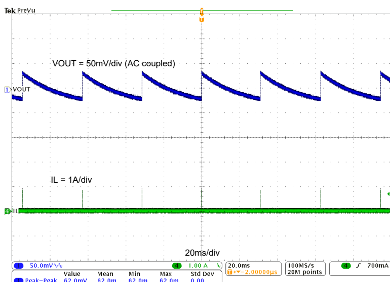
图 3-9. TPS542021EVM 输出电压纹波, I_{OUT} = 0A
