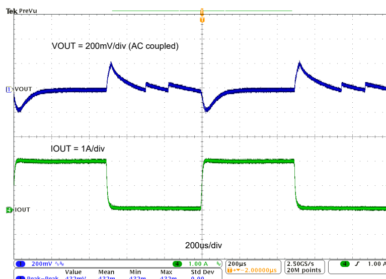
图 3-1. TPS542021EVM 负载瞬态响应, 0A 至 2A 负载阶跃
