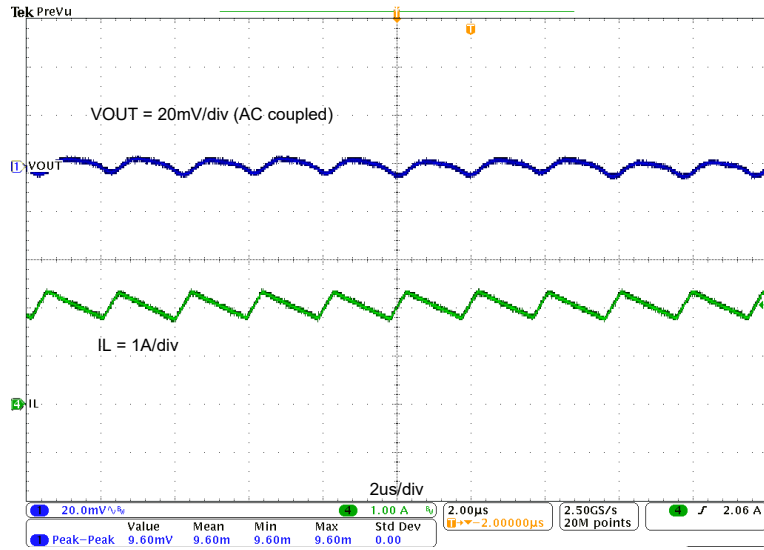
图 3-6. TPS542021EVM 输出电压纹波， I_{OUT} = 2A
