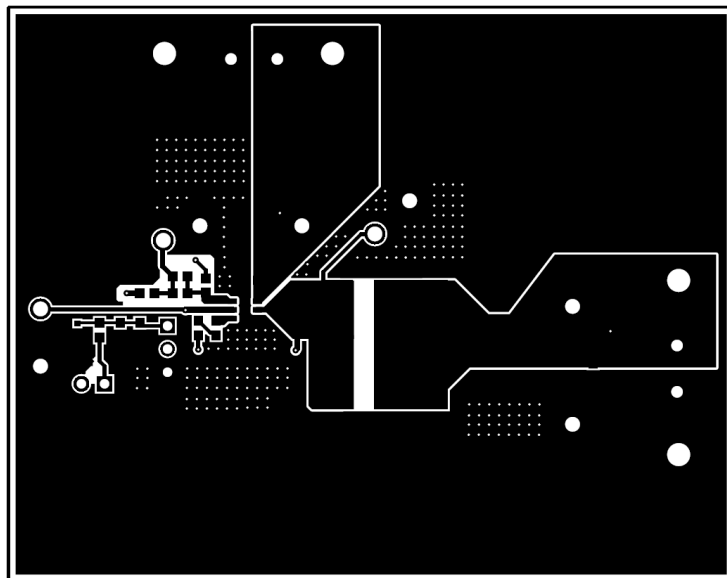
图 4-3. TPS542021EVM 顶层
