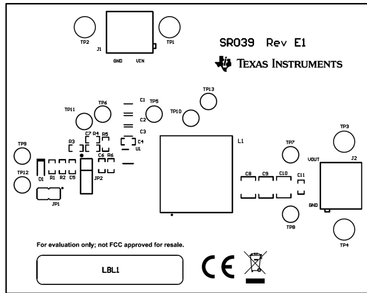
图 4-2. TPS542021EVM 顶层装配图
