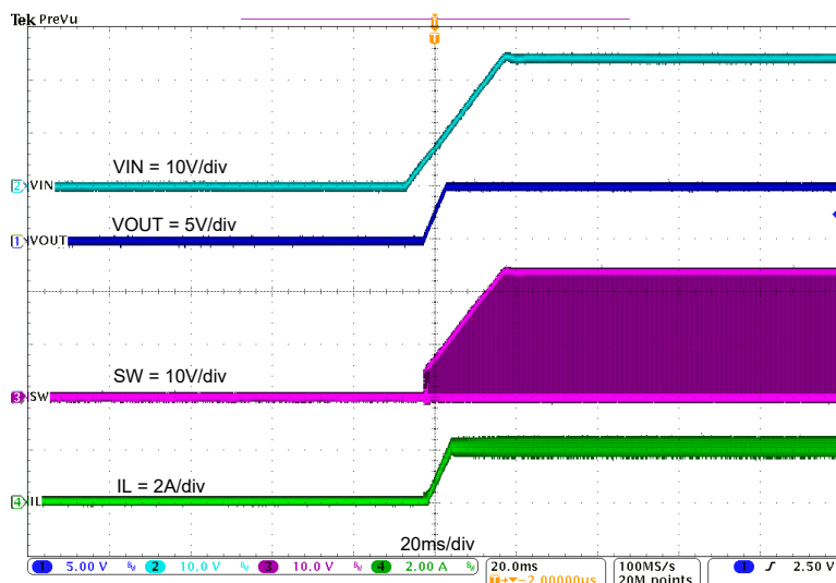
图 3-4. TPS542021EVM 相对于 V_{IN} 的启动
