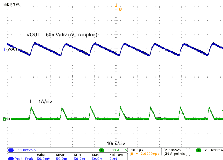
图 3-7. TPS542021EVM 输出电压纹波， I_{OUT} = 0.1A
