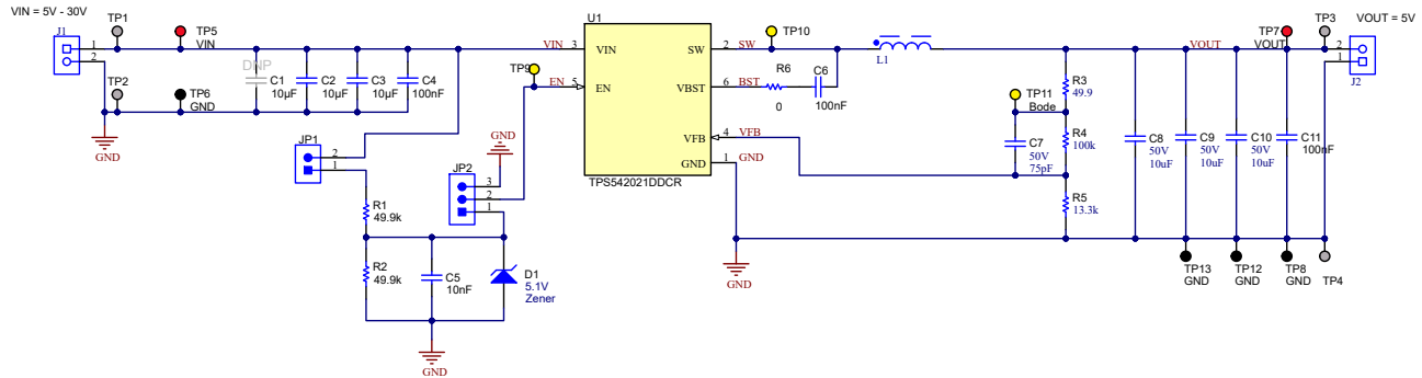
图 4-1. TPS542021EVM 原理图
