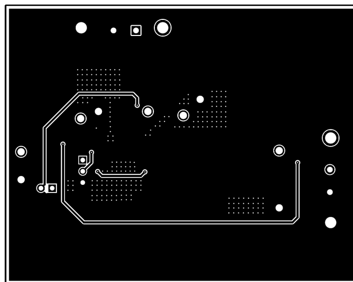
图 4-4. TPS542021EVM 底层
