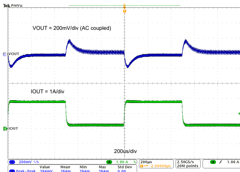
图 3-2. TPS542021EVM 负载瞬态响应，0.2A 至 1.8A 负载阶跃
