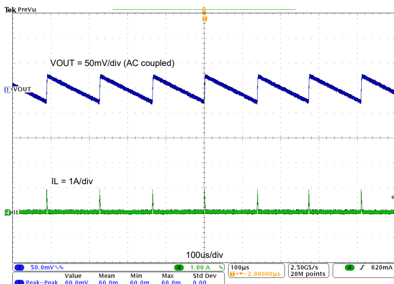
图 3-8. TPS542021EVM 输出电压纹波, I_{OUT} = 0.01A
