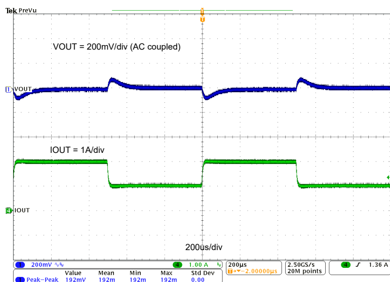
图 3-3. TPS542021EVM 负载瞬态响应，1A 至 2A 负载阶跃
