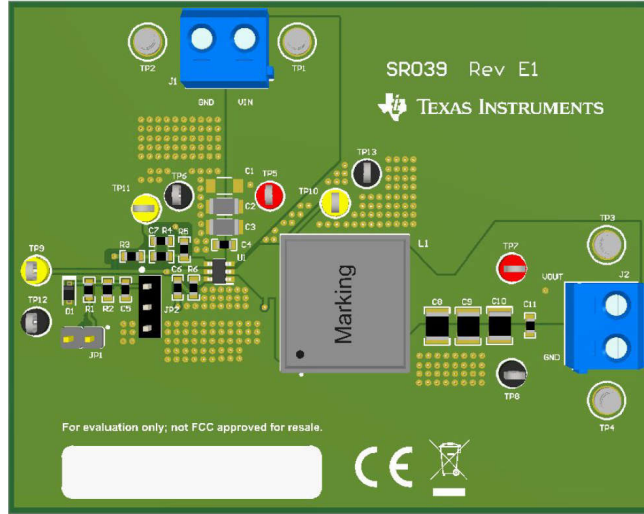
图 2-1. TPS542021EVM 连接器和跳线布置
