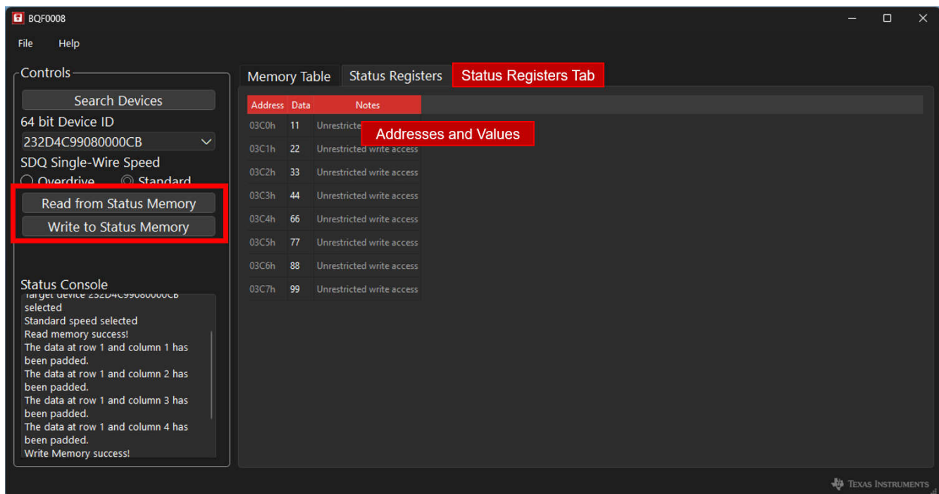
图 3-16. 状态寄存器表和控件
