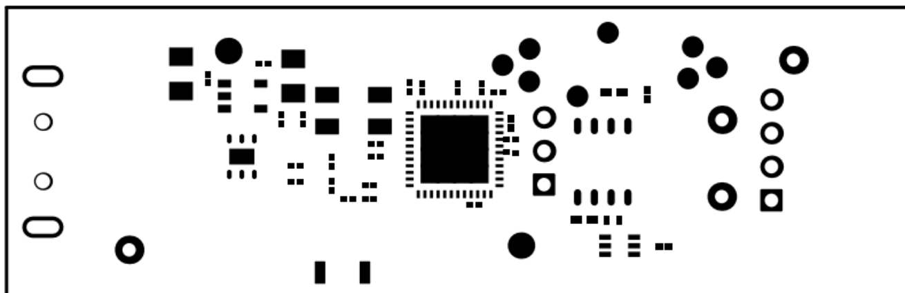
图 4-6. BQF0008EVM 阻焊层 (底部)
