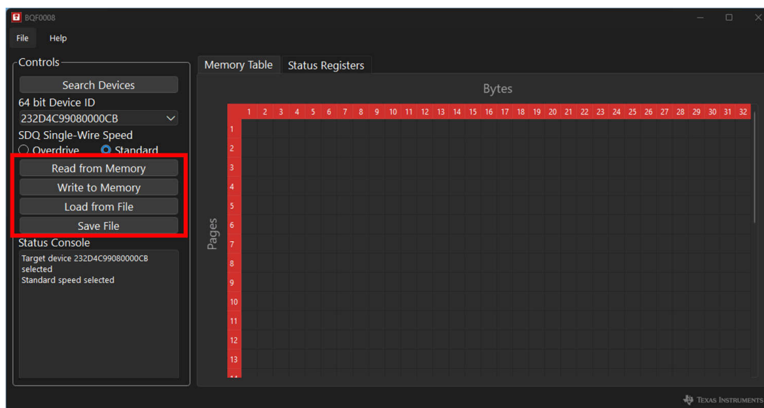
图 3-10. 存储器表控件
