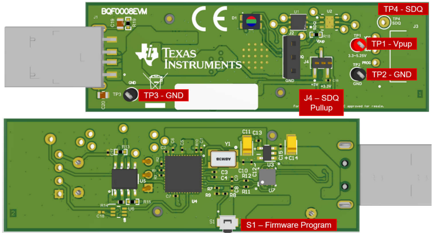
图 2-1. BQF0008EVM 测试点和开关
