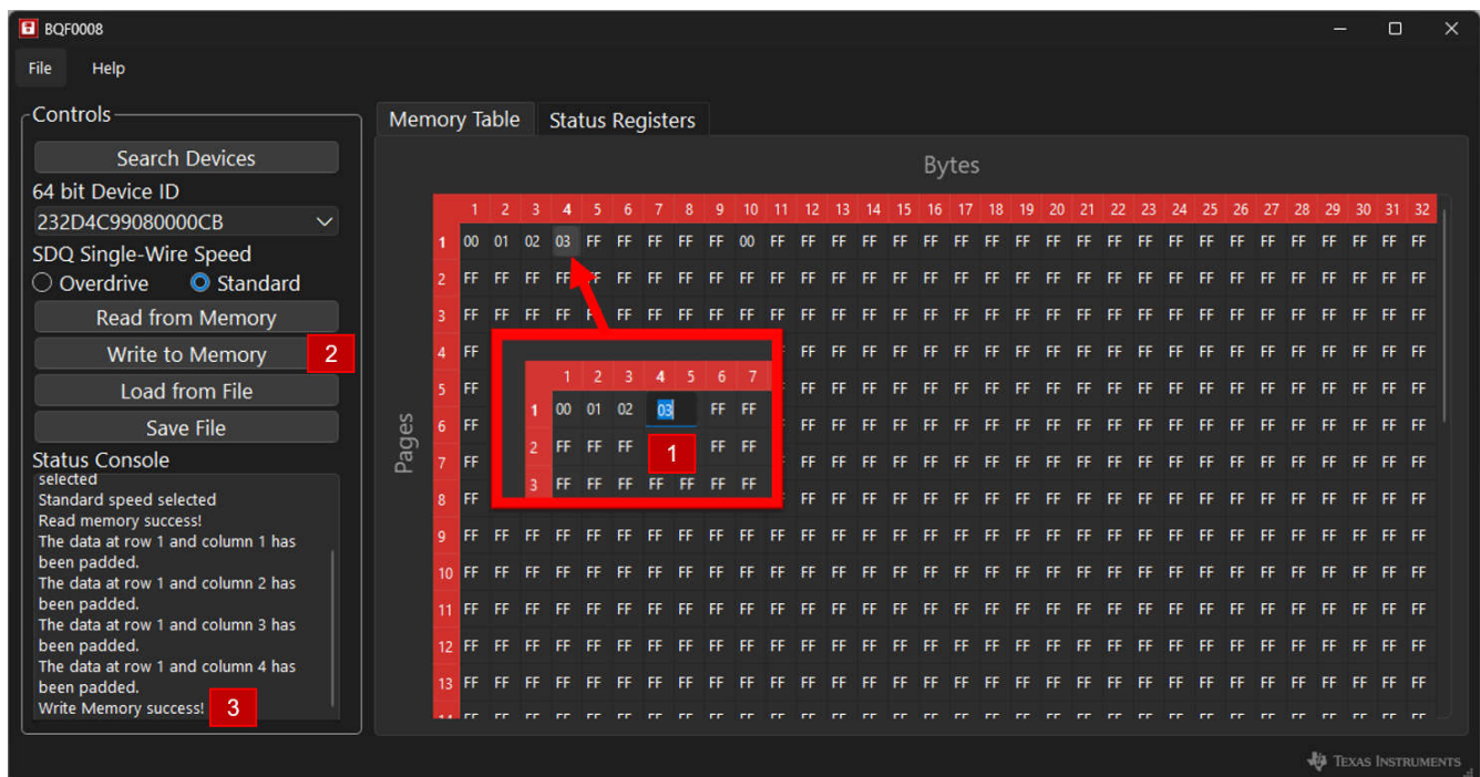
图 3-12. 写入到存储器
