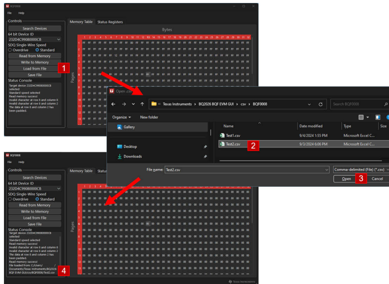
图 3-13. 文件加载过程
