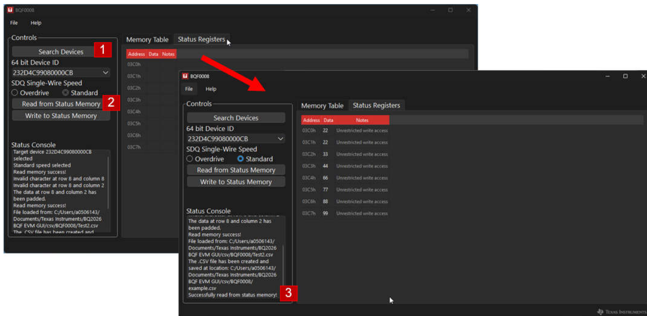
图 3-17. 从状态存储器中读取
