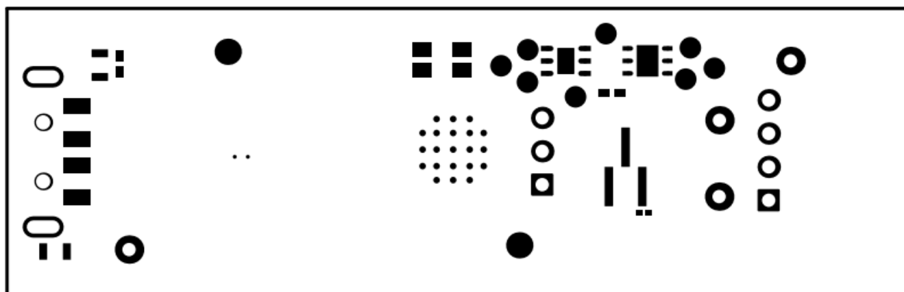
图 4-3. BQF0008EVM 阻焊层 (顶部)
