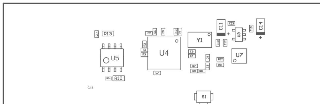
图 4-9. PCB 装配图 ( 底视图 )
