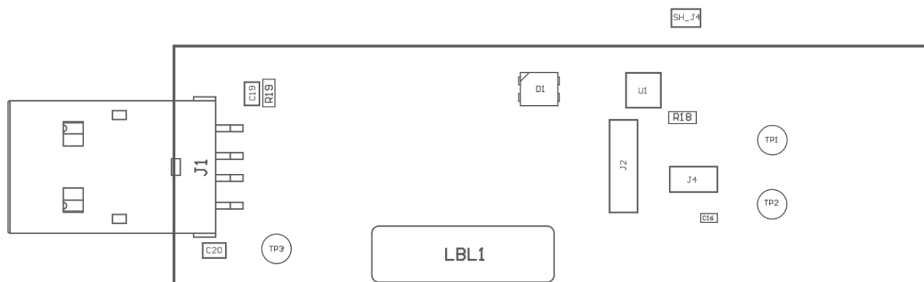
图 4-8. PCB 装配图 ( 顶视图 )
