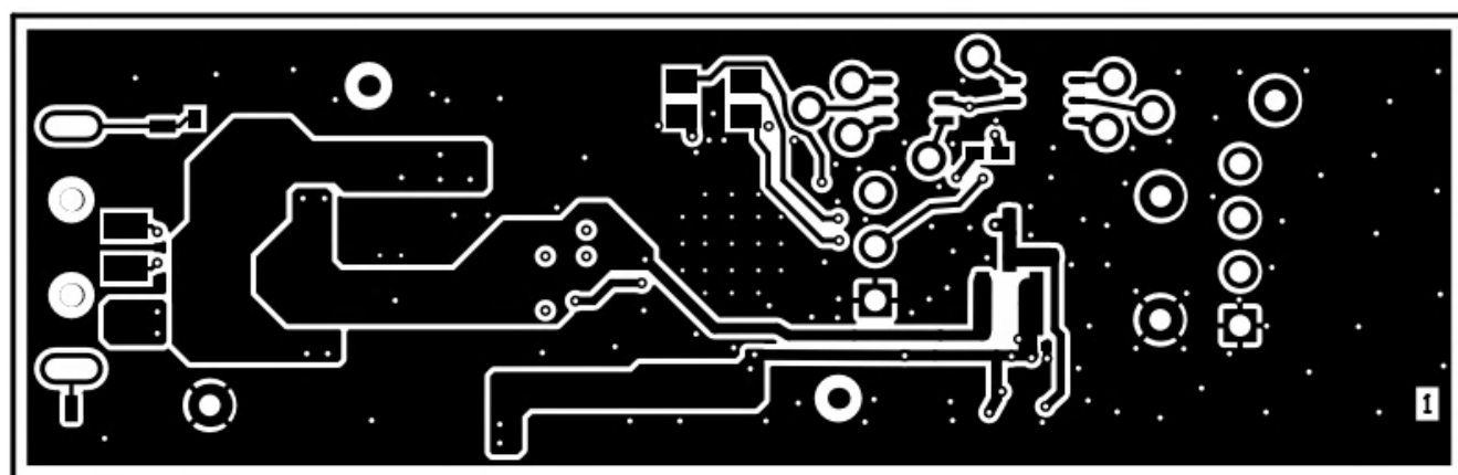
图 4-4. BQF0008EVM 覆铜 (顶部)
