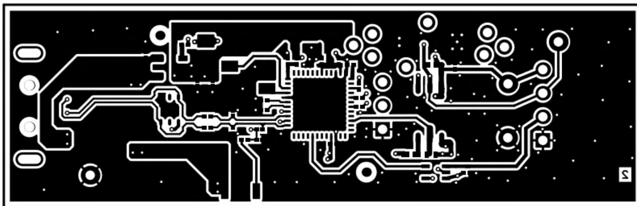
图 4-7. BQF0008EVM 覆铜 (底部)
