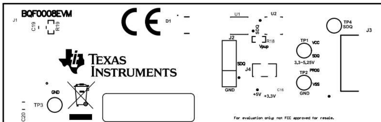
图 4-2. BQF0008EVM 丝印 (顶部)
