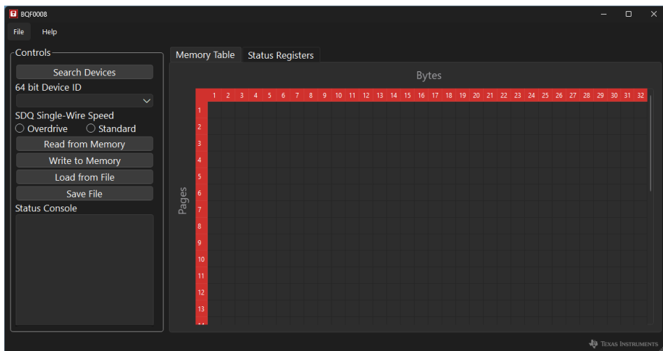
图 3-3. EVM GUI 主屏幕
