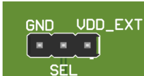
图 2-2. 接头 J7 : J7-1 (VDD_EXT)、J7-2 ( 连接到器件 SEL )、J7-3 (GND)
