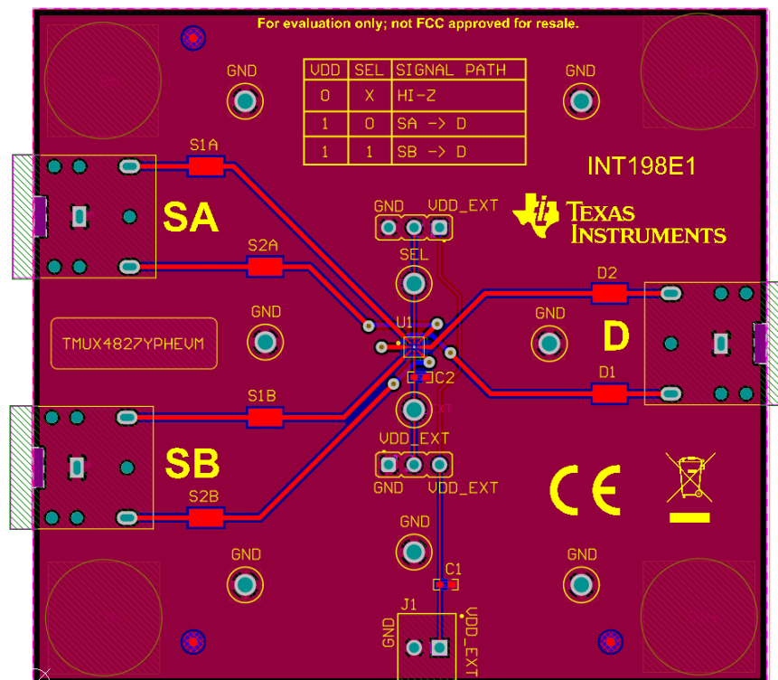
图 3-2. TMUX2889YBHEVM 顶层布局
