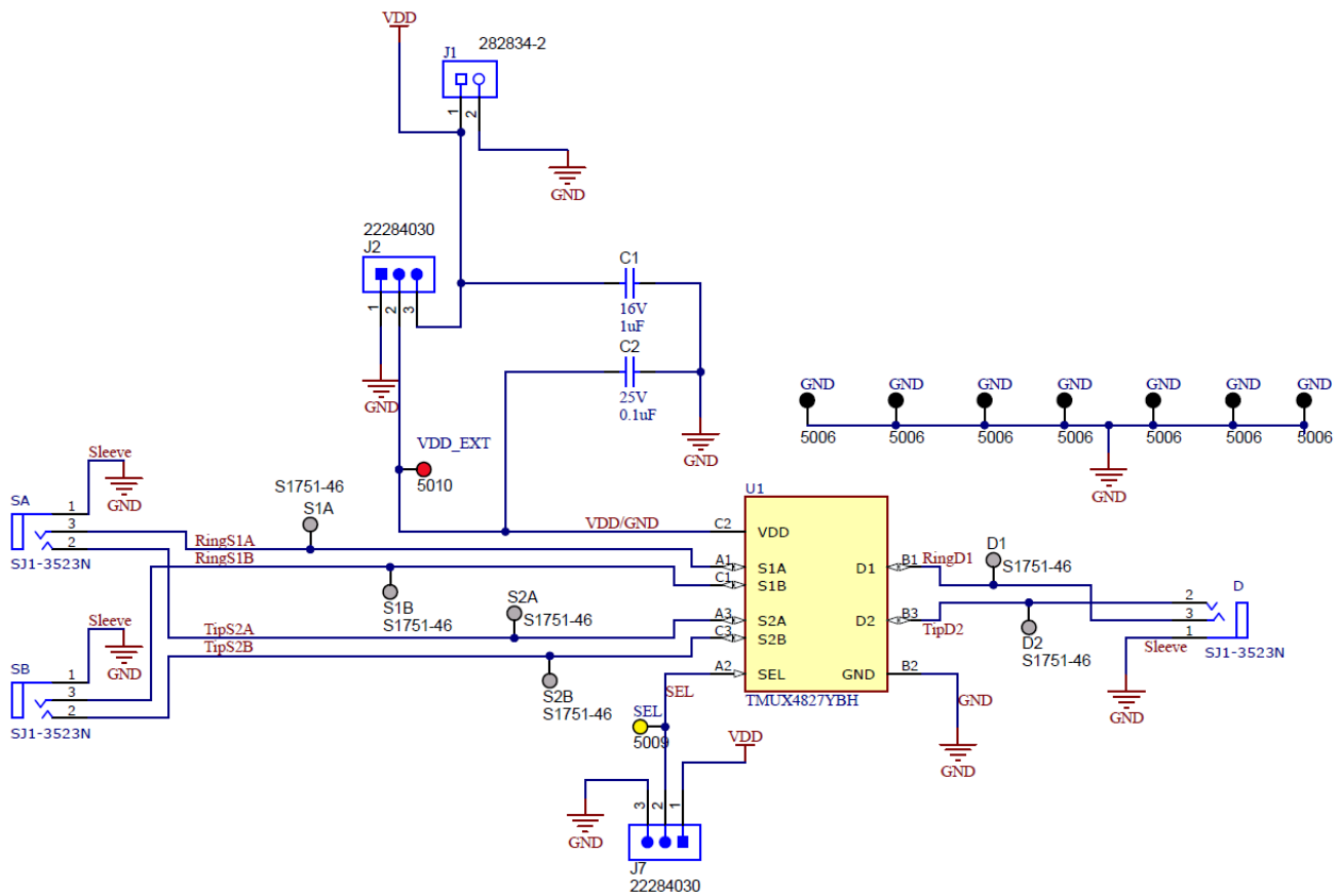
图 3-1. TMUX2889YBHEVM 原理图
