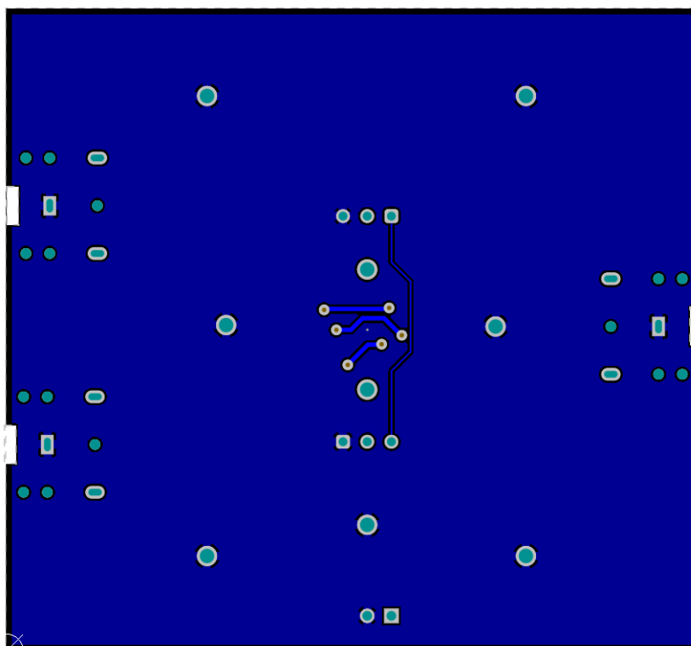
图 3-3. TMUX2889YBHEVM 底层布局
