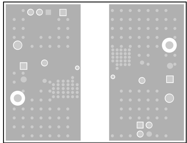
图 4-5. 接地层 2
