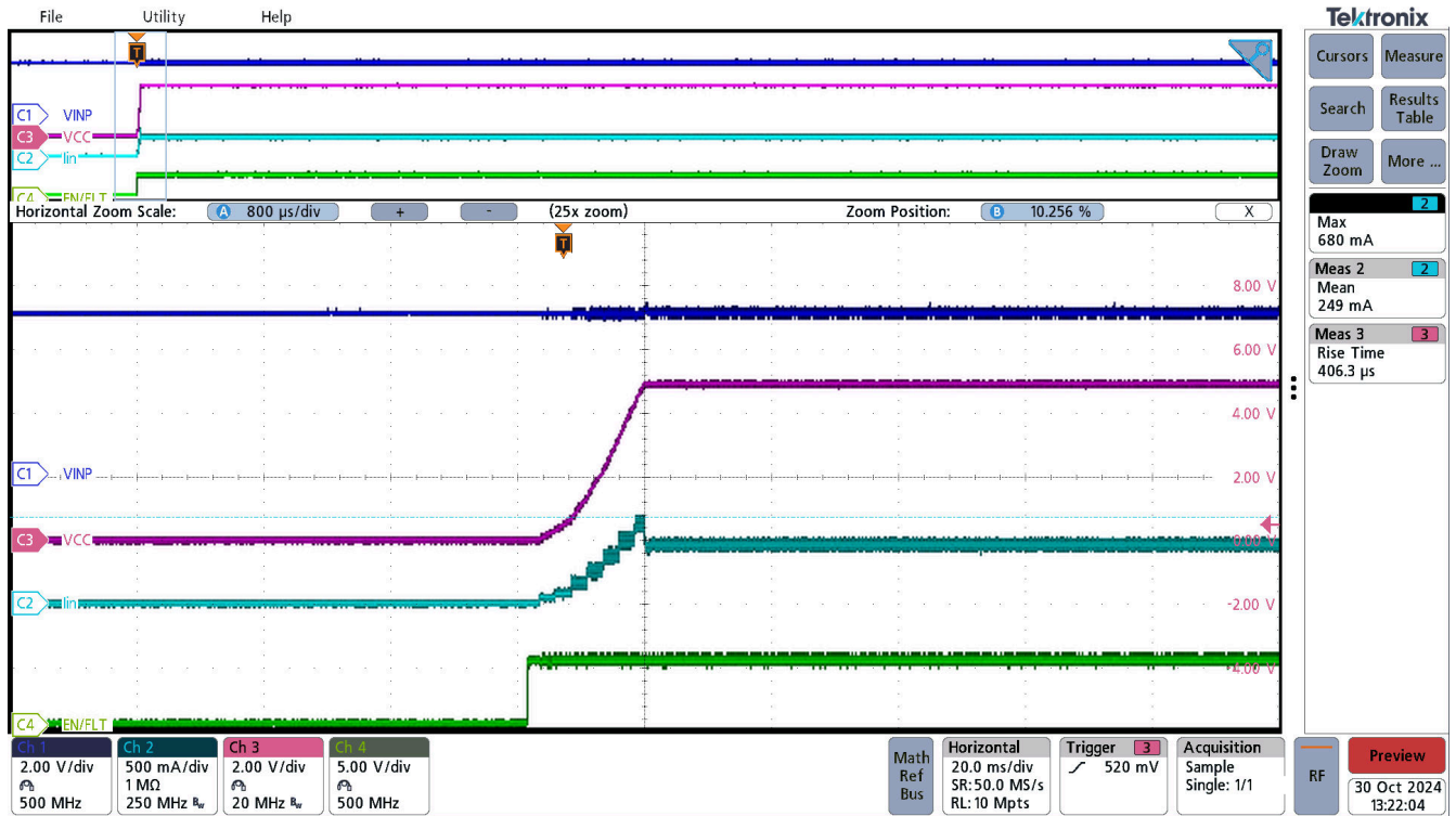
图 3-11. UCC33421-Q1 浪涌电流，序列 VINP=5.0V → EN =5.0V，VCC=5.0V，Rload=18 \Omega
