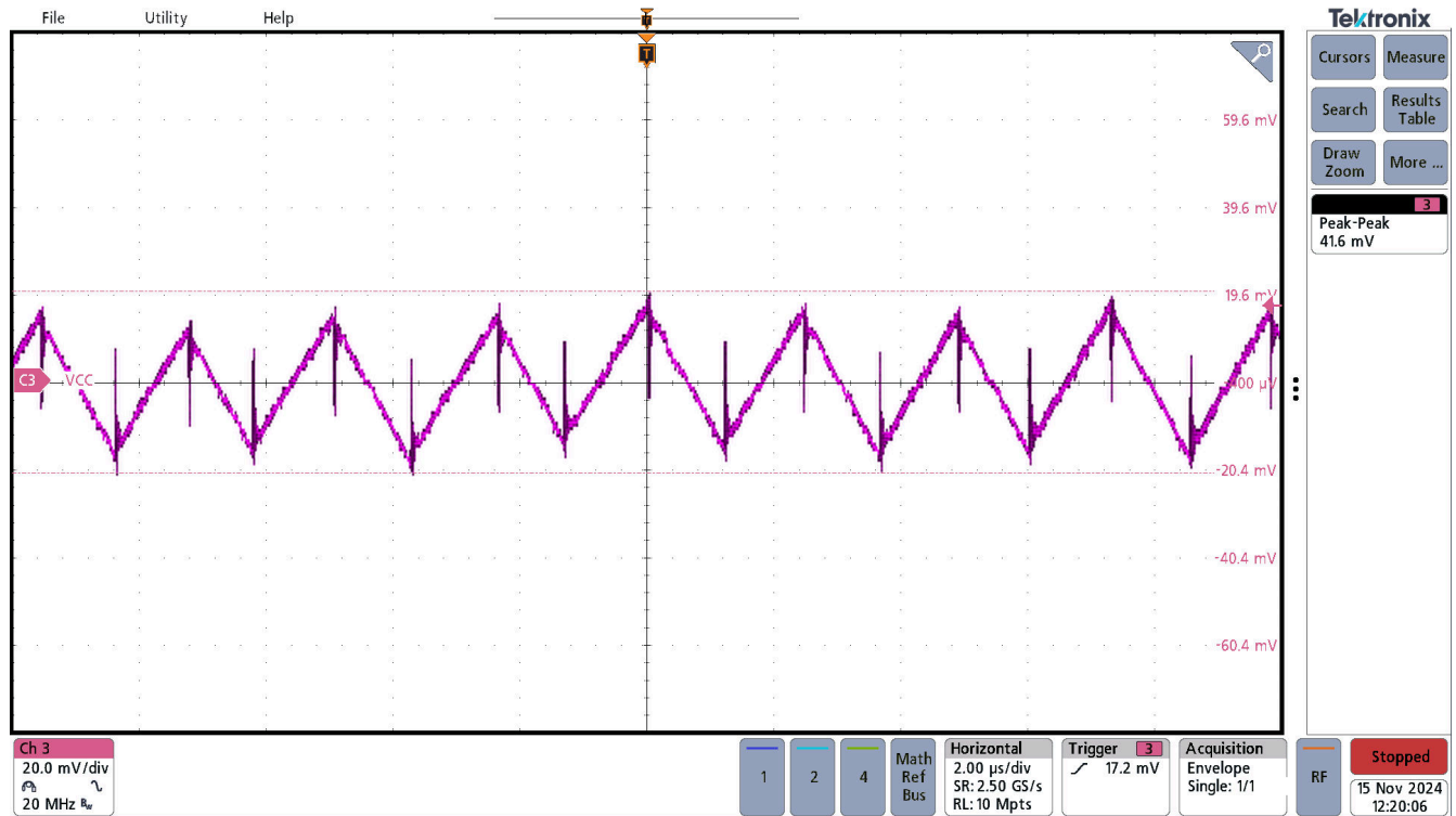
图 3-16. UCC33411-Q1 VCC 交流纹波, VINP=5.0V, VCC = 5.0V, I OUT = 300mA
