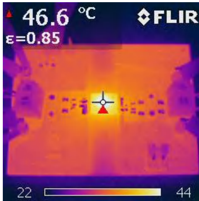
图 3-26. UCC33411-Q1 VINP=5.0V , VCC=3.3V , I OUT =150mA , P out =0.5W , TA=25°C
