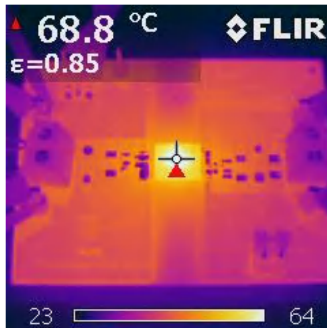
图 3-24. UCC33411-Q1 VINP=5.0V , VCC=3.3V , I OUT =300mA , P out =1W , TA=25°C
