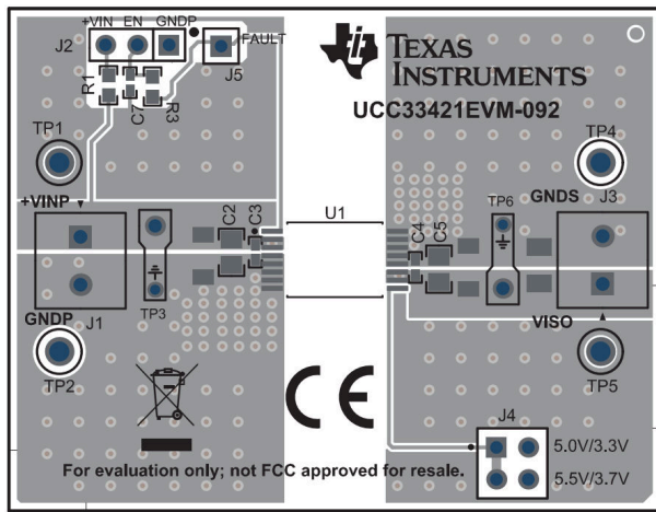
图 4-4. PCB 顶层，组装
