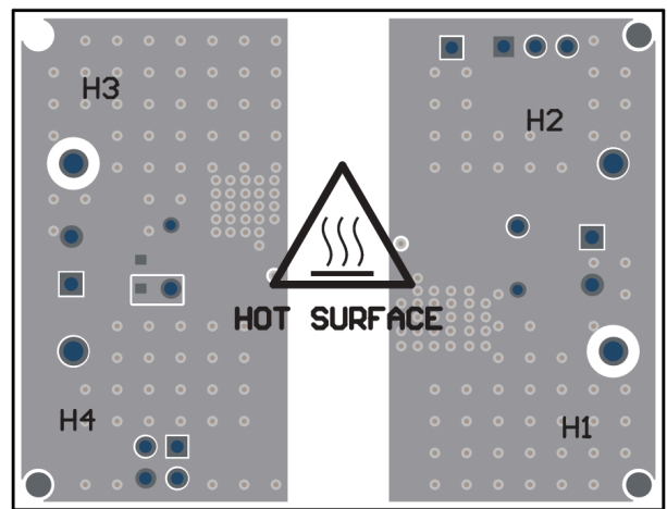
图 4-7. PCB 底层，组装 ( 镜像视图 )
