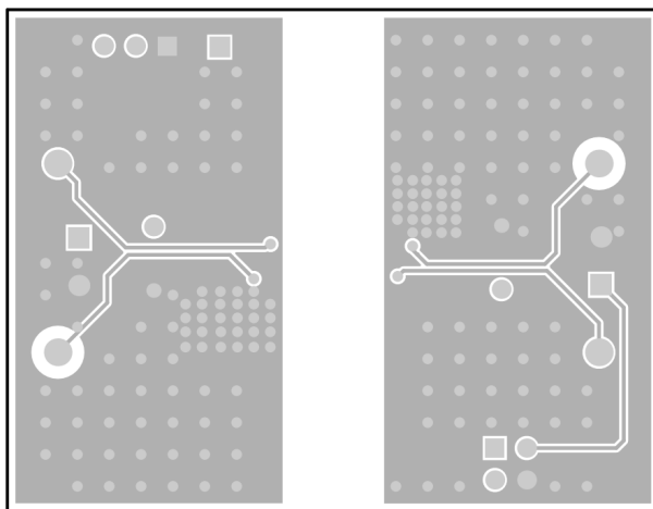
图 4-6. 接地层 3
