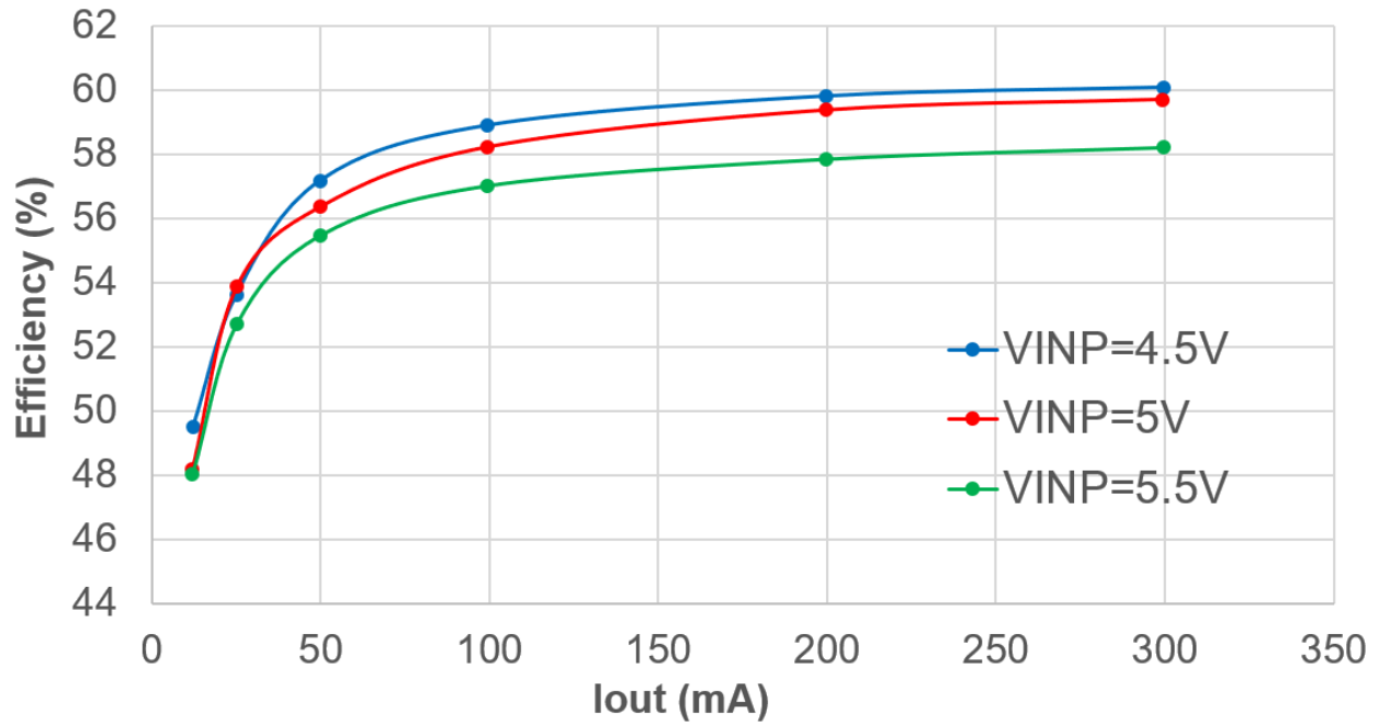
图 3-1. UCC33421-Q1 在 VCC = 5.0V 时的效率
