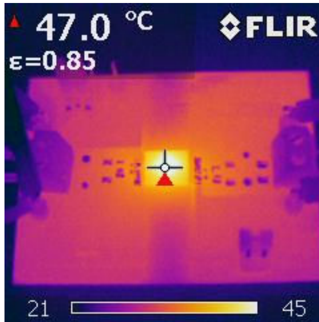
图 3-25. UCC33421-Q1 VINP=5.0V , VCC=5.0V , I OUT =150mA , P out =0.75W , TA=25°C
