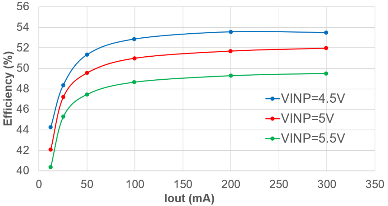
图 3-2. UCC33411-Q1 在 VCC = 3.3V 时的效率
