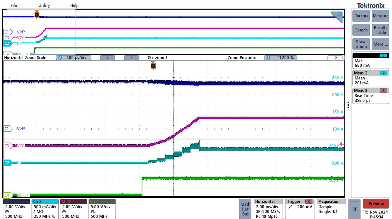
图 3-12. UCC33411-Q1 浪涌电流，序列 VINP=5.0V → EN =5.0V，VCC=3.3V，Rload=10 \Omega
