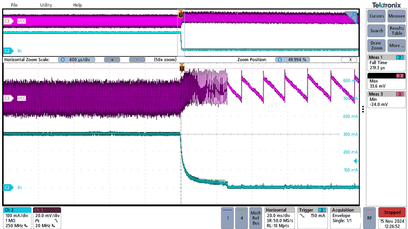
图 3-20. UCC33411-Q1 负载瞬态，VINP=5.0V，VCC=3.3V，满载 ( I_{out}=300\text{mA} ) 到空载 ( I_{out}=0\text{mA} )
