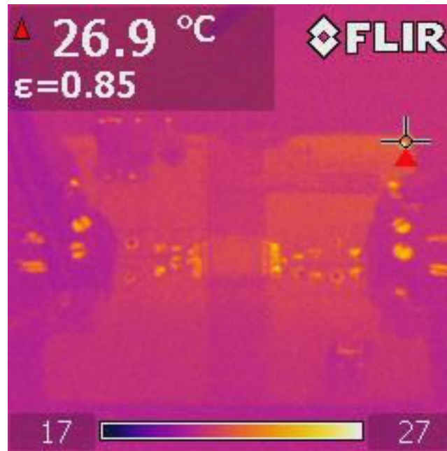
图 3-27. UCC33421-Q1 VINP=5.0V , VCC=5.0V , I OUT =0mA , P out =0W , TA=25°C
