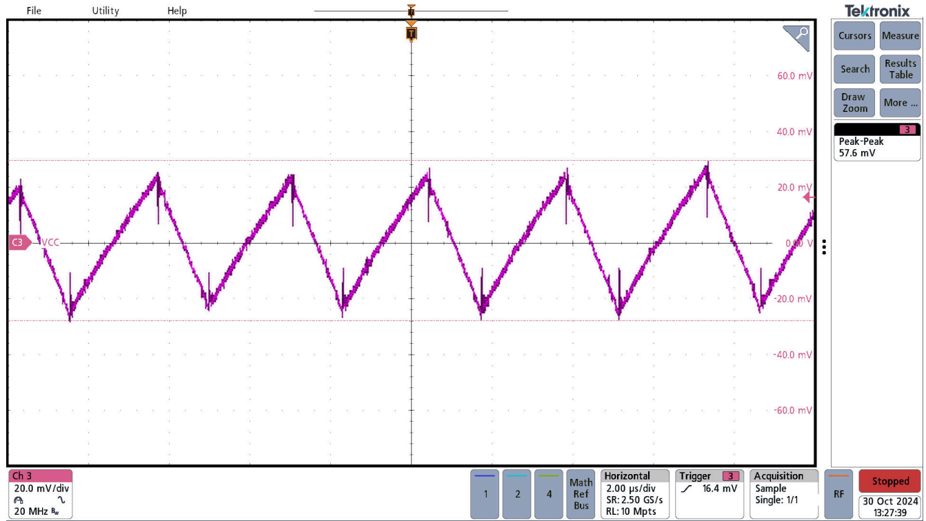
图 3-15. UCC33421-Q1 VCC 交流纹波, VINP=5.0V, VCC = 5.0V, I OUT = 300mA
