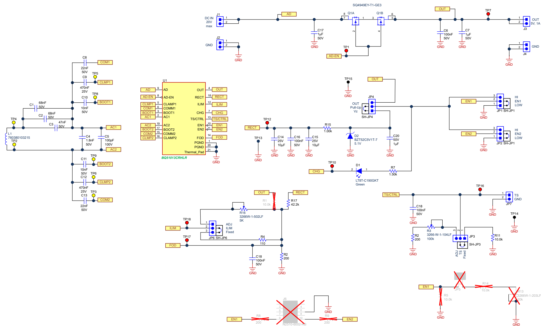
图 3-1. BQ51013C 原理图
