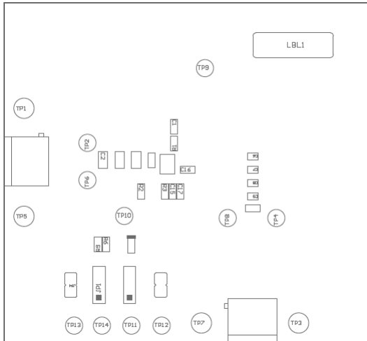
图 4-7. 顶层元件图
