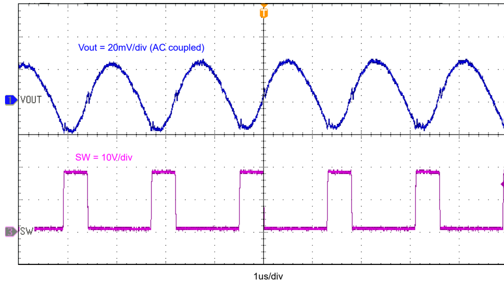
图 3-9. TPS513885EVM 输出电压纹波, I_{OUT} = 12A
