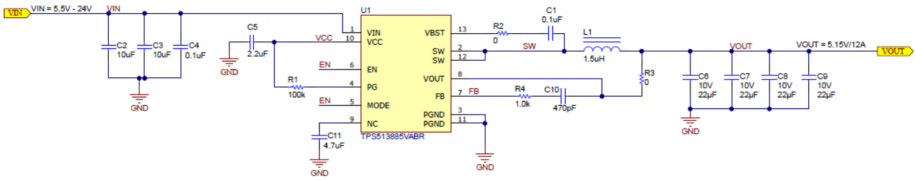
图 1-1. TPS513885 同步降压稳压器简化原理图
