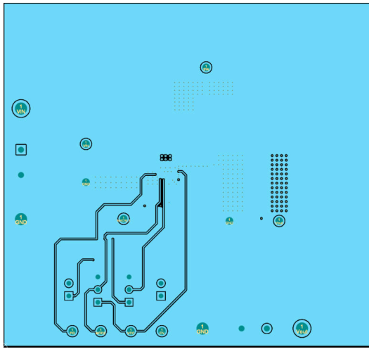
图 4-4. 第 3 层铜 ( 顶视图 )
