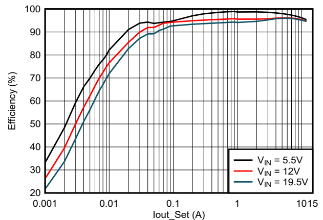
图 3-2. 效率, V_{EN} = 1.2V (OOA 模式), V_{OUT} = 5.15V , 560kHz
