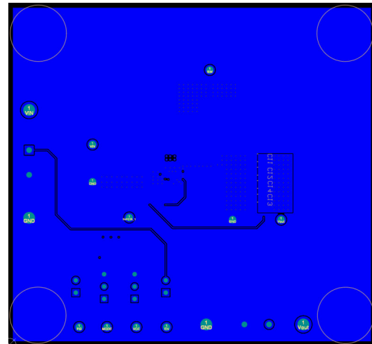
图 4-5. 底层铜 ( 顶视图 )
