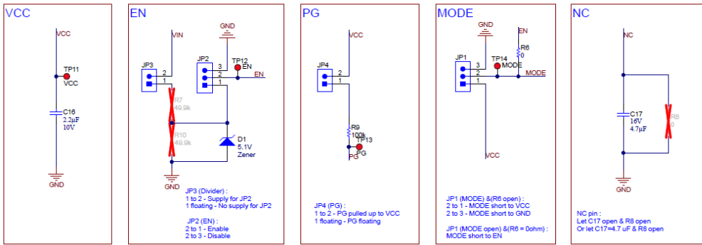
图 4-1. TPS513885EVM 原理图
