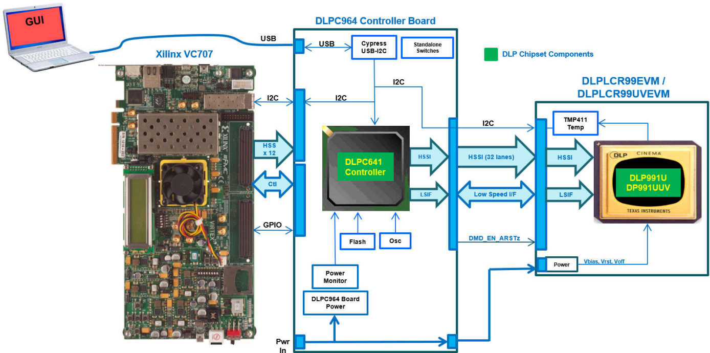
图 1-2. DLPLCR964EVM 硬件元件
