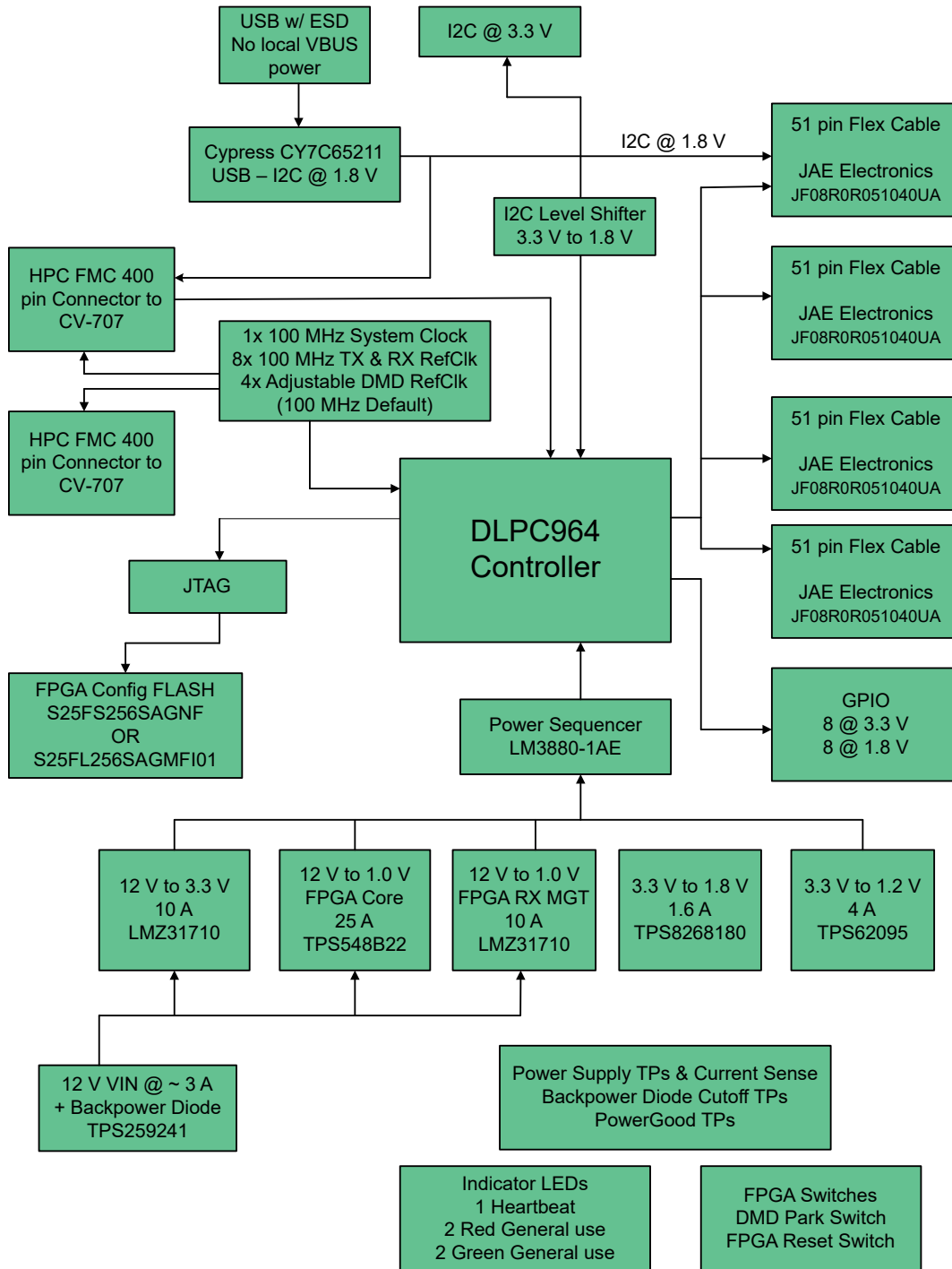
图 1-1. DLP LightCrafter DLPC964 EVM 方框图
