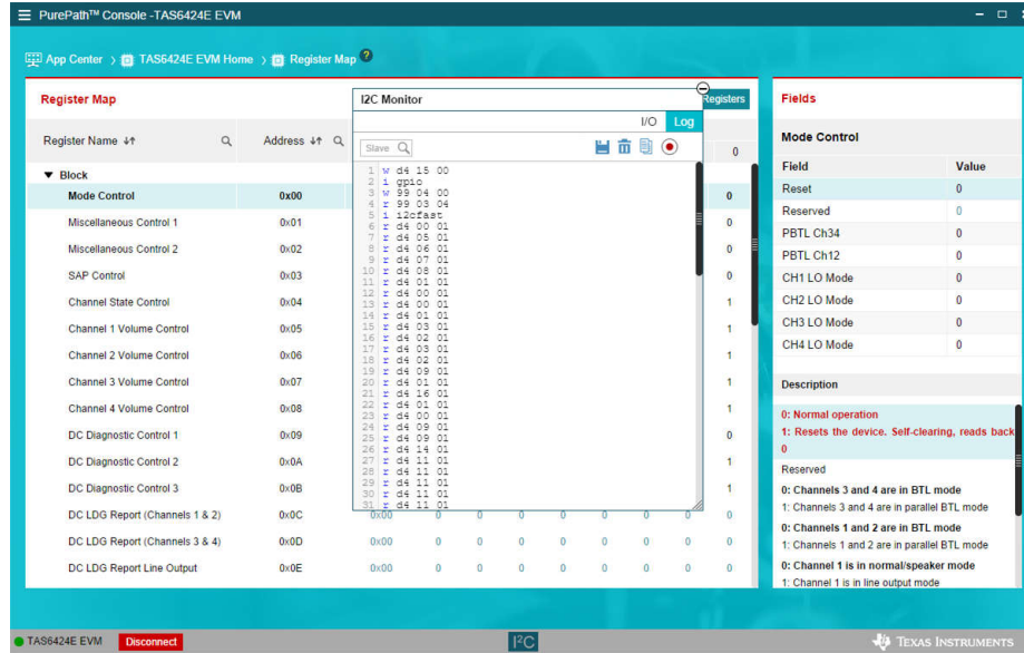
图 2-18. I2C 窗口 - I2C 日志记录
