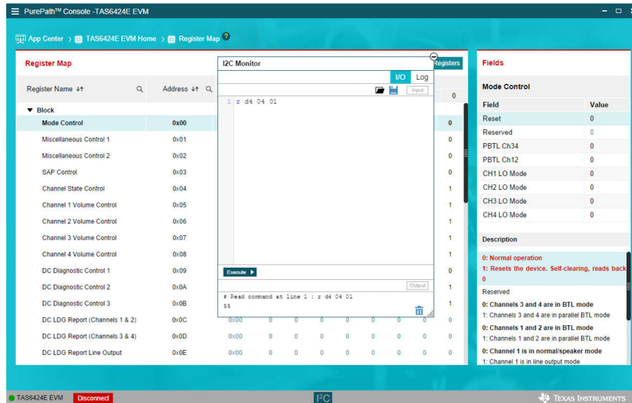
图 2-19. I2C 窗口 - 发送 I2C 命令
