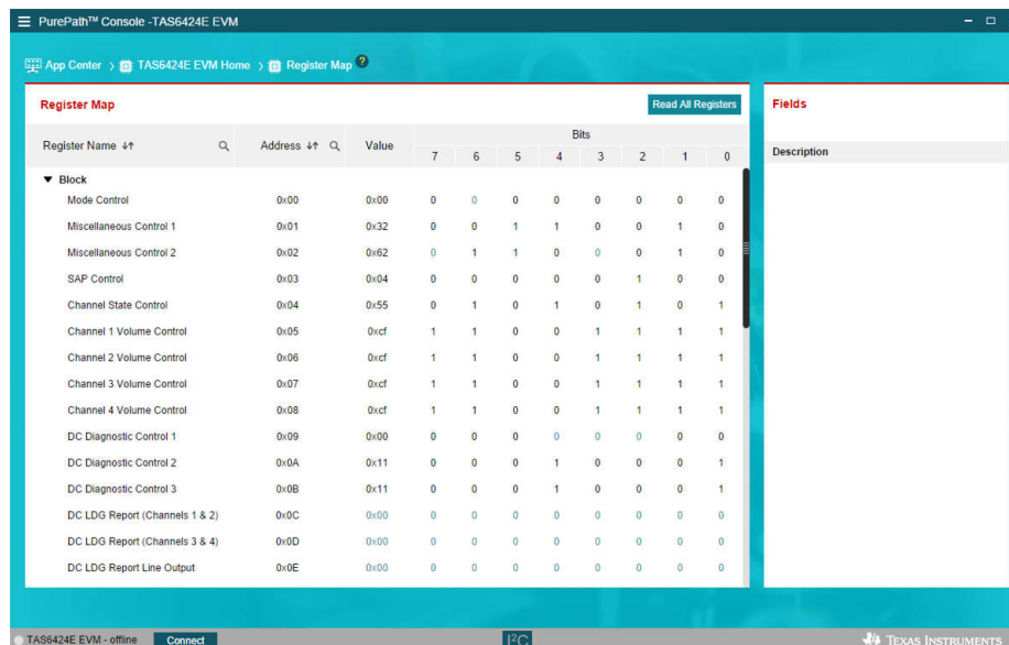
图 2-6. TAS6424E EVM 寄存器映射窗口
