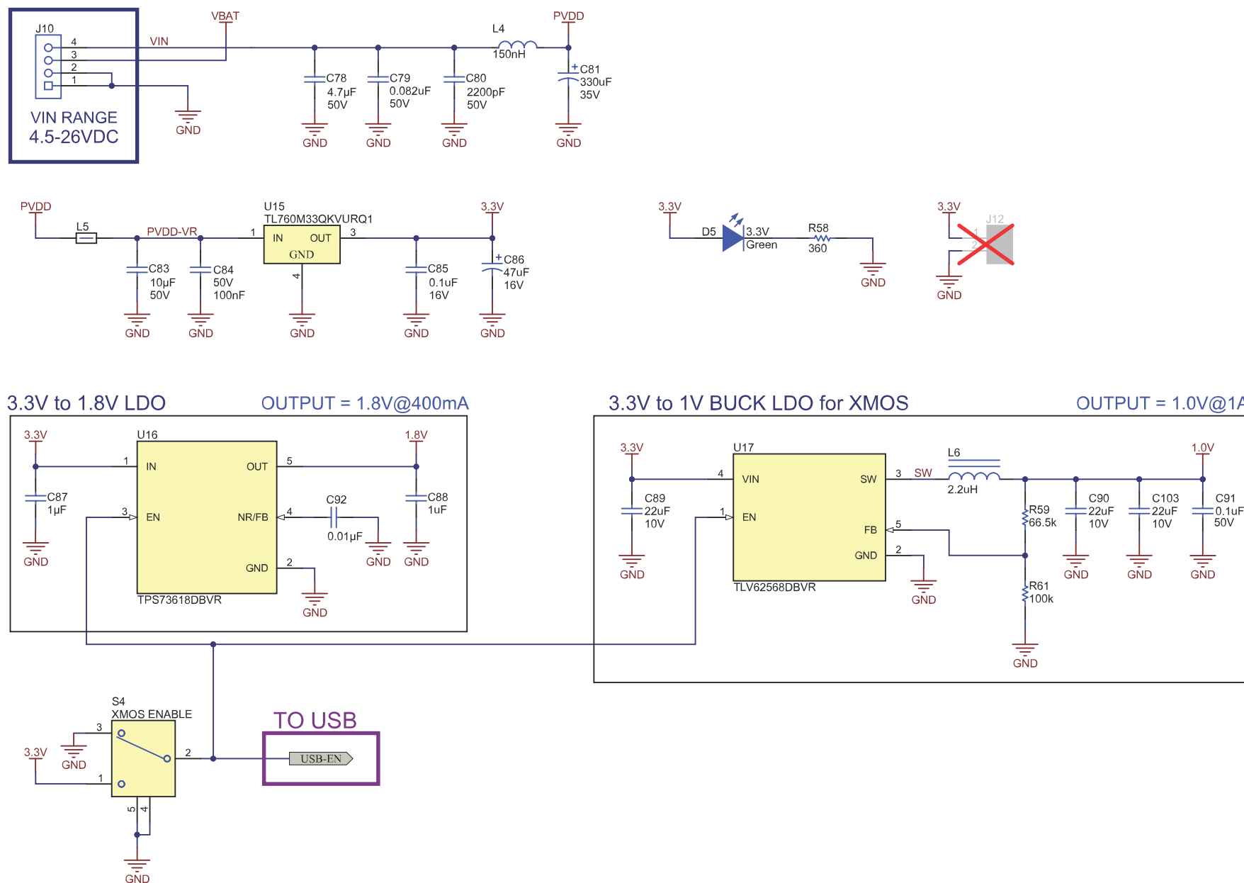
图 3-4. 原理图 ( 页面 4 )
