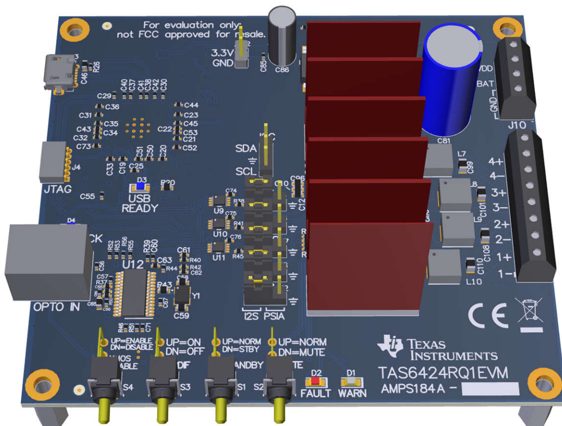
图 1-1. TAS6424R-Q1 EVM
