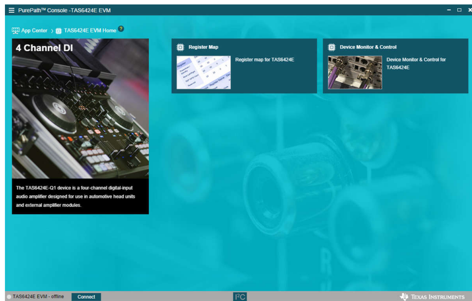
图 2-5. TAS6424E EVM 主窗口
