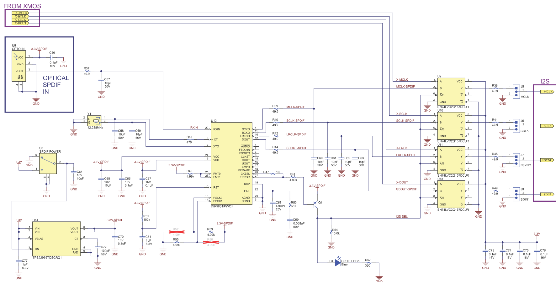
图 3-2. 原理图 ( 页面 2 )
