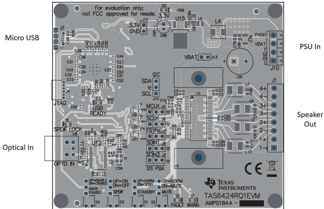
图 2-8. TAS6424R-Q1 EVM 连接
