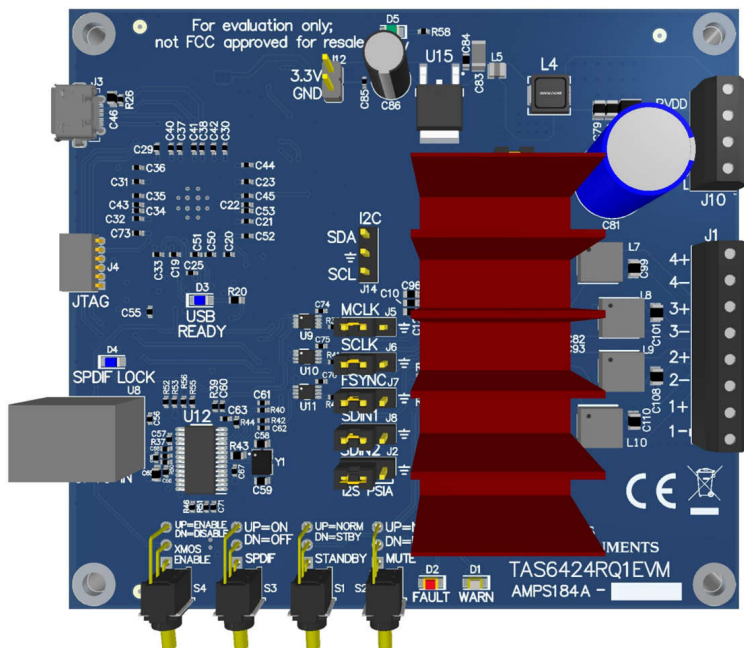
图 3-5. TAS6424R-Q1 EVM 顶视图
