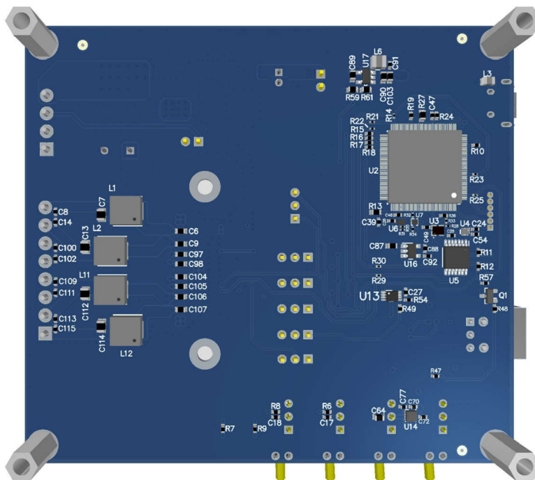
图 3-6. TAS6424R-Q1 EVM 底视图
