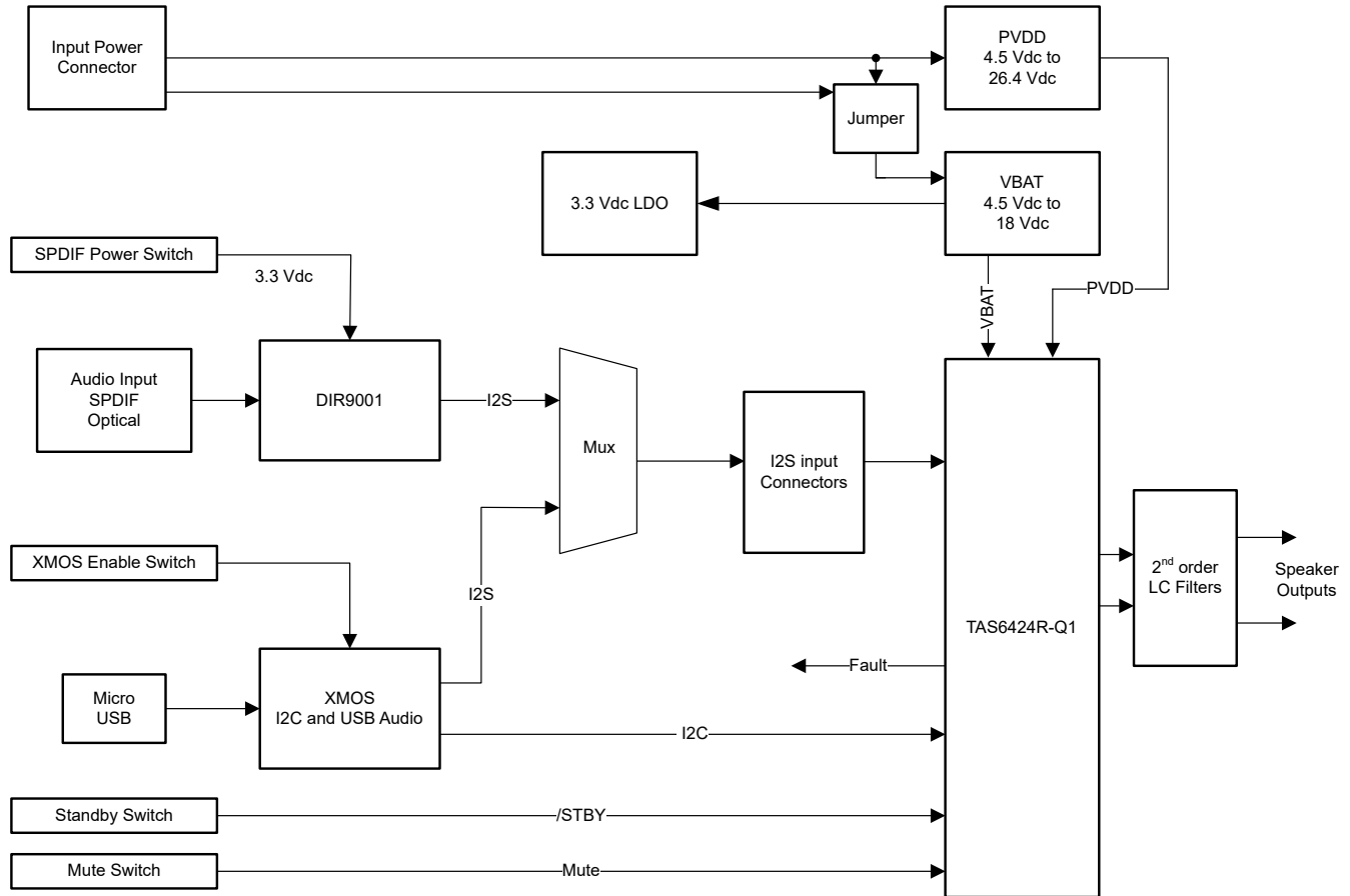
图 1-2. EVM 方框图
