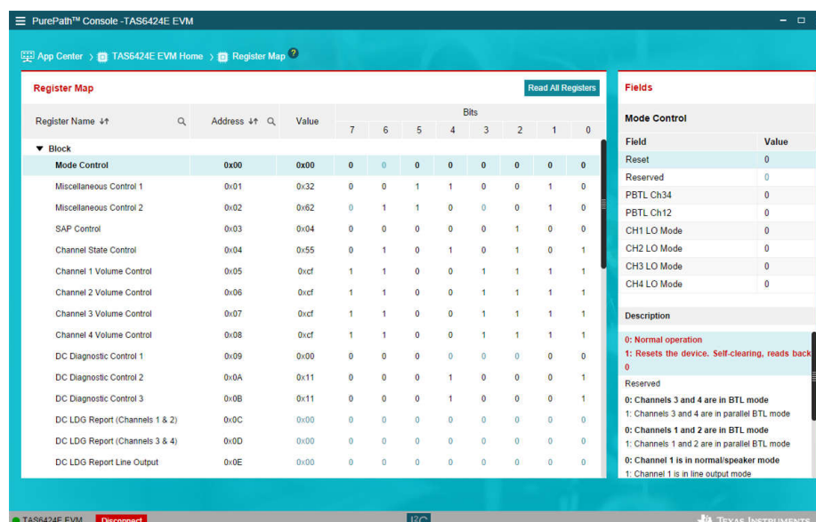
图 2-17. 寄存器映射窗口 - 展开
