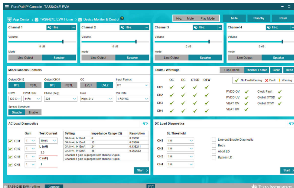
图 2-7. TAS6424E EVM 器件监测和控制窗口
