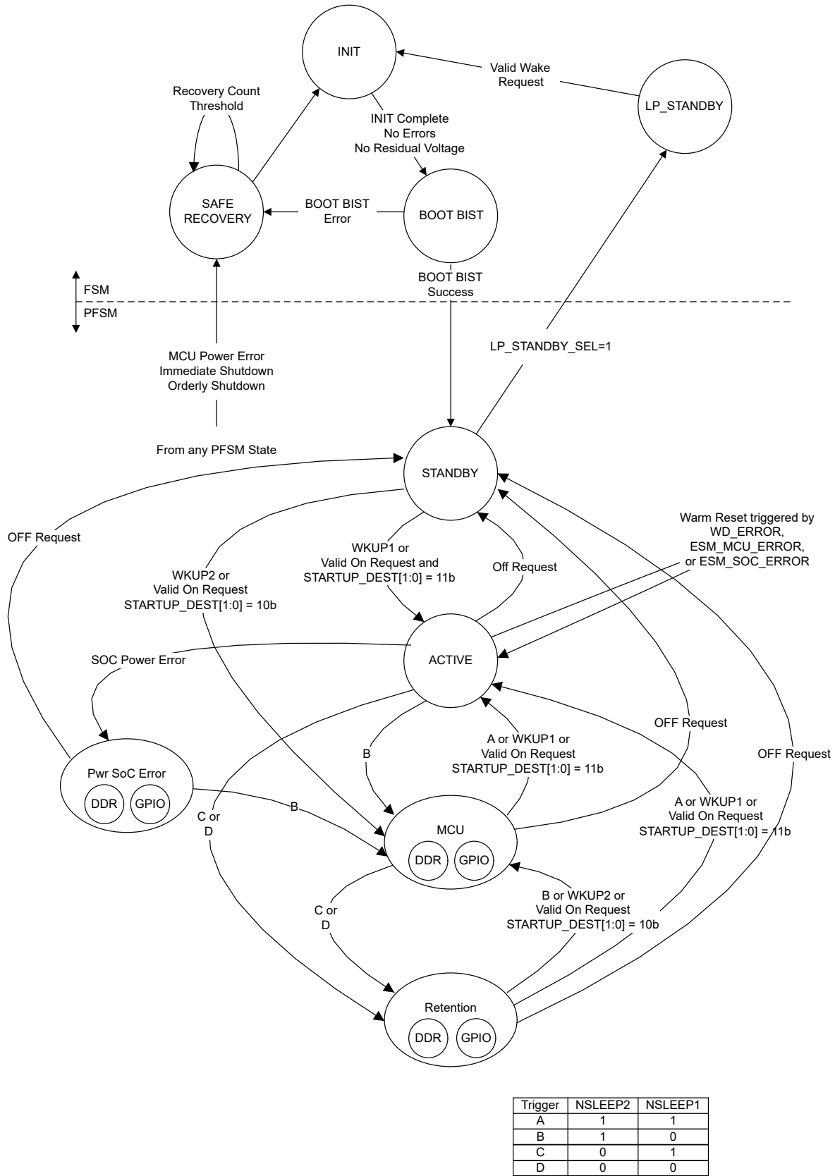
图 6-1. 可预配置有限状态机 (PFMS) 的任务状态和转换
