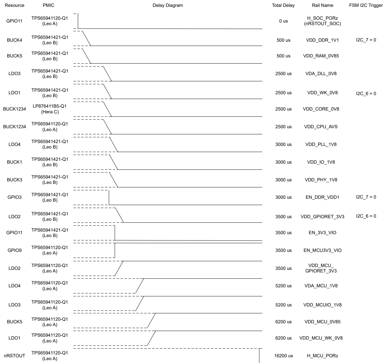
图 6-10. 两个 PMIC 上的 I2C 触发条件均为低电平时的 TO_MCU 序列
