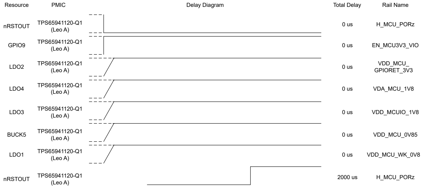
图 6-8. MCU_TO_WARM 序列
