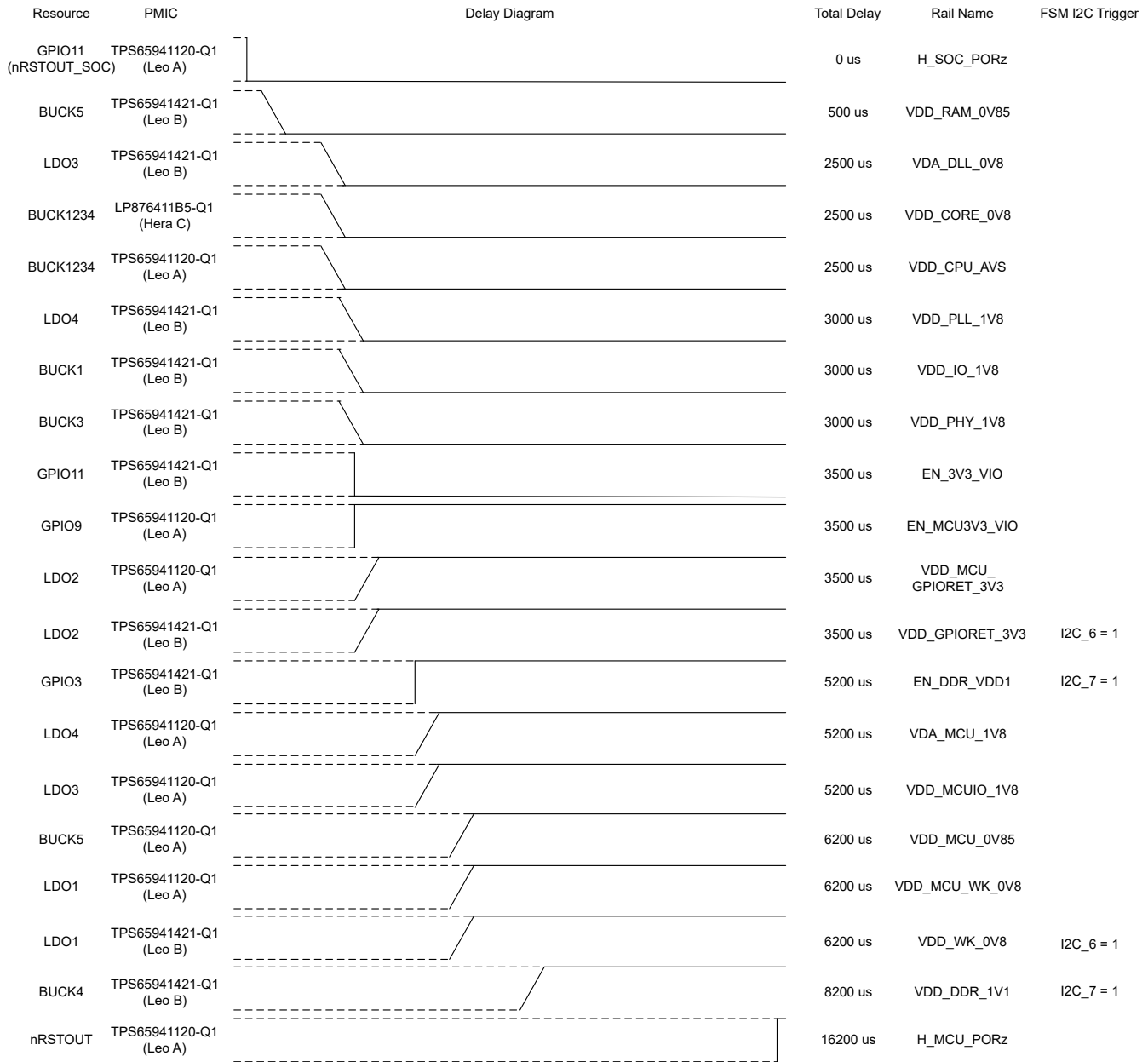
图 6-9. 两个 PMIC 上的 I2C 触发条件均为高电平时的 TO_MCU
