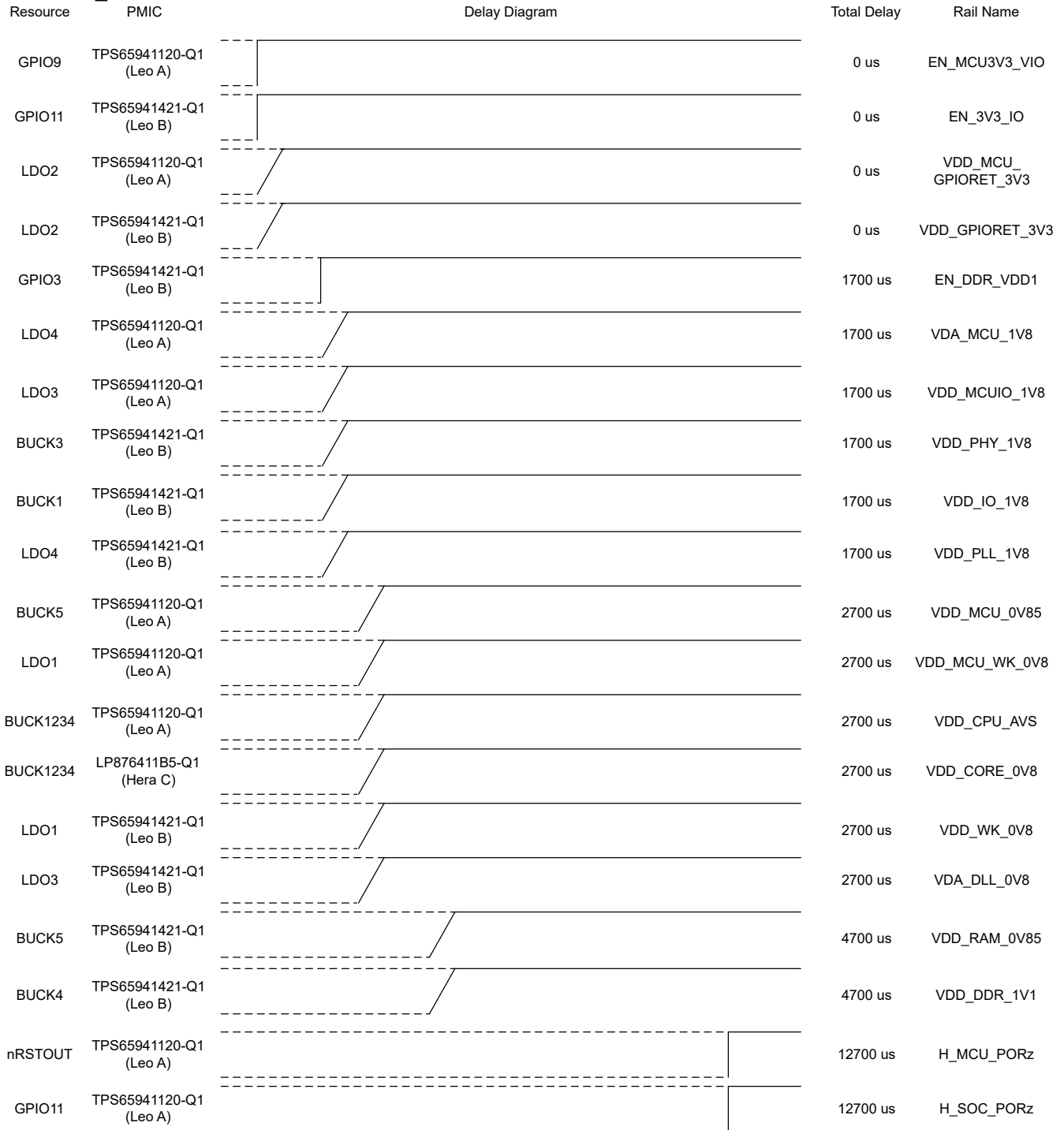
图 6-11. TO_ACTIVE 序列
