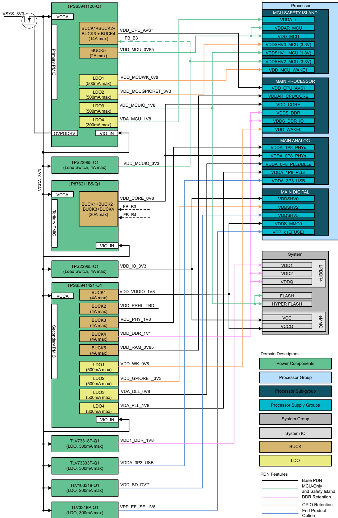
图 3-1. 电源连接
