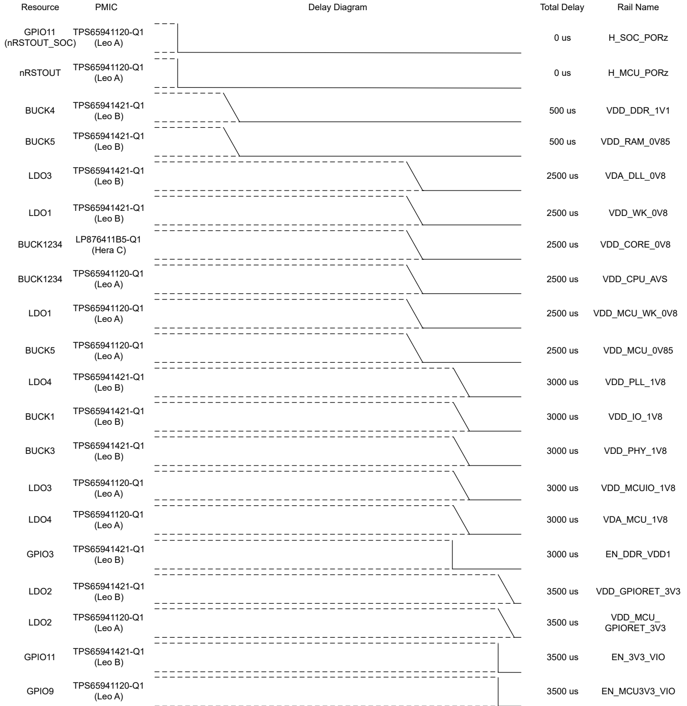
图 6-3. TO_SAFE_ORDERLY 和 TO_STANDBY 电源序列
