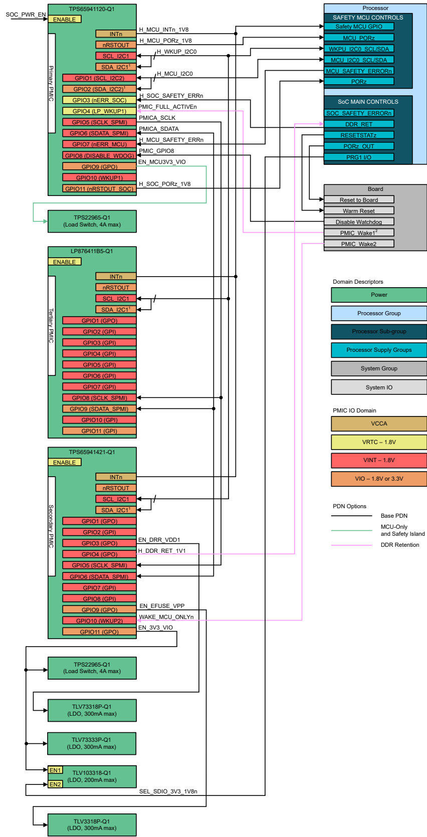
图 3-2. PDN-0A 数字连接
