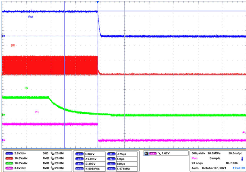
图 5-9. 启用关断，强制 PWM ( V_{IN} = 12V , V_{OUT} = 3.3V , I_{OUT} = 1A )
