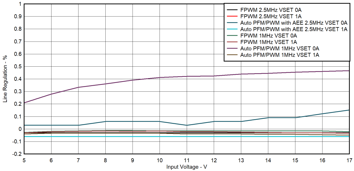
图 5-3. 线路调节 ( V_{IN} = 5V - 17V , V_{OUT} = 3.3V , I_{OUT} = 0A 和 1A , F_{SW} = 2.5MHz 和 1MHz )
