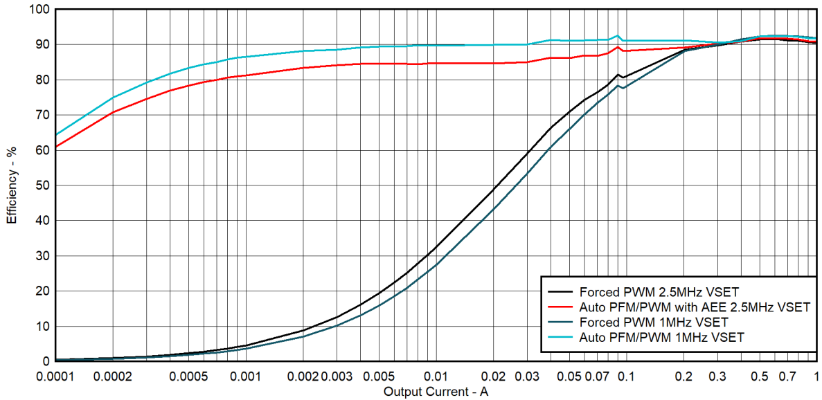
图 5-1. 效率 ( V_{IN} = 12V , V_{OUT} = 3.3V , F_{SW} = 2.5MHz 和 1MHz )
