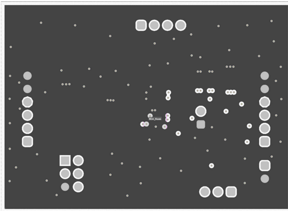
图 6-3. 内层 1
