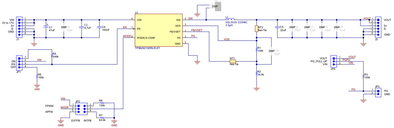
图 7-1. TPS629210EEVM 原理图
