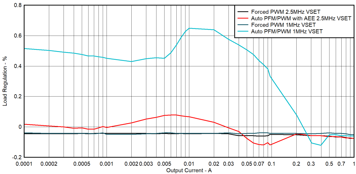
图 5-2. 负载调节 ( V_{IN} = 12V , V_{OUT} = 3.3V , F_{SW} = 2.5MHz 和 1MHz )
