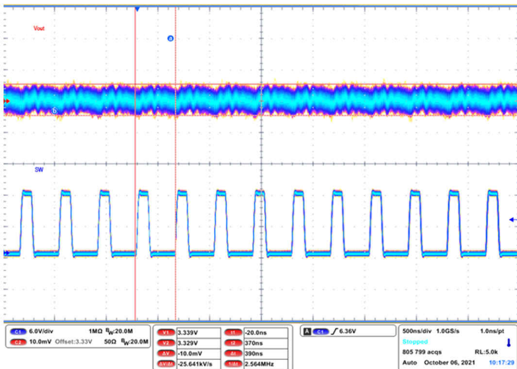
图 5-6. 输出电压纹波，强制 PWM ( V_{IN} = 12V , V_{OUT} = 3.3V , I_{OUT} = 1A )
