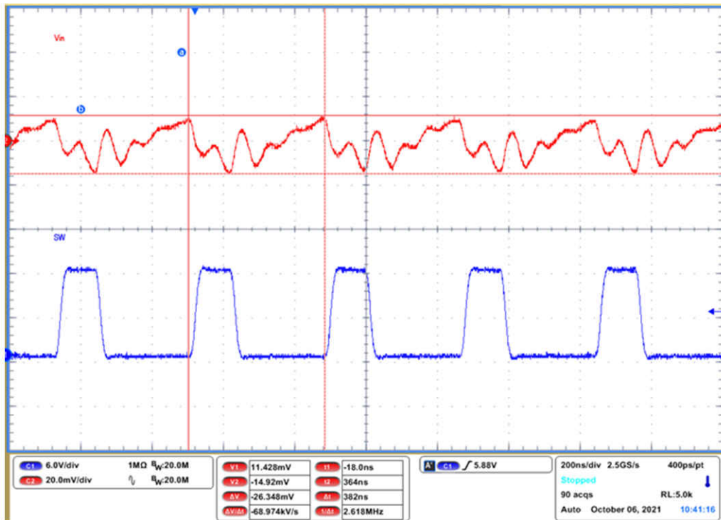
图 5-7. 输入电压纹波，强制 PWM ( V_{IN} = 12V , V_{OUT} = 3.3V , I_{OUT} = 1A )
