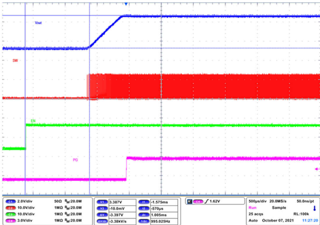
图 5-8. 启用启动，强制 PWM ( V_{IN} = 12V , V_{OUT} = 3.3V , I_{OUT} = 1A )
