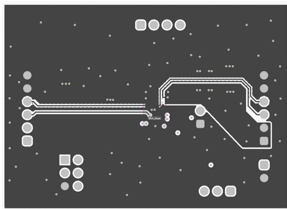
图 6-4. 内层 2
