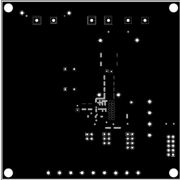
图 8-3. 第 2 层覆铜
