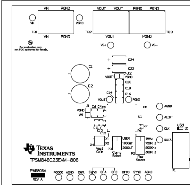
图 8-1. 顶部元件
