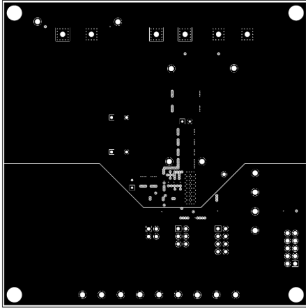
图 8-5. 第 4 层覆铜
