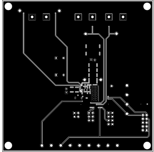
图 8-6. 第 5 层覆铜
