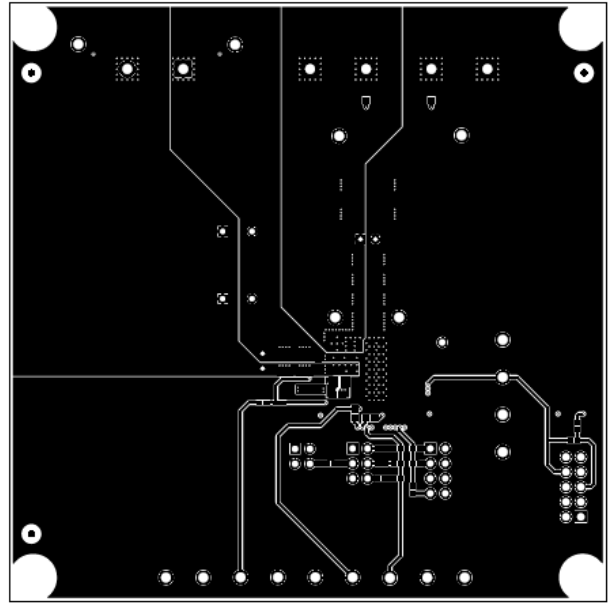
图 8-2. 顶部覆铜
