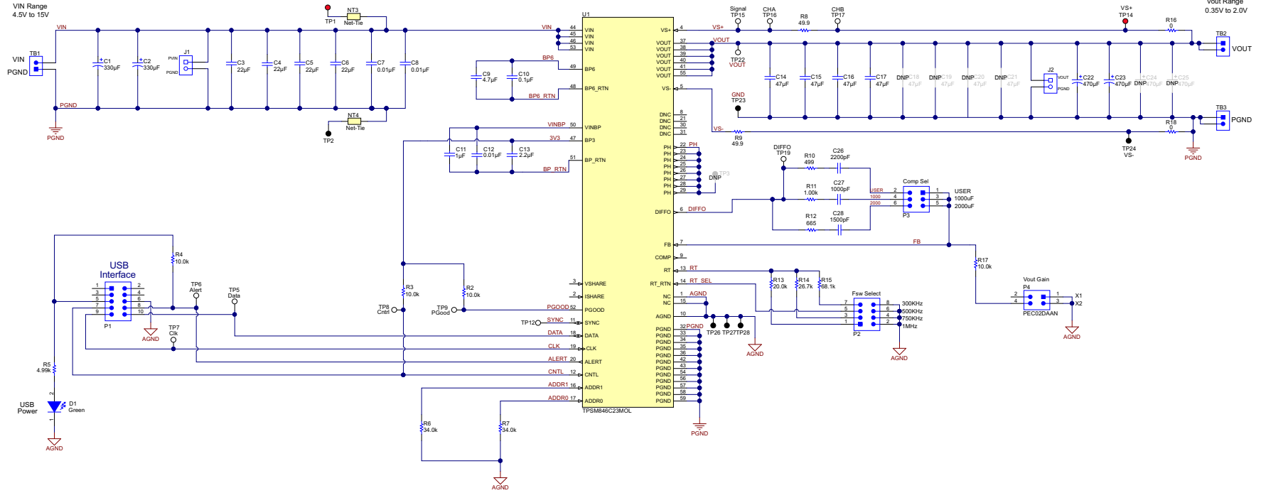
图 6-1. TPSM846C23EVM 原理图
