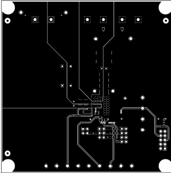
图 8-7. 底部覆铜
