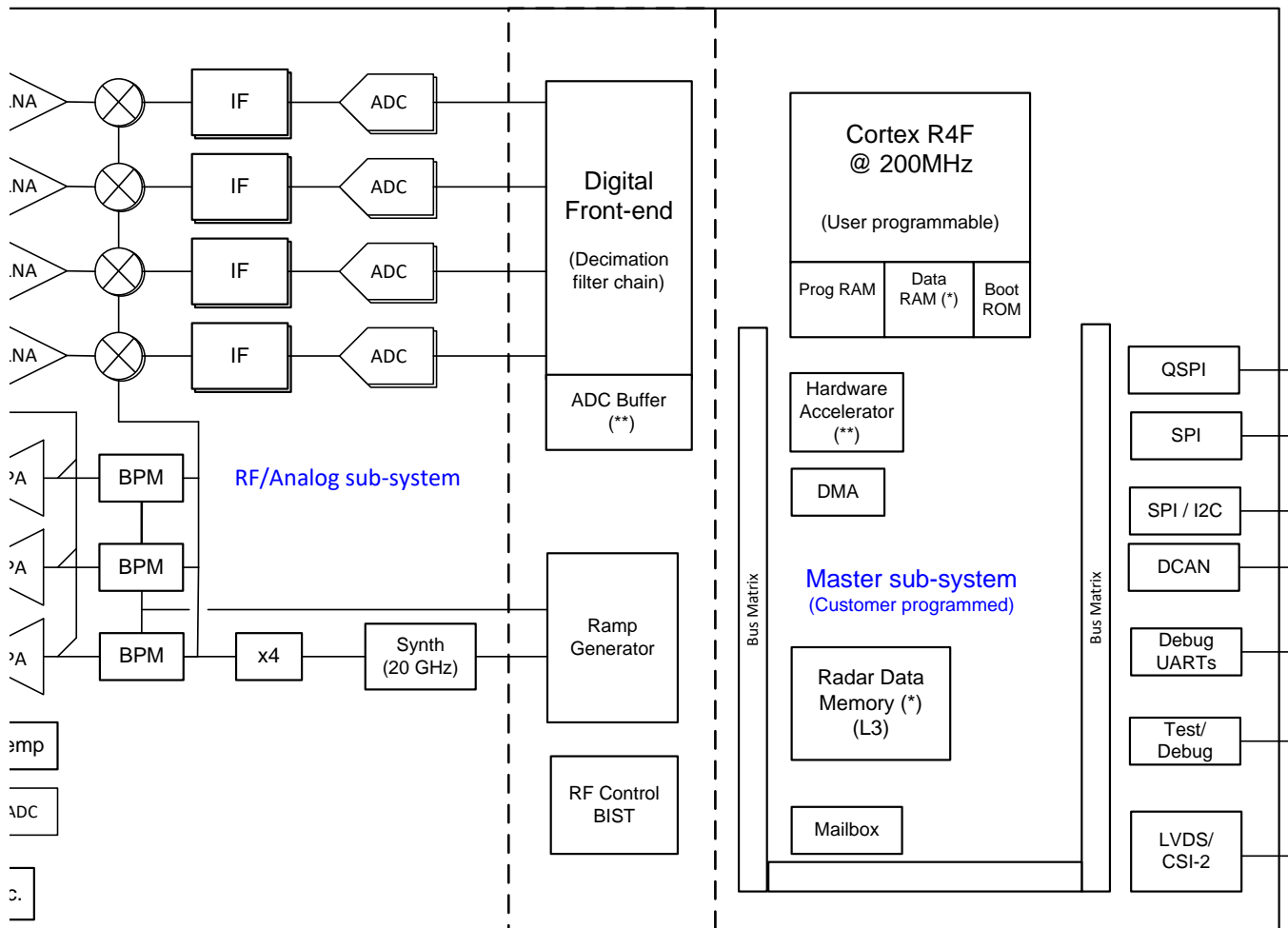
图 5. TIDEP-0091 IWR 1443 mmWave Sensor Block Diagram
