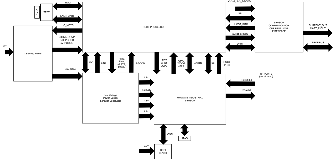
图 2. TIDEP-0091 Block Diagram
