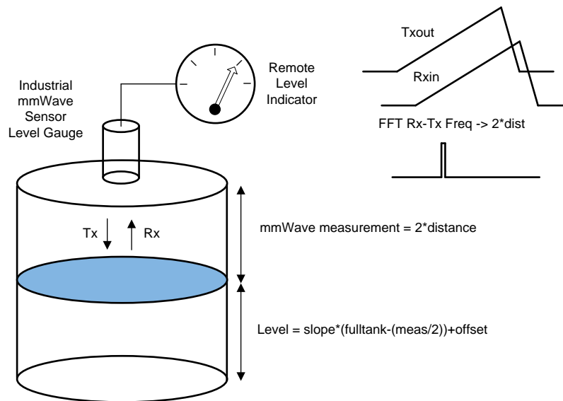
图 1. TIDEP-0091 System Block Diagram
