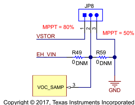
图 21. Default Solar MPPT: JP8 Connect 1-2; Default Thermal MPPT: JP8: Connect 2-3
