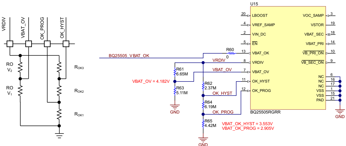
图 20. bq25505 Settings
