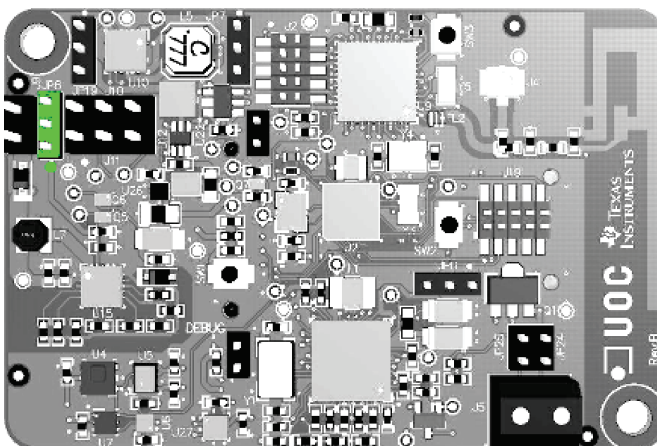
图 21. Default Solar MPPT: JP8 Connect 1-2; Default Thermal MPPT: JP8: Connect 2-3
