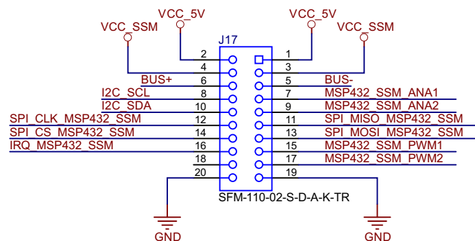
图 5. SSI on I3Mote
