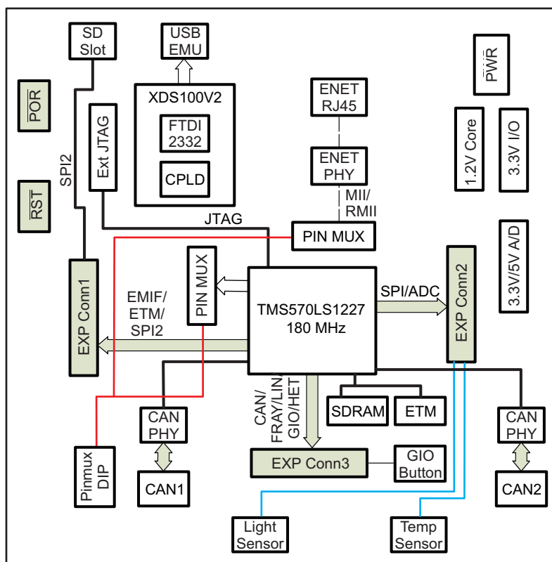
图 1-1. TMS570LS12HDK 方框图
