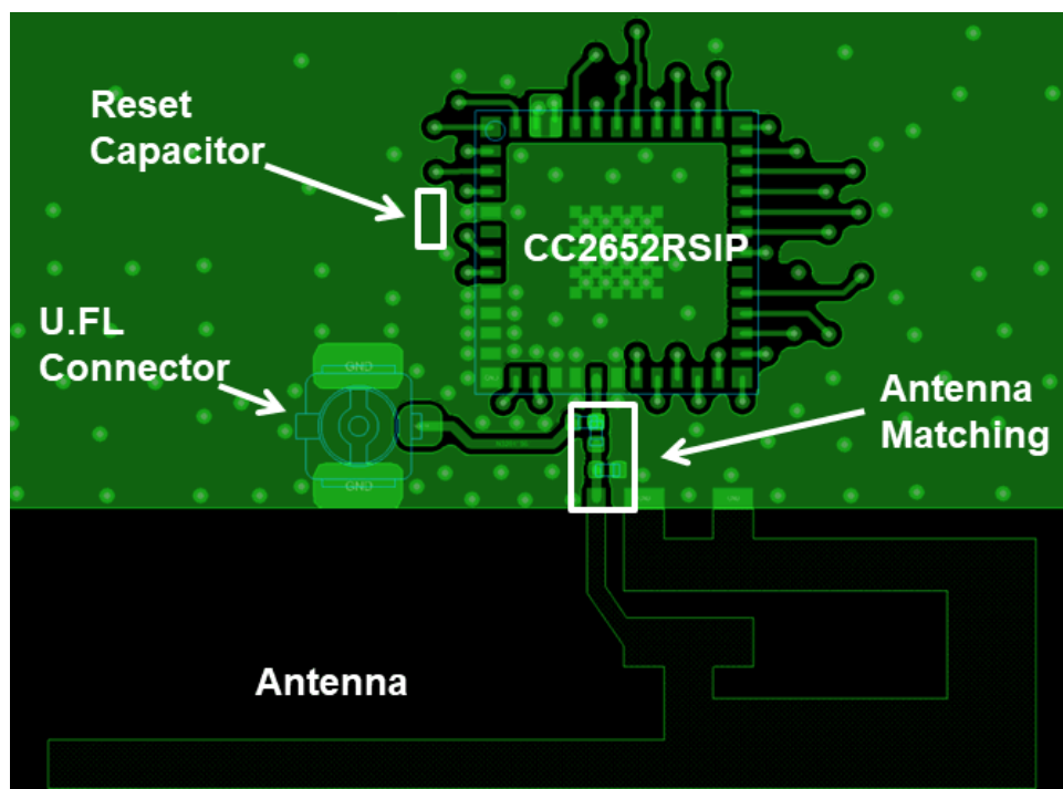
图 10-2. Module Layout Guidelines
