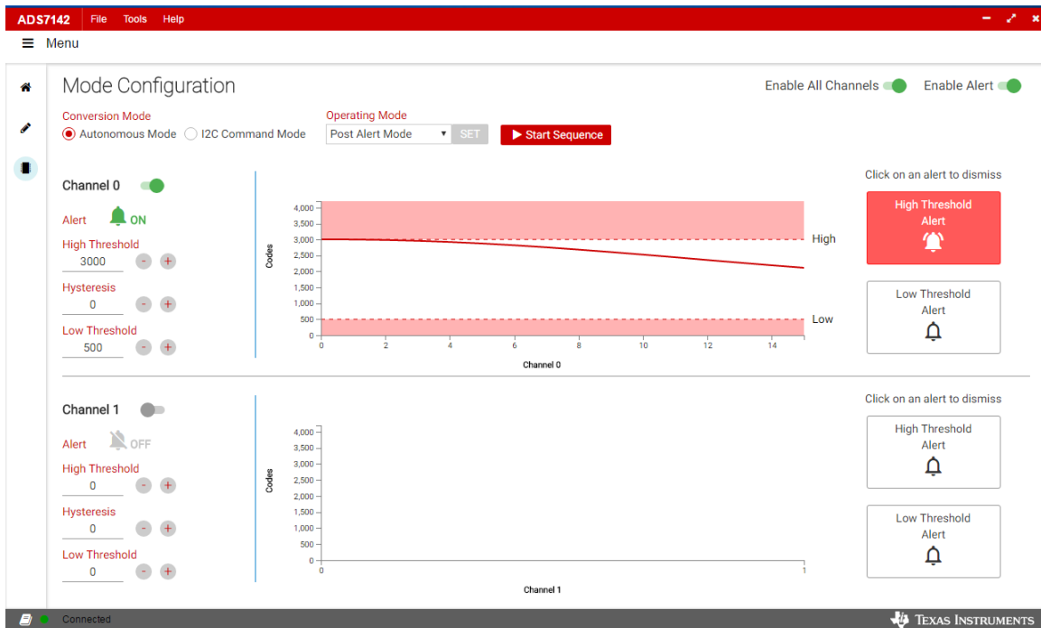
图 8-7. Post-Alert Data Capture
