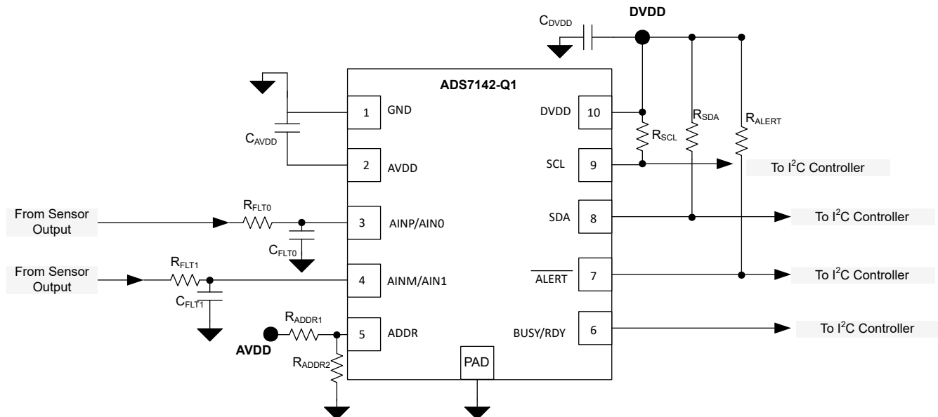
图 8-10. Example Schematic
