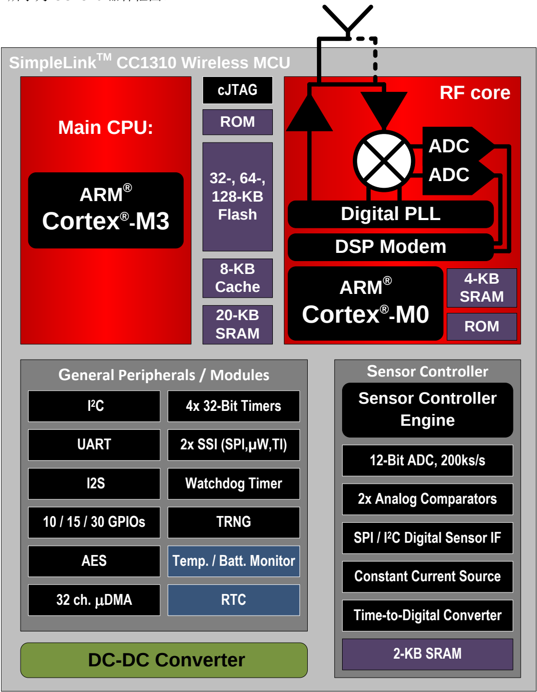
图 1-1. CC1310 框图
