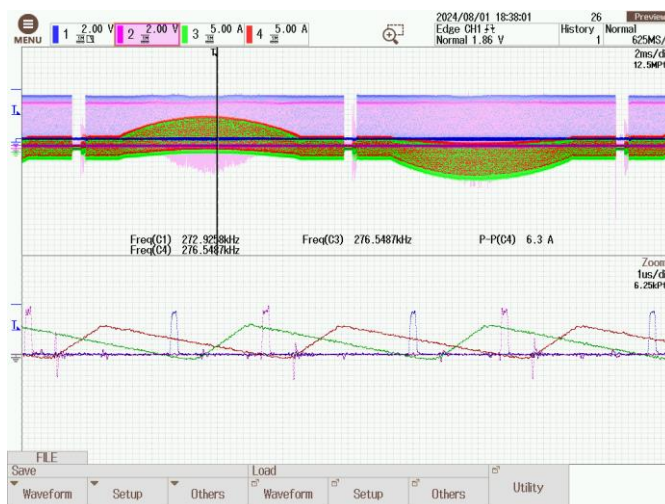
Figure 11. 消除 A 相和 B 相间的重叠后，正常波形
