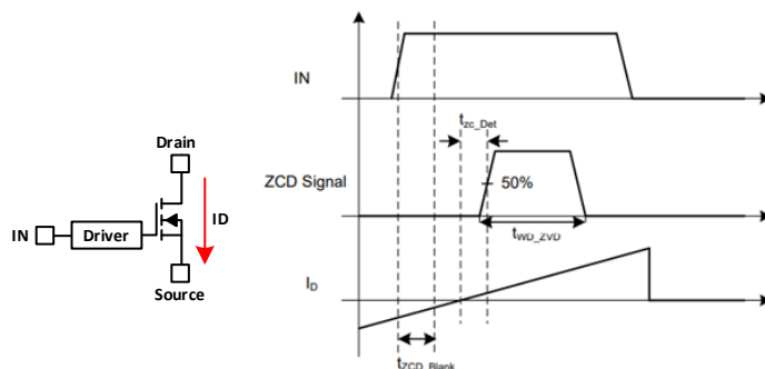
Figure 2. ZCD 脉冲时序，IN 引脚置高时刻且电流为负时
