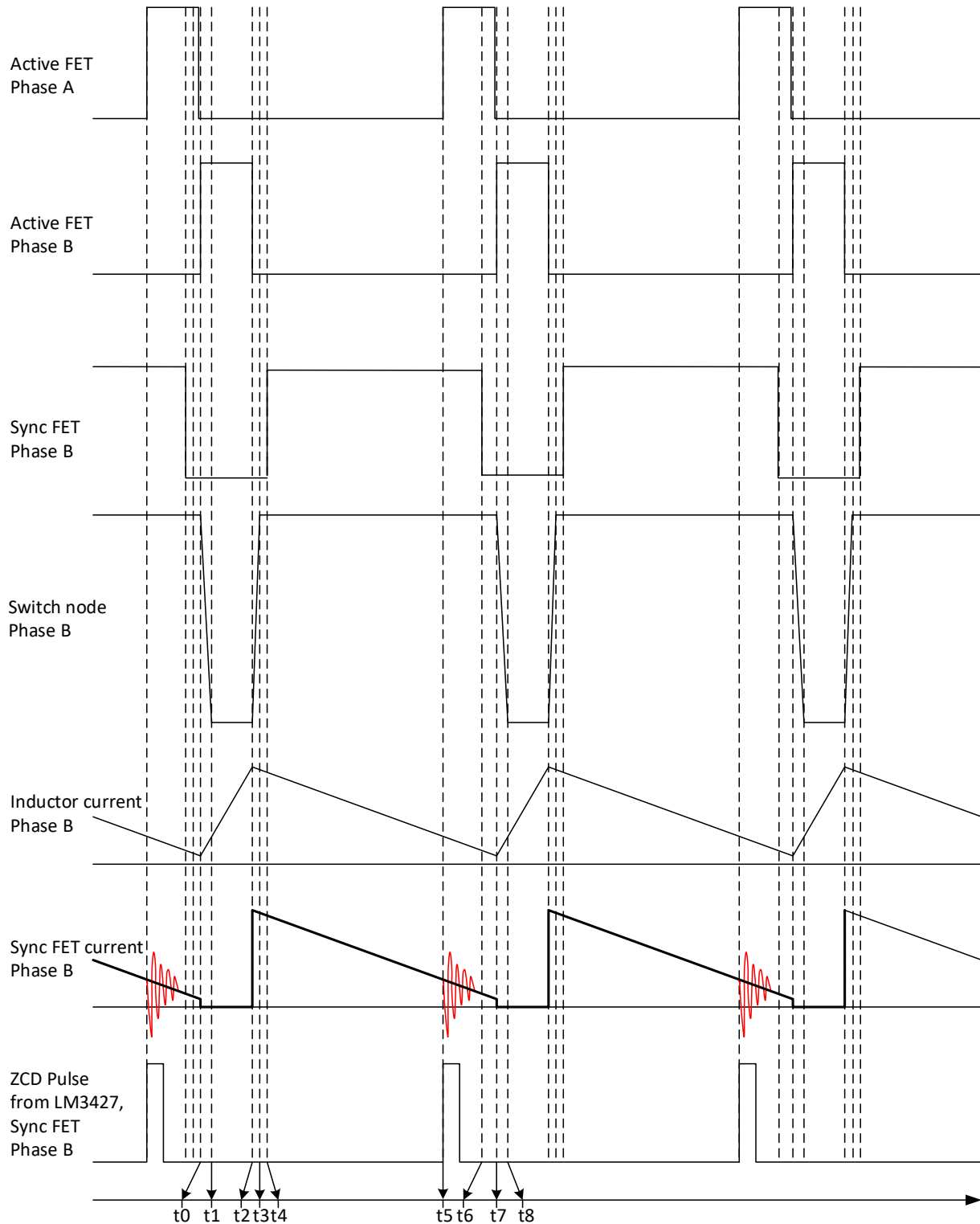
Figure 9. ZCD 问题时序
