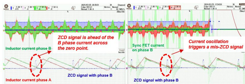
Figure 7. B 相 ZCD 信号在 B 相电流过零前提前发出
