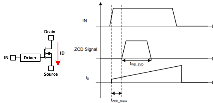
Figure 3. ZCD 脉冲时序，IN 引脚置高时刻且电流为正时
