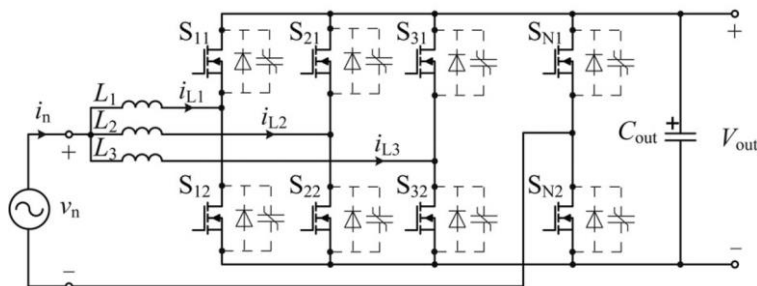
Figure 1. 三相交错 TCM PFC 拓扑结构
