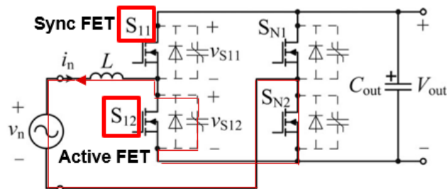
Figure 4. 单相 TCM PFC 运行结构
