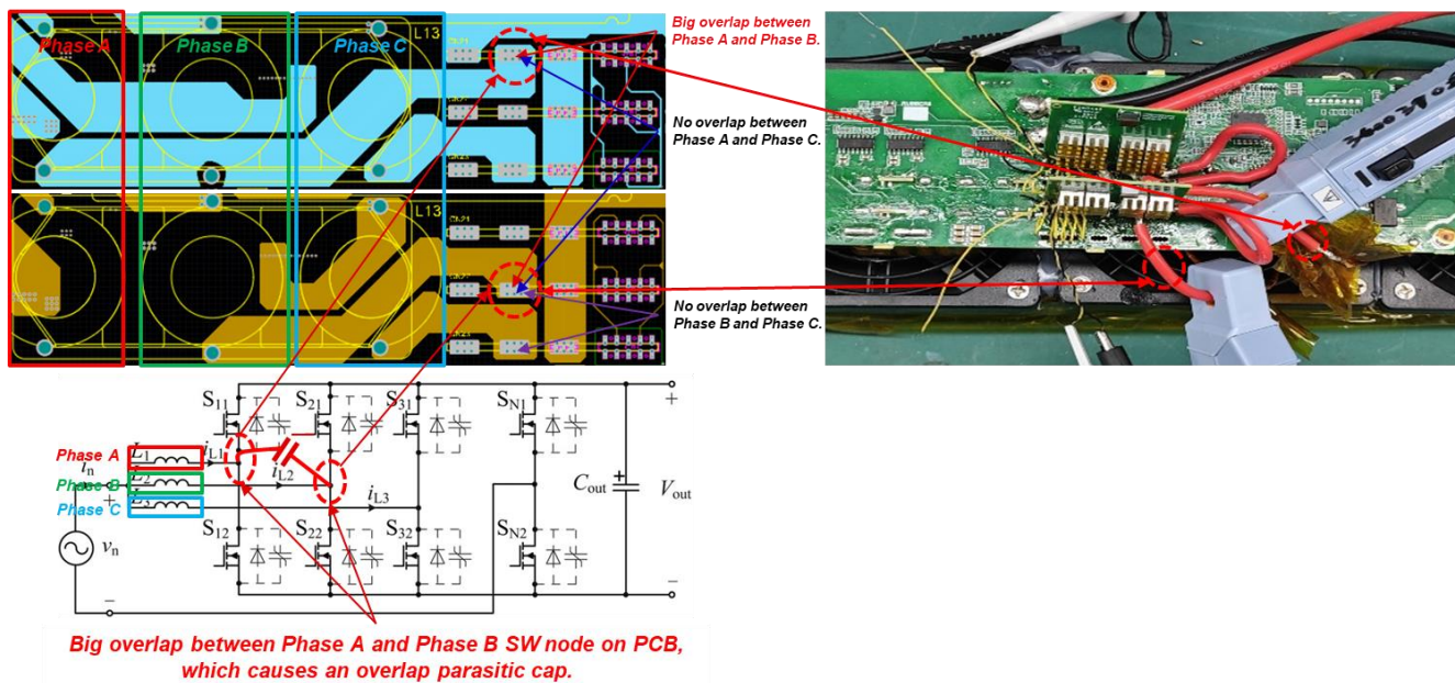
Figure 10. 通过外部飞线消除 A 相和 B 相间的重叠
