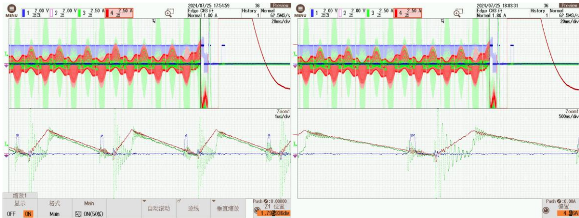
Figure 8. 问题波形，流经 B 相的电流的震荡造成了 B 相 ZCD 信号提前发出
