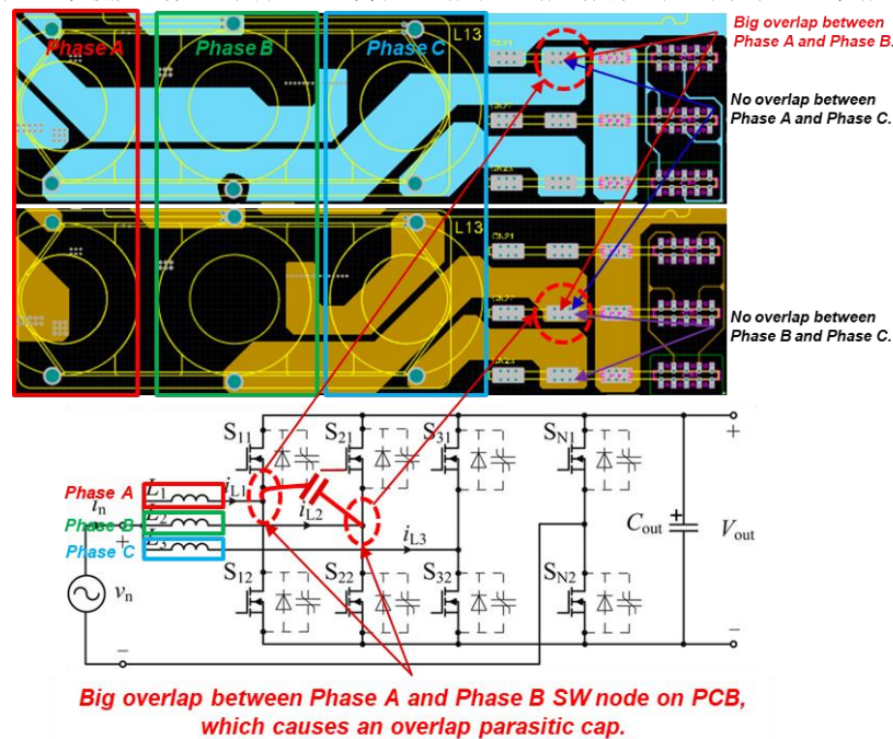
Figure 6. “不完美”的 PCB 设计, 相邻 SW 节点平面间存在大面积交叠
