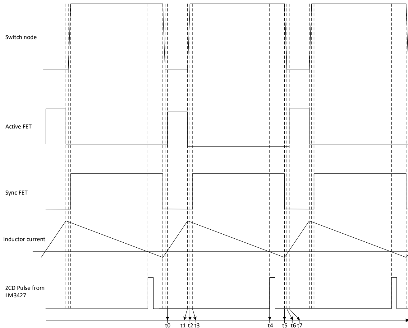
Figure 5. 基于 LMG3427 的 TCM PFC 的应用时序
