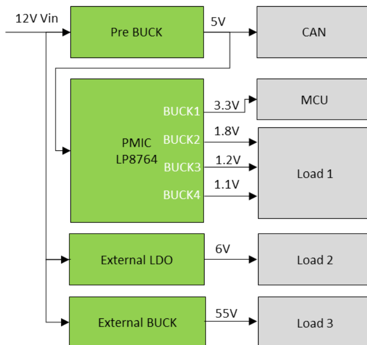
图 1-2. LP8764 自定义 NVM 案例系统架构
