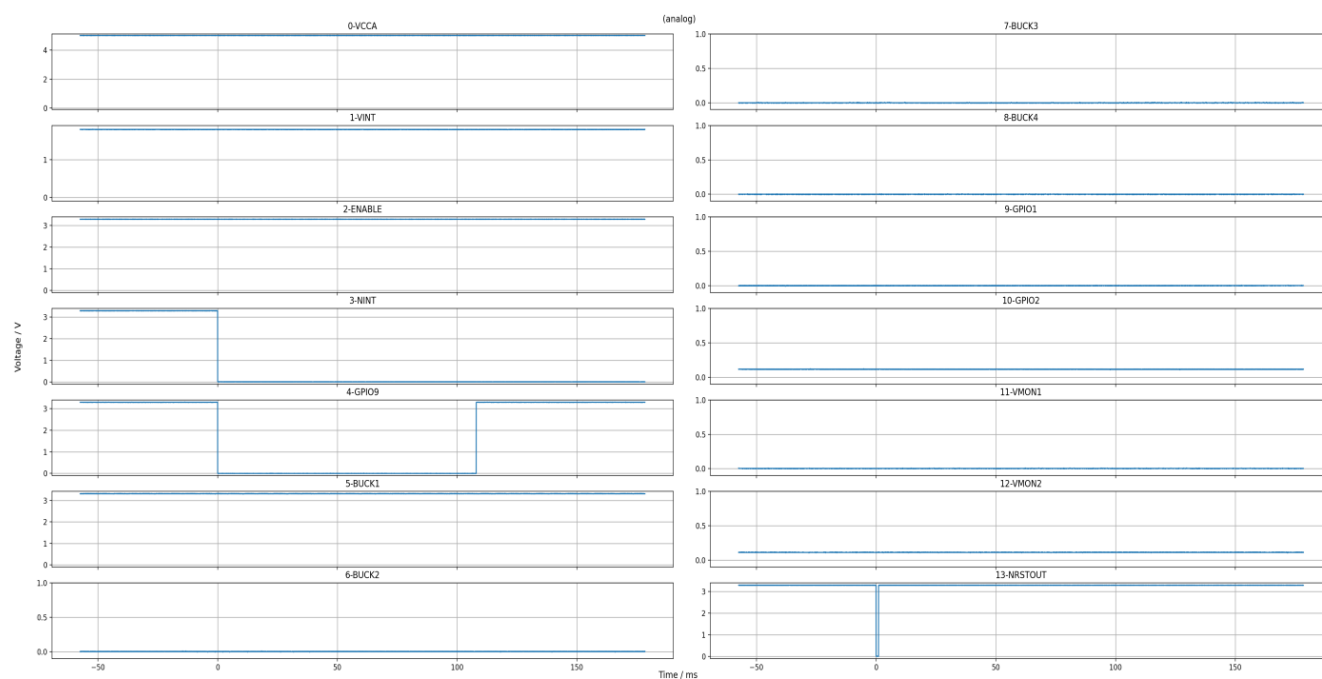
图 3-4. MCU2WARM 时序测试
