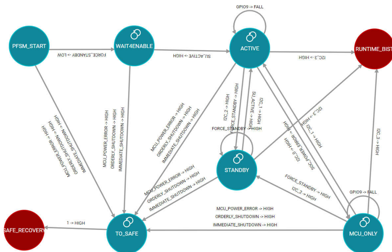
图 2-10. PFSM 设置
