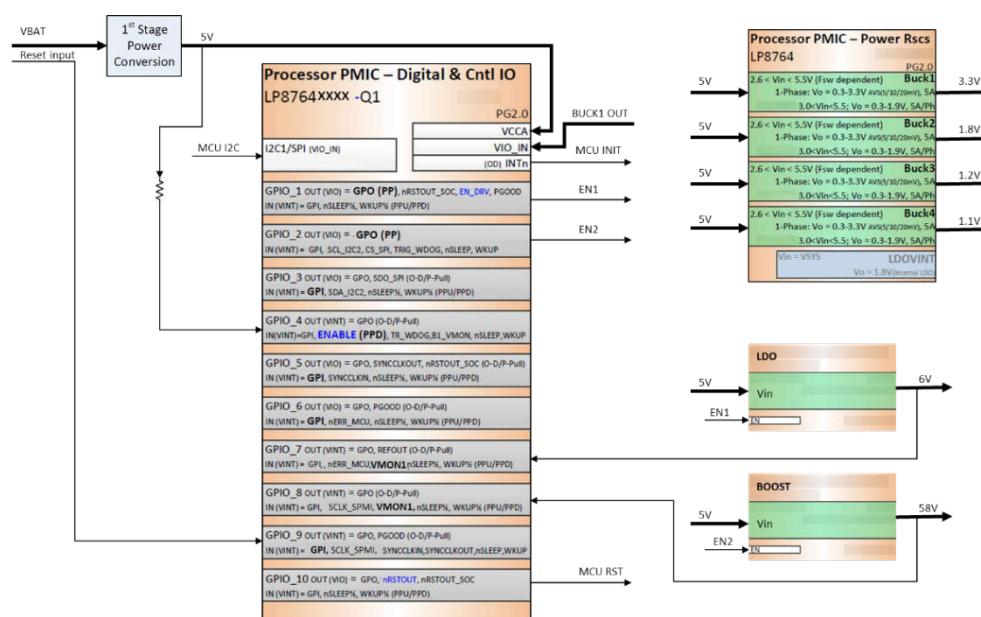
图 2-3. 系统电源架构方案
