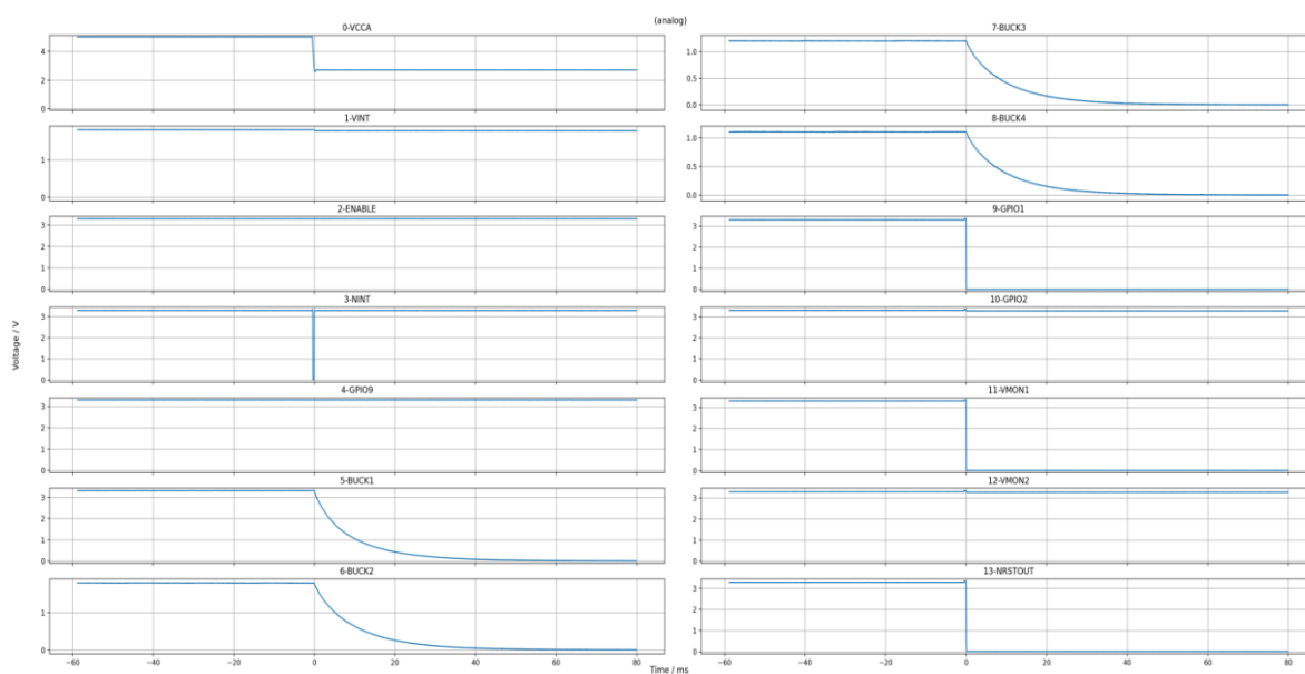
图 3-8. ACT2SAFE 时序测试
