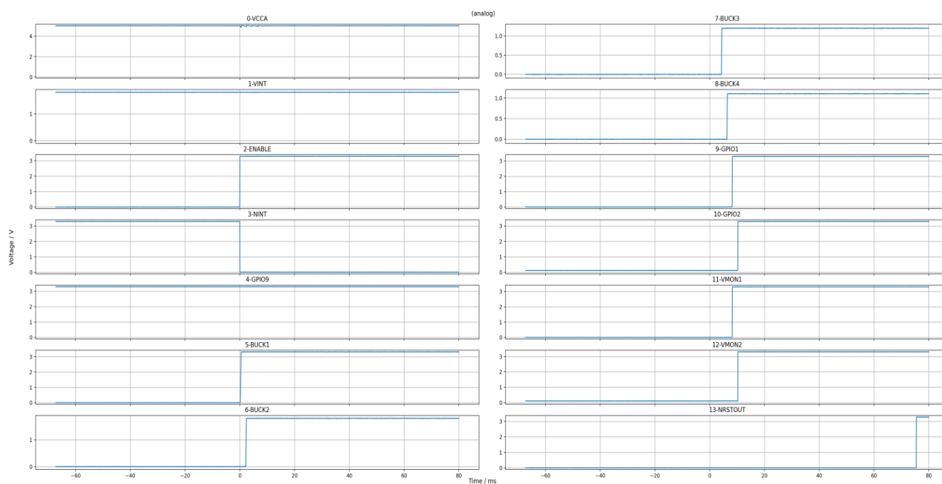
图 3-6. STANDBY2ACT 时序测试
