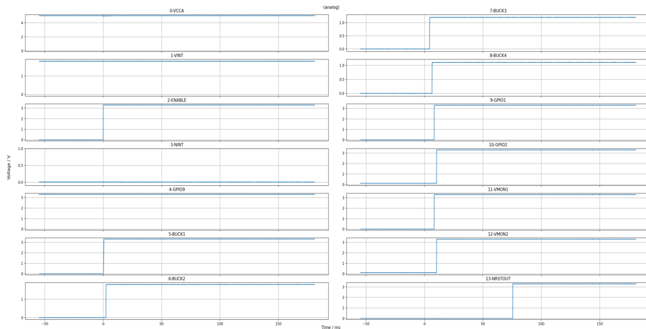
图 3-1. START2ACT 时序测试
