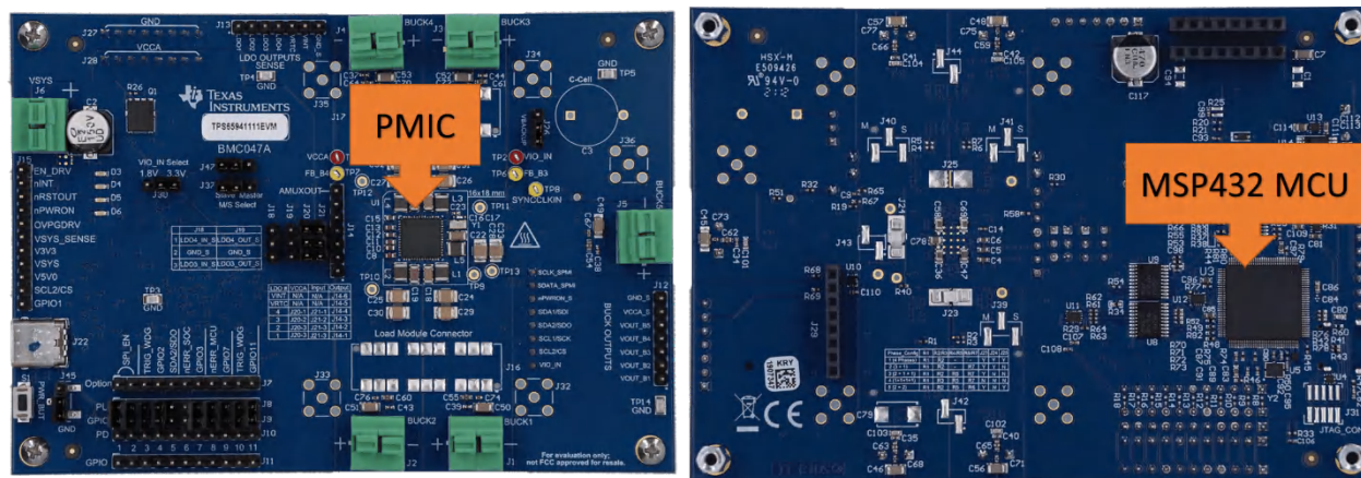
图 4-1. TPS6594 EVM 照片
