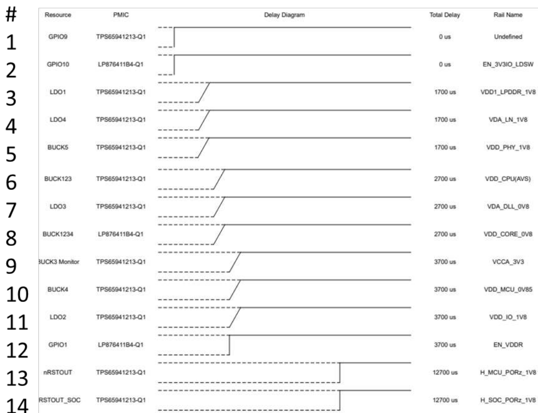
图 3-1. PDN 0A 上电时序
