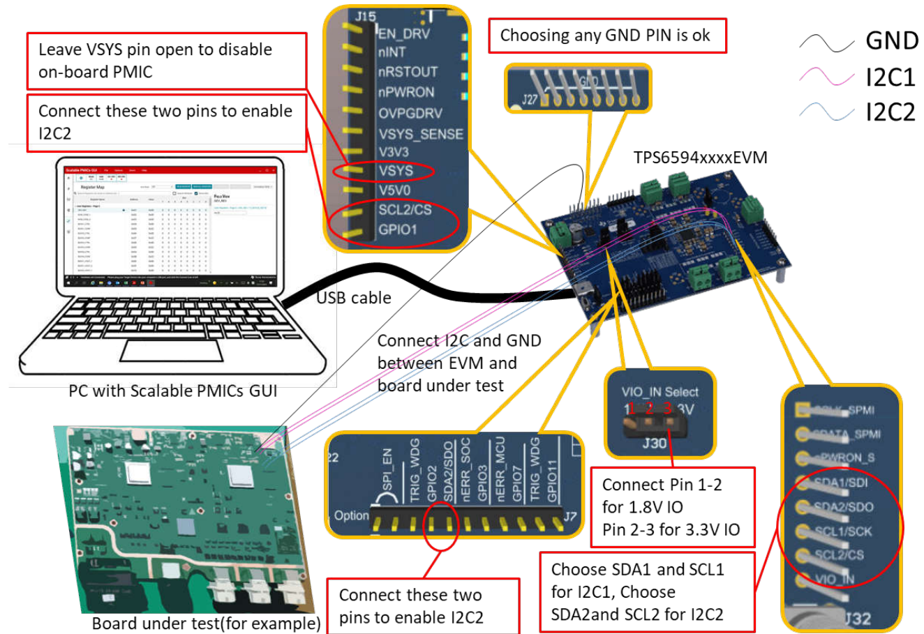
图 4-2. 使用 EVM 读取待测板 PMIC 寄存器示意图
