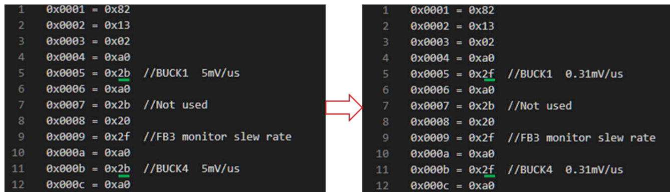
图 5-6. 修改 NVM bin 文件
