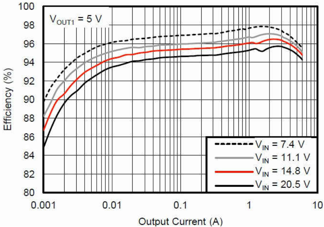
图 2-1. TPS51285A 效率图
