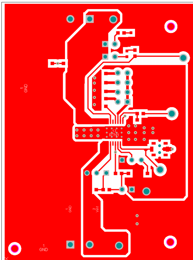
Figure 12. LM76202-Q1EVM Top Layer
