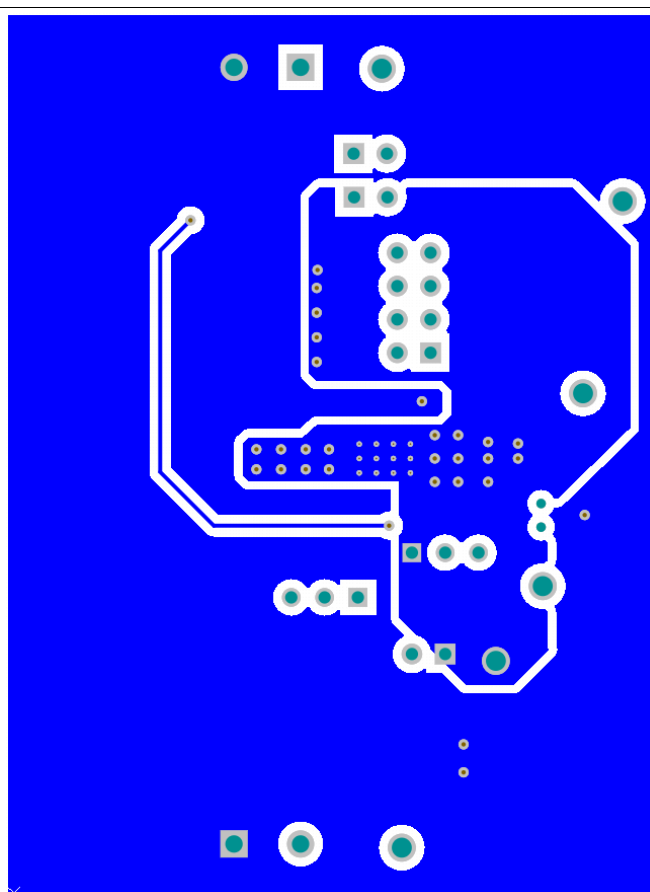
Figure 13. LM76202-Q1EVM Bottom Layer
