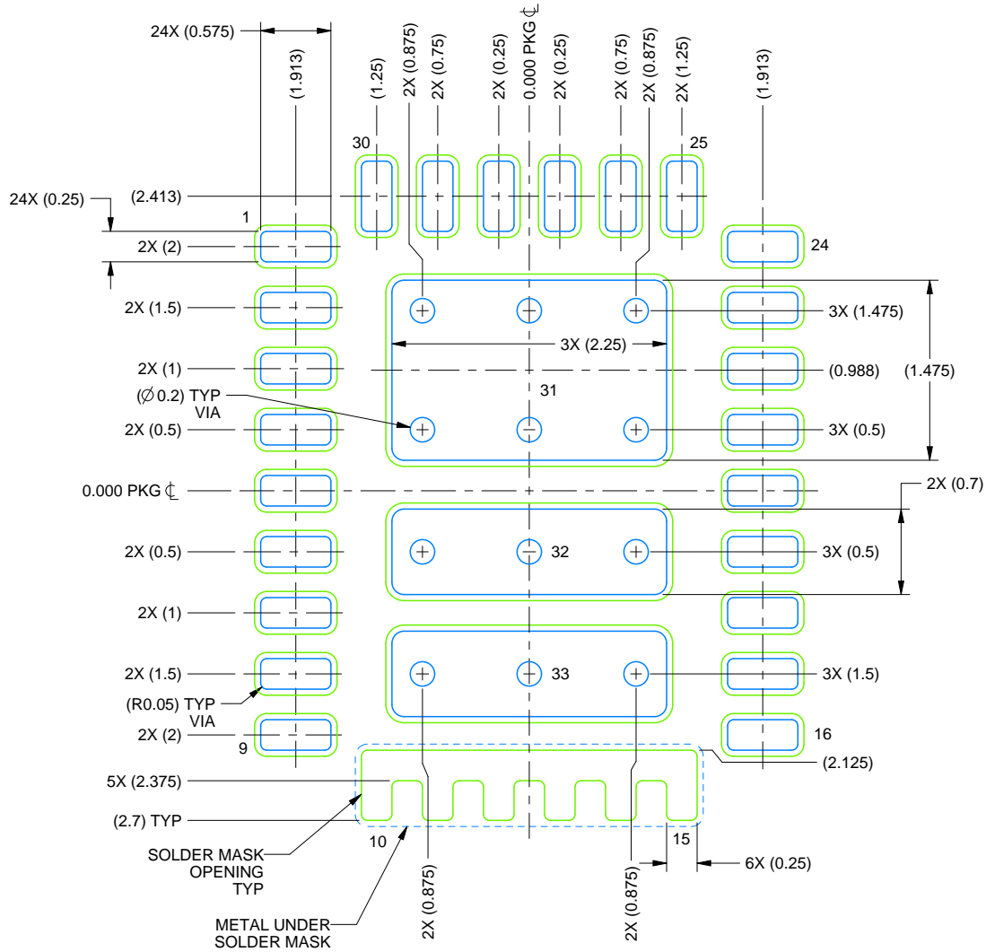
LAND PATTERN EXAMPLE SCALE: 18X
