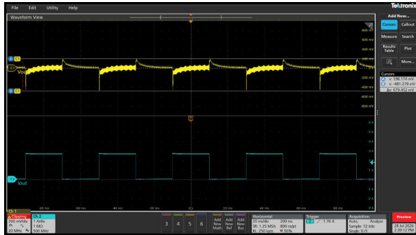
图 3-52. V_{OUT} = 24V 过冲/下冲= 198mV/-481mV 条件下的负载瞬态响应
