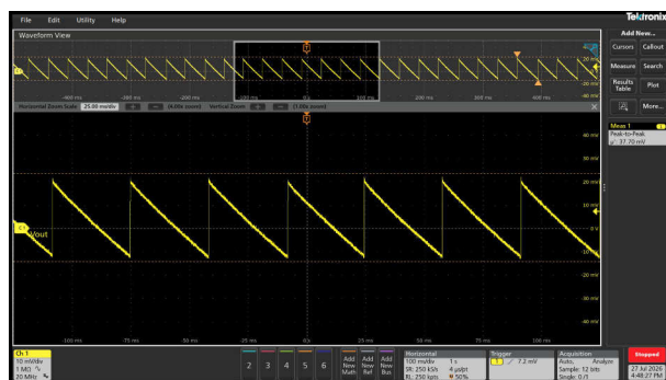
图 3-46. V_{OUT} = 12V 且无负载时的典型纹波电压 (38mVpp)
