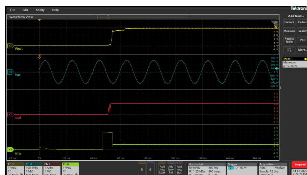
图 3-69. 5V 和 3A 下的启动响应
