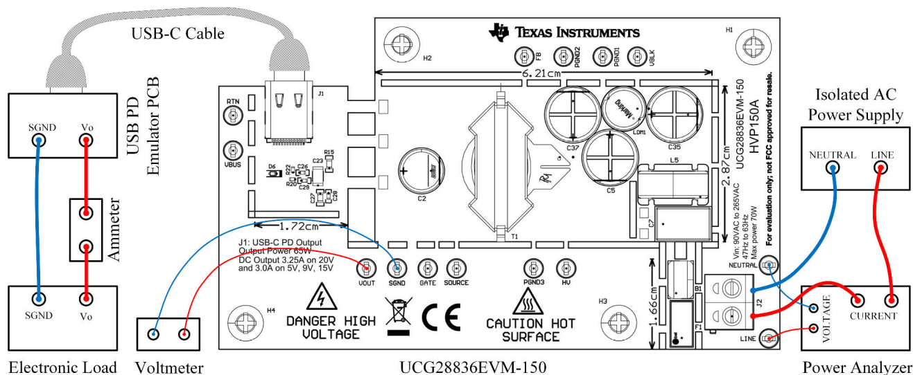
图 3-1. 使用 USB-C PD 负载的 UCG28836EVM-150 测试设置图
