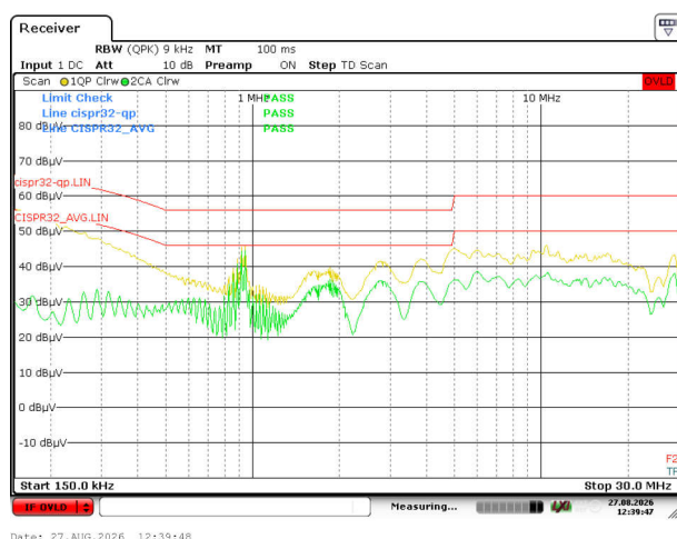
图 3-88. V_{IN} = 230V_{RMS} 、 V_{OUT} = 20V 且 I_{OUT} = 0.325A 时为火线
