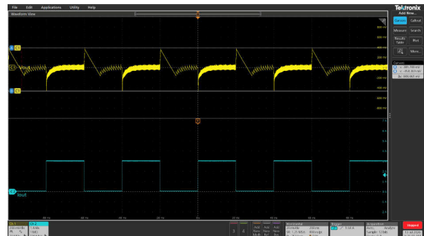
图 3-57. V_{OUT} = 5V 过冲/下冲= 390mV/-458mV 条件下的瞬态响应
