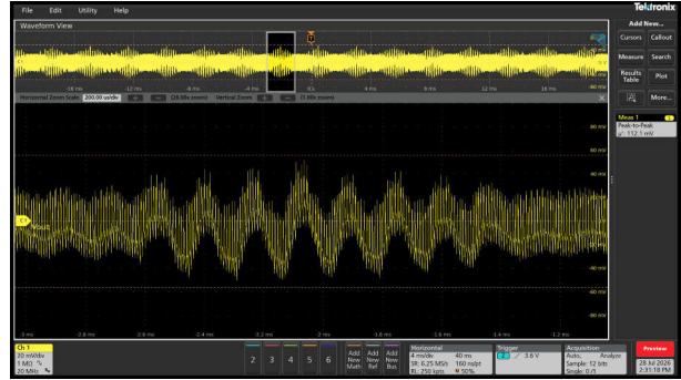
图 3-41. V_{OUT} = 24V 且满负载时的典型纹波电压 (112mVpp)
