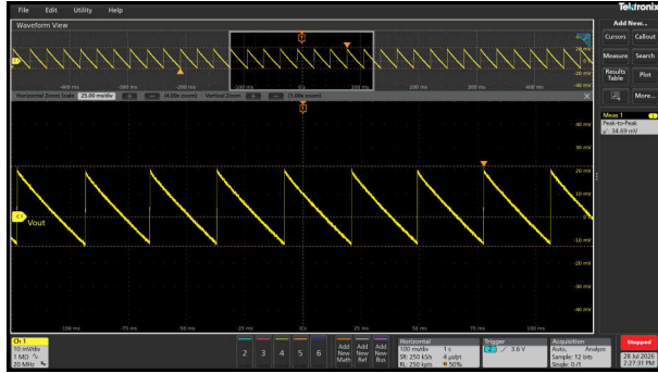
图 3-40. V_{OUT} = 24V 且无负载时的典型纹波电压 (35mVpp)
