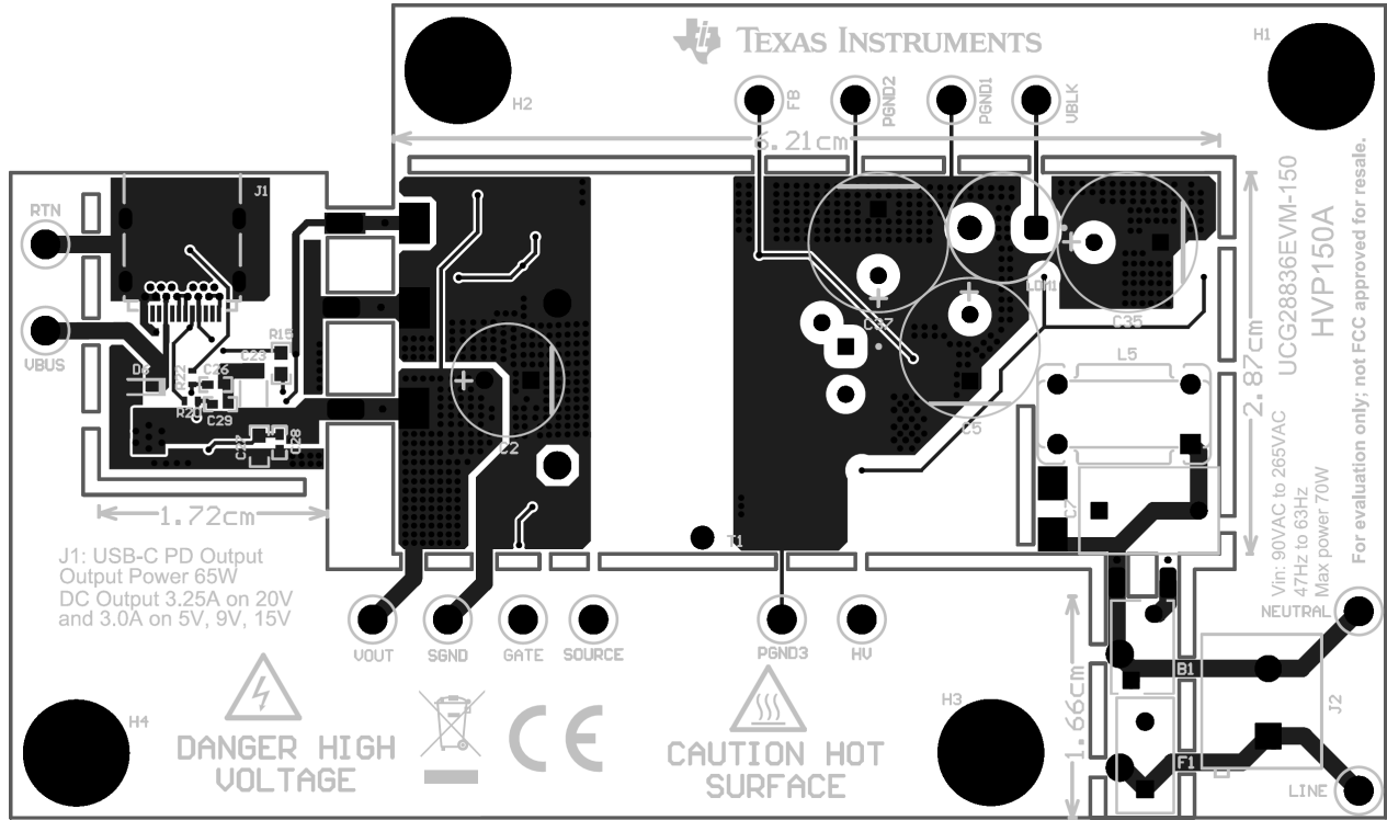
图 4-3. 顶层
