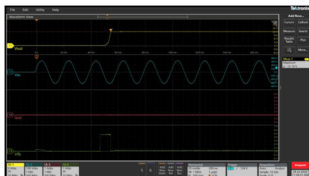
图 3-66. 12V 和 0A 下的启动响应
