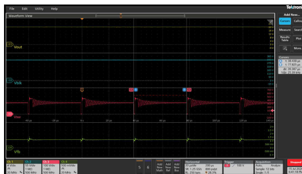
图 3-35. 230Vac/4.4W ( 25kHz 频率-折返/Vfb - 1.15V )
