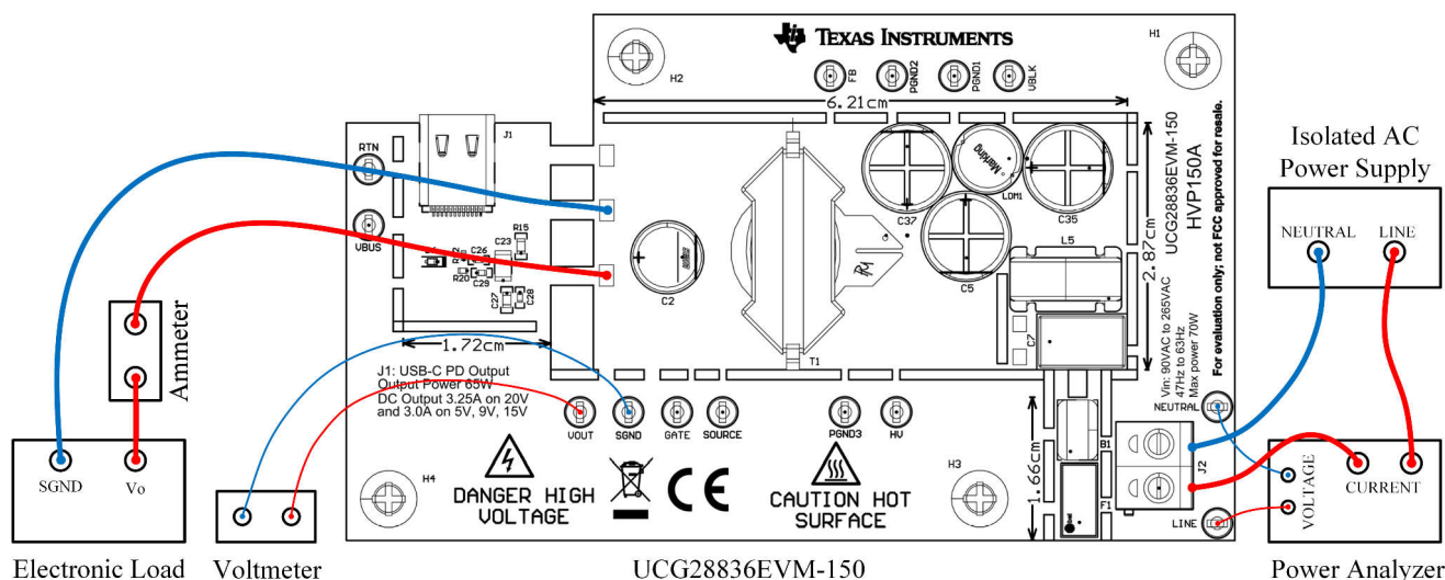
图 3-2. 使用非 USB-C PD 负载的 UCG28836EVM-150 测试设置图
