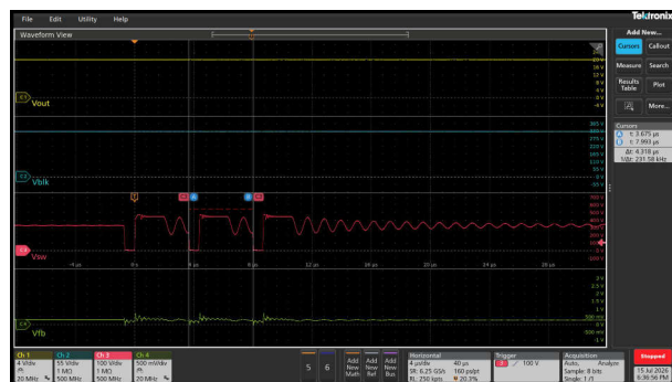
图 3-34. 230Vac/0.4W ( 231kHz 突发频率/Vfb - 0.26V )
