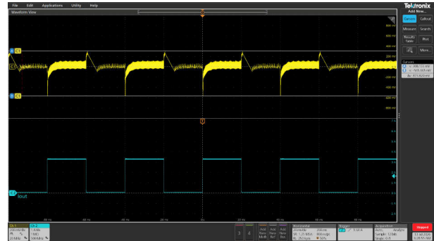
图 3-53. V_{OUT} = 20V 过冲/下冲= 308mV/-566mV 条件下的瞬态响应
