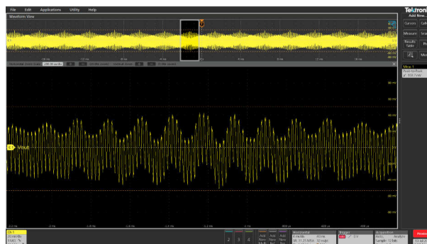
图 3-51. V_{OUT} = 5V 且满负载时的典型纹波电压 (104mVpp)
