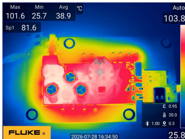
图 3-70. 顶面为 90Vac 至 24V/2.71A
