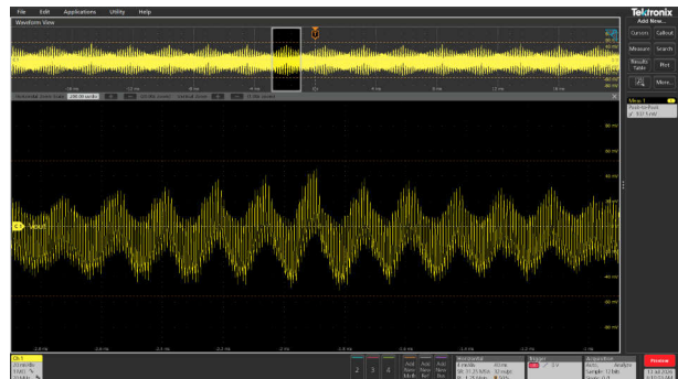
图 3-43. V_{OUT} = 20V 且满负载时的典型纹波电压 (108mVpp)
