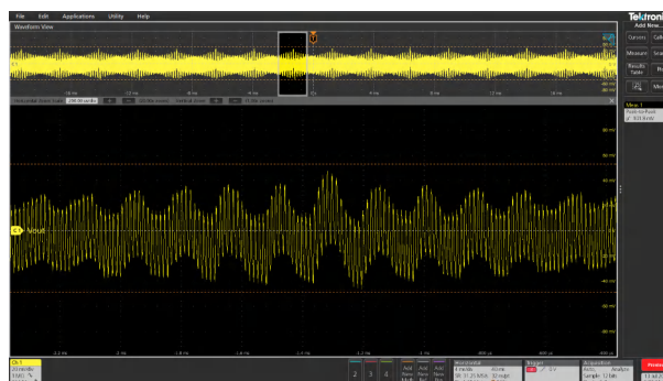
图 3-49. V_{OUT} = 9V 且满负载时的典型纹波电压 (102mVpp)
