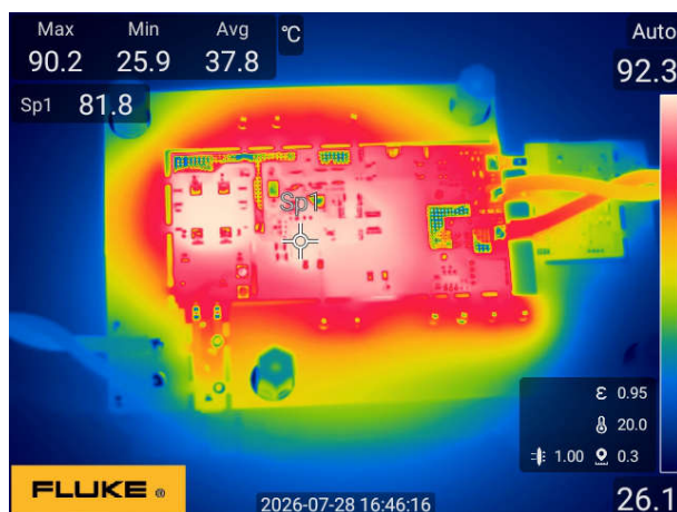
图 3-73. 底面为 115Vac 至 24V/2.71A
