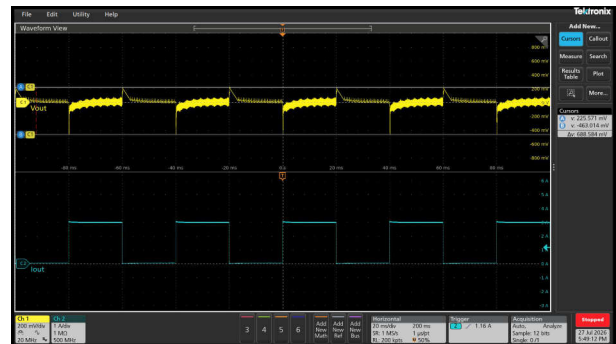
图 3-55. V_{OUT} = 12V 过冲/下冲= 225mV/-463mV 条件下的瞬态响应
