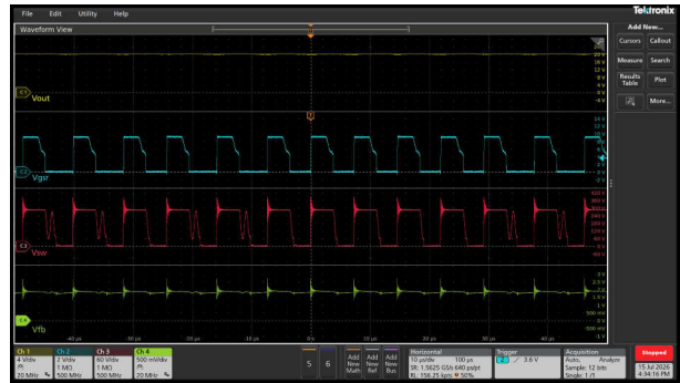
图 3-15. V_{in} = 115\text{Vac} , V_{out} = 20\text{V}
