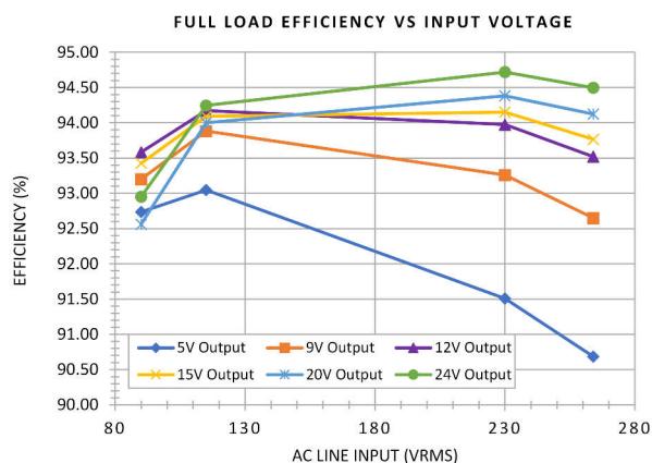
图 3-6. 满负载效率与输入电压间的关系
