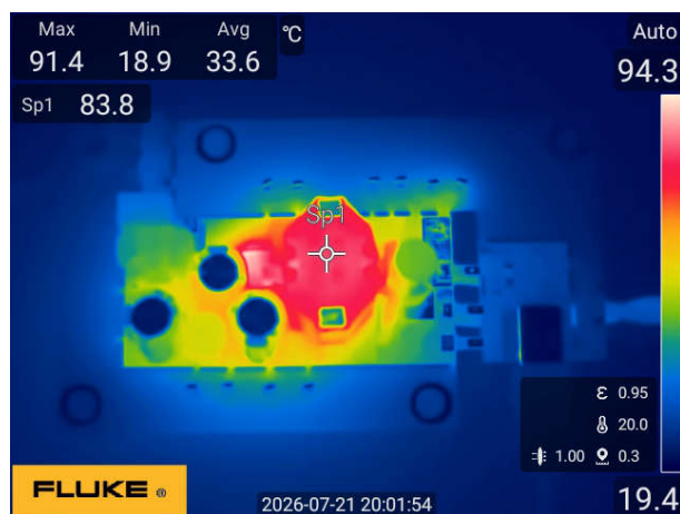
图 3-84. 顶面为 264Vac 至 20V/3.25A
