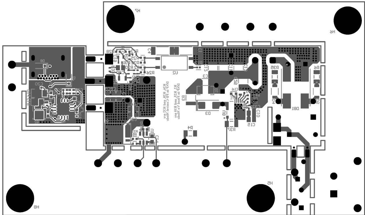
图 4-4. 底层
