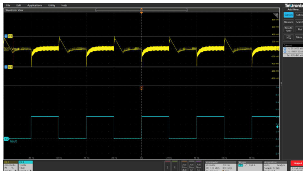
图 3-56. V_{OUT} = 9V 过冲/下冲= 351mV/-488mV 条件下的瞬态响应
