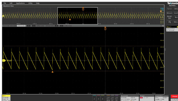
图 3-44. V_{OUT} = 15V 且无负载时的典型纹波电压 (75mVpp)
