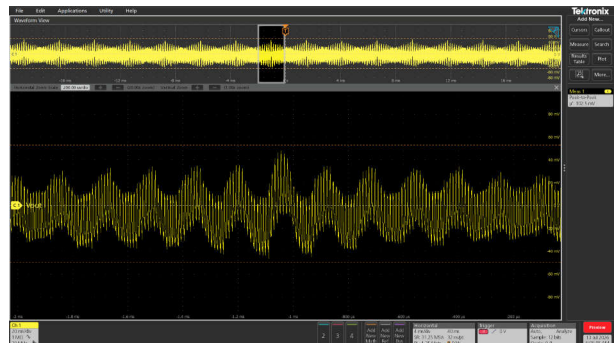
图 3-45. V_{OUT} = 15V 且满负载时的典型纹波电压 (103mVpp)
