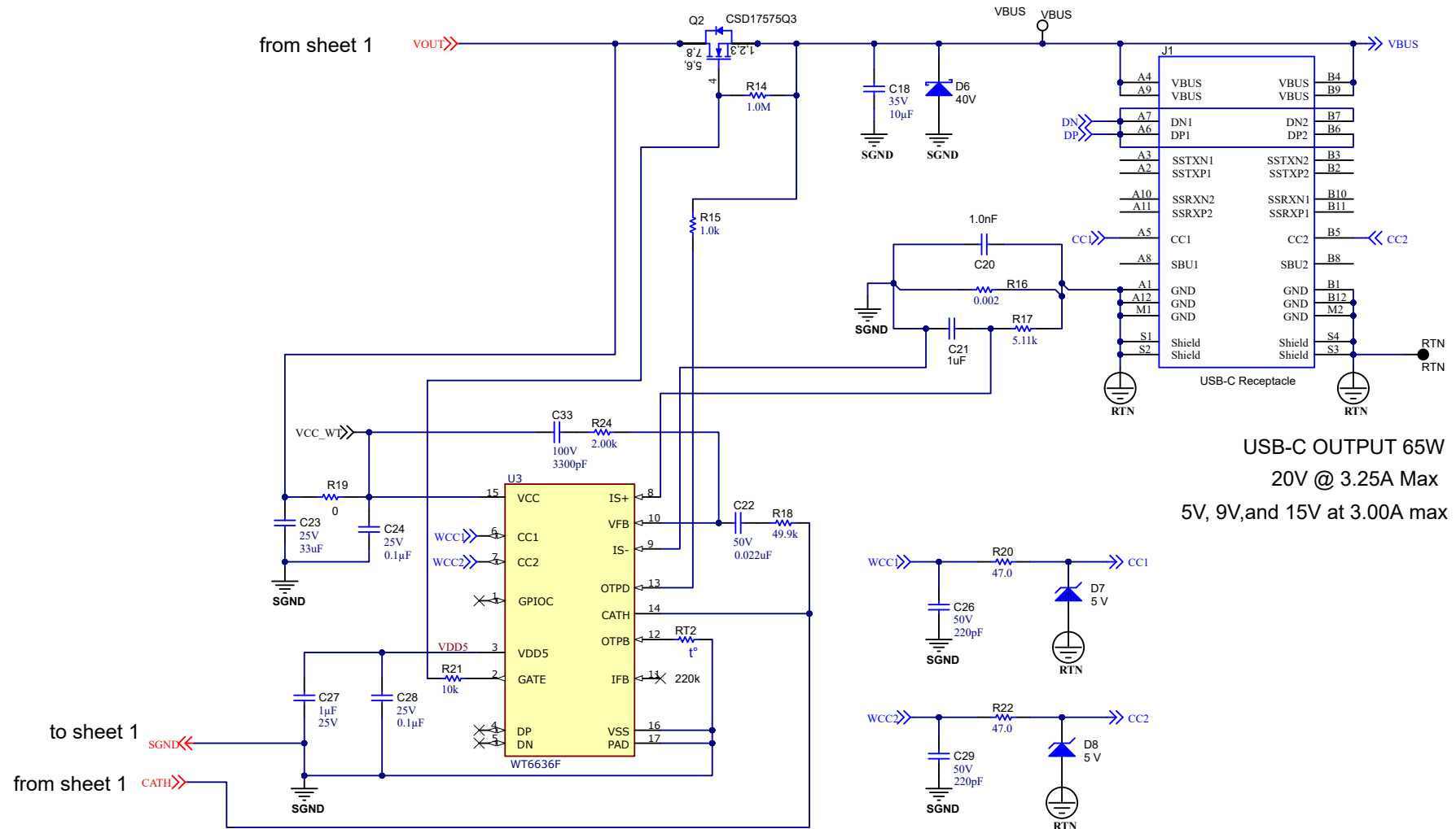
图 4-2. UCG28836EVM-150 PD 控制器电路原理图
