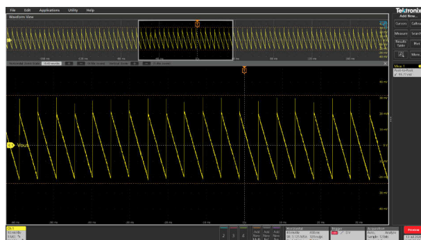
图 3-48. V_{OUT} = 9V 且无负载时的典型纹波电压 (56mVpp)
