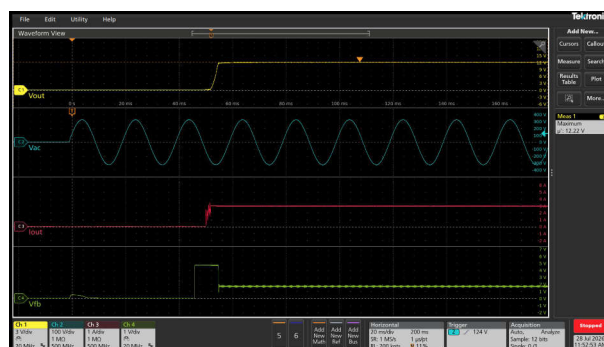
图 3-67. 12V 和 3A 下的启动响应
