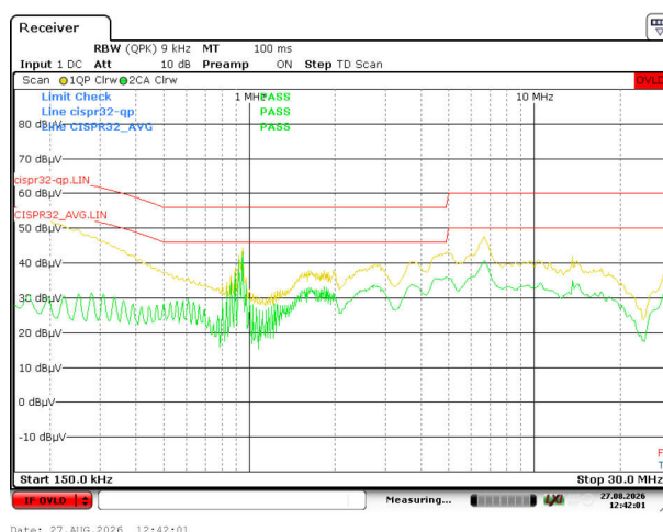
图 3-89. V_{IN} = 230V_{RMS} 、 V_{OUT} = 20V 、 I_{OUT} = 0.325A 时为零线
