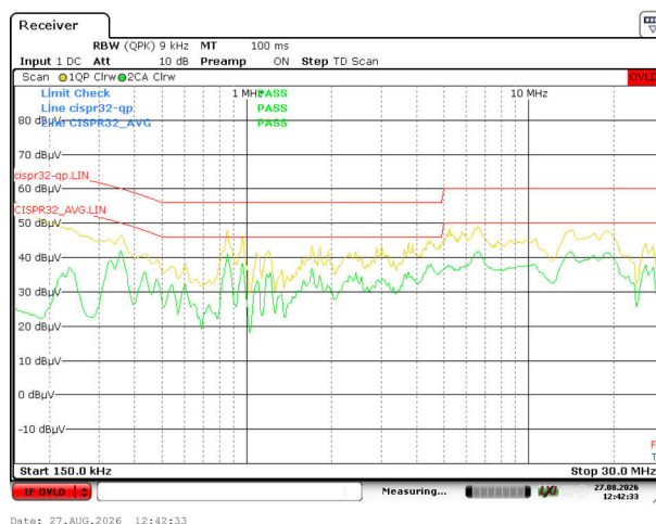
图 3-87. V_{IN} = 230V_{RMS} 、 V_{OUT} = 20V 、 I_{OUT} = 3.25A 时为零线
