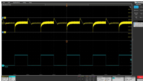
图 3-54. V_{OUT} = 15V 过冲/下冲= 312mV/-523mV 条件下的瞬态响应
