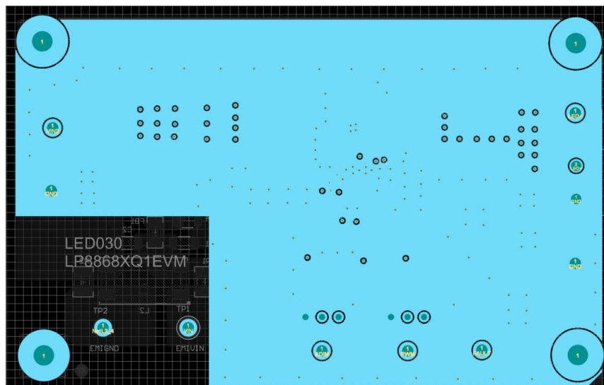
图 3-4. LP8868XQ1EVM 内层 2
