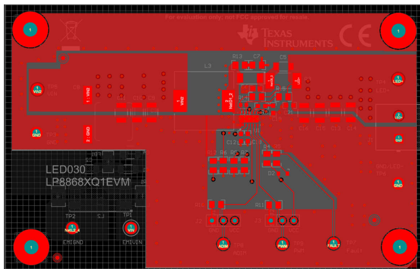
图 3-2. LP8868XQ1EVM 顶层
