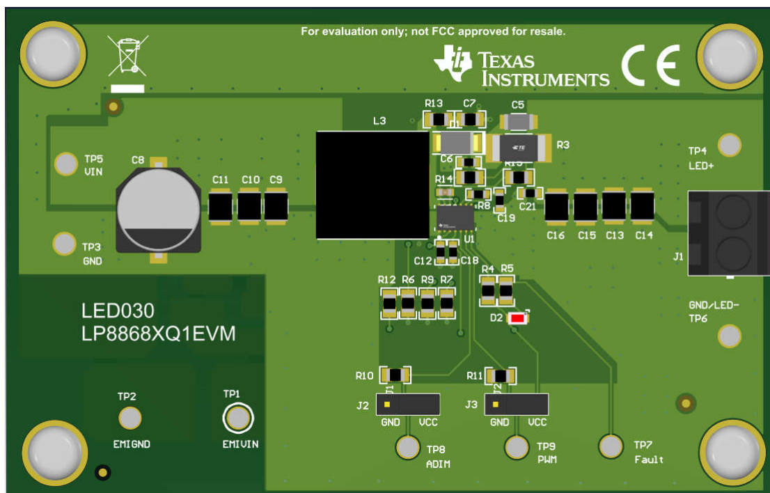
图 1-1. LP8868XQ1EVM 套件
