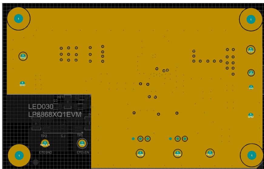
图 3-3. LP8868XQ1EVM 内层 1
