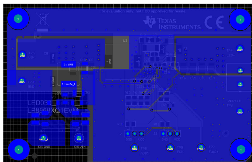
图 3-5. LP8868XQ1EVM 底层
