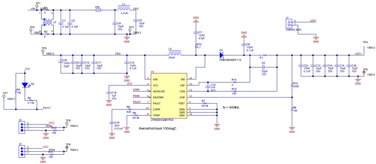
图 3-1. LP8868XQ1EVM 原理图
