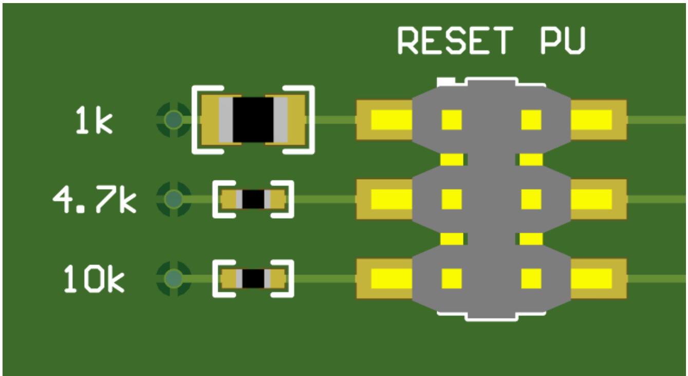
图 2-5. 接头 3x2 复位 PU : 顶部 ( 复位-1k )、中间 ( 复位-4.7k )、底部 ( 复位-10k )
