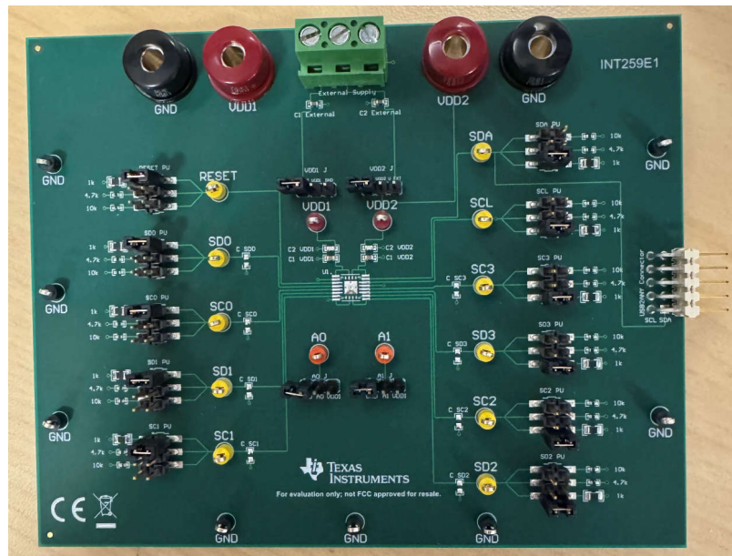
TCA984649-EVM (顶视图)
