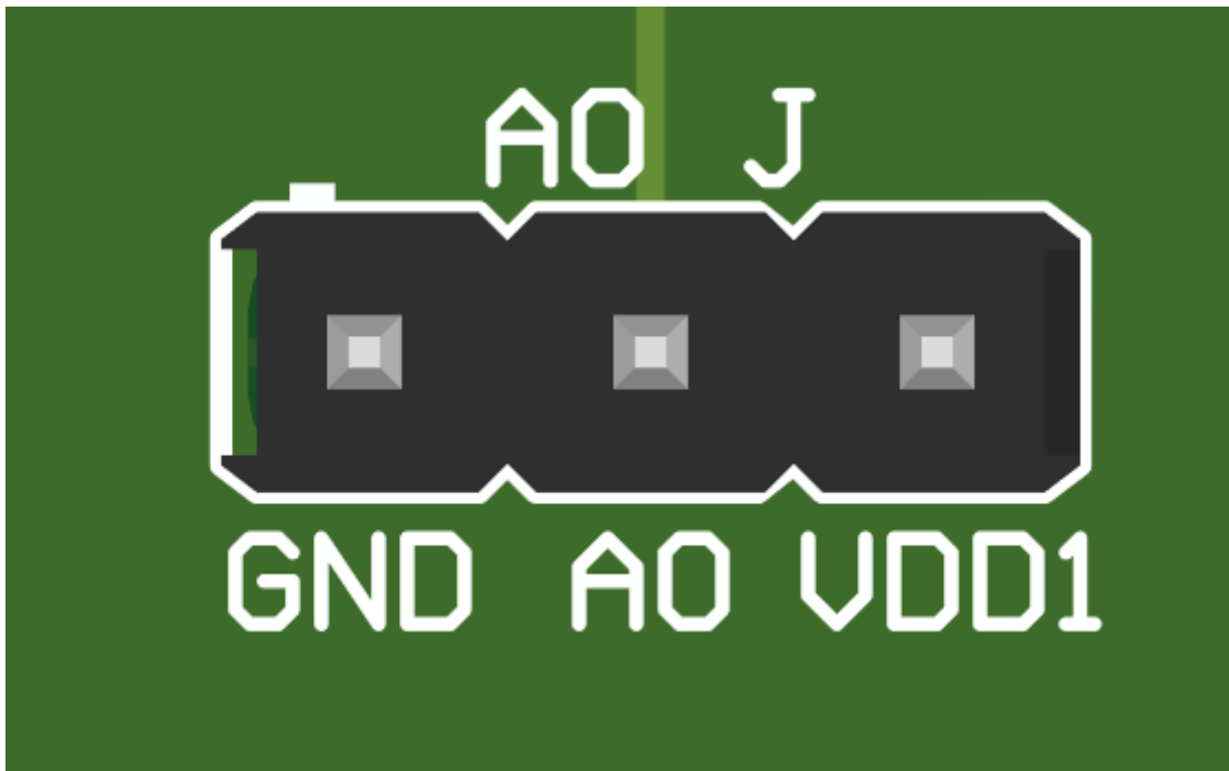
图 2-3. 接头 A0 J : J-1 (GND)、J-2 ( 连接到器件 A0 )、J-3 (VDD1)
