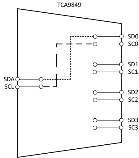
图 1-2. TCA9849 简化电路
