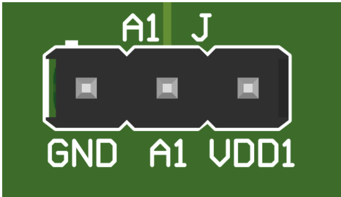
图 2-4. 接头 A1 J : J-1 (GND)、J-2 ( 连接到器件 A1 )、J-3 (VDD1)
