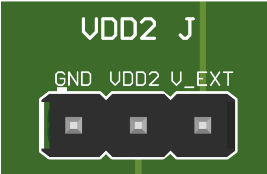
图 2-2. 接头 VDD2 J : J-1 ( GND )、J-2 ( 连接到器件 VDD2 )、J-3 ( 外部电源 )
