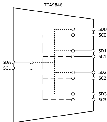
图 1-1. TCA9846 简化电路
