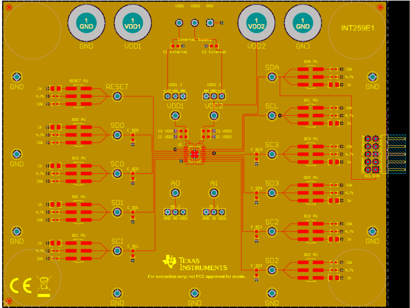
图 3-2. TCA984649-EVM 顶层布局
