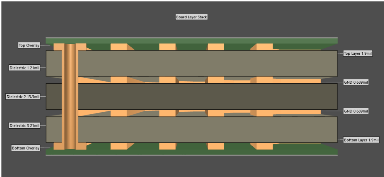
图 3-6. TRF2001PEVM 堆叠 (以 mil 为单位)
