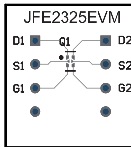
图 3-2. JFE2325EVM PCB 布局复合视图 ( 顶视图 )
