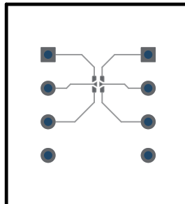
图 3-3. JFE2325EVM PCB 顶层掩膜
