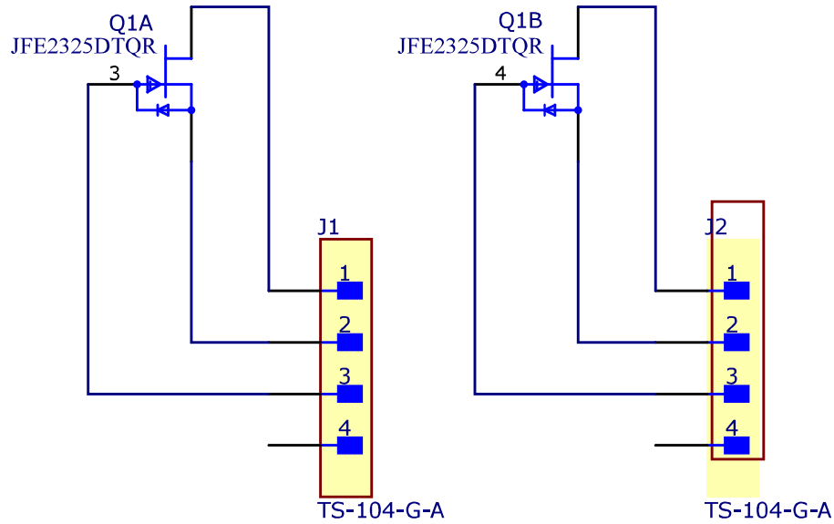
图 3-1. JFE2325EVM 原理图
