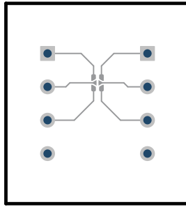
图 3-4. JFE2325EVM PCB 顶层
