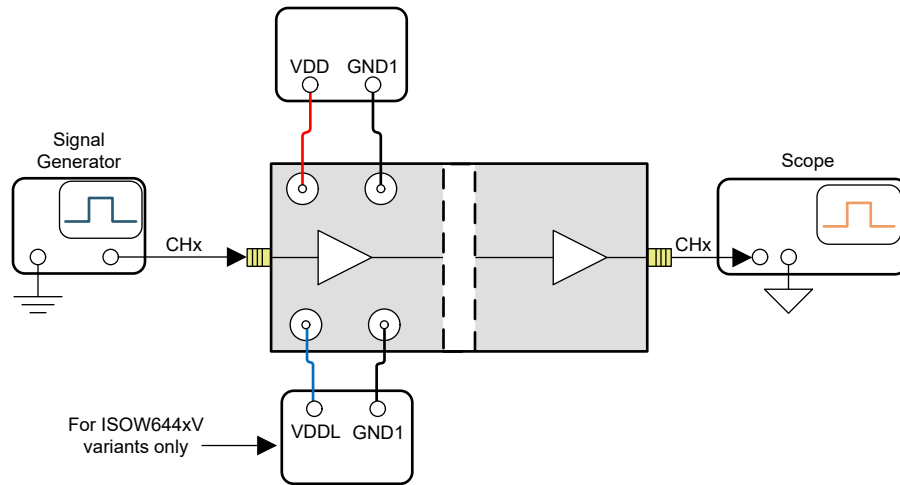
图 2-3. EVM 典型测试设置
