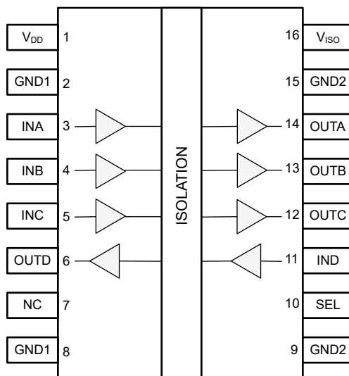
图 2-1. ISOW6441 具有集成式直流/直流转换器的四通道数字隔离器引脚配置
