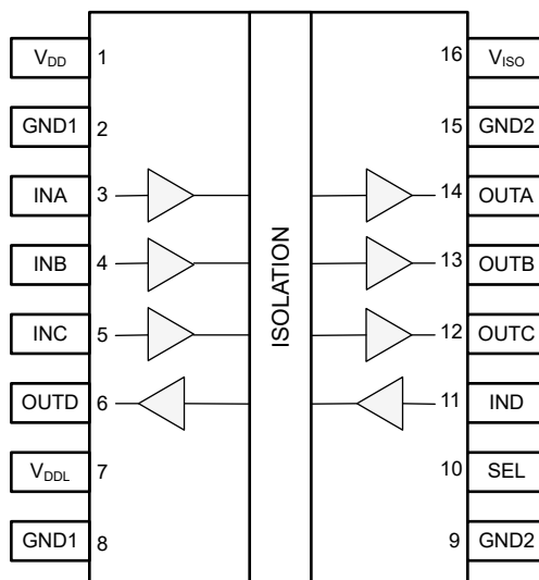
图 2-2. ISOW6441V 具有集成式直流/直流转换器的四通道数字隔离器引脚配置
