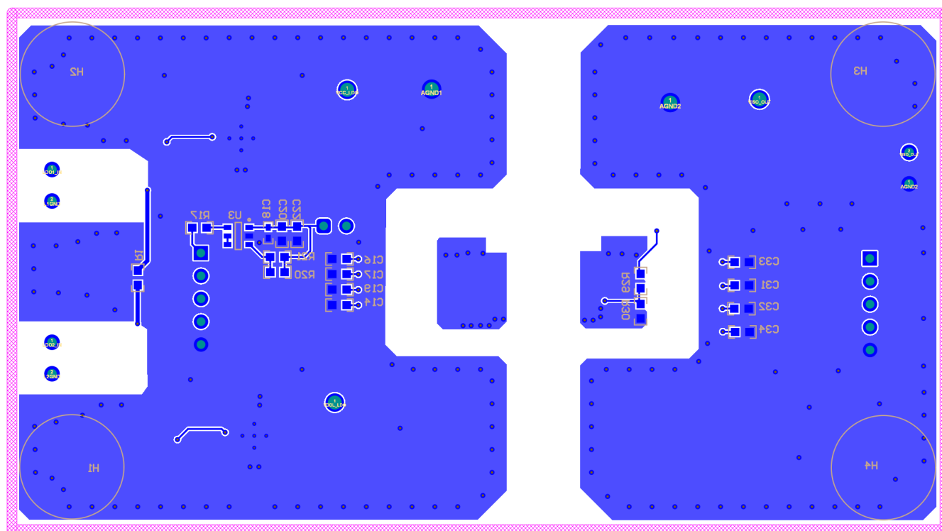
图 3-3. ISOW6441DWEEVM PCB 布局 - 底层
