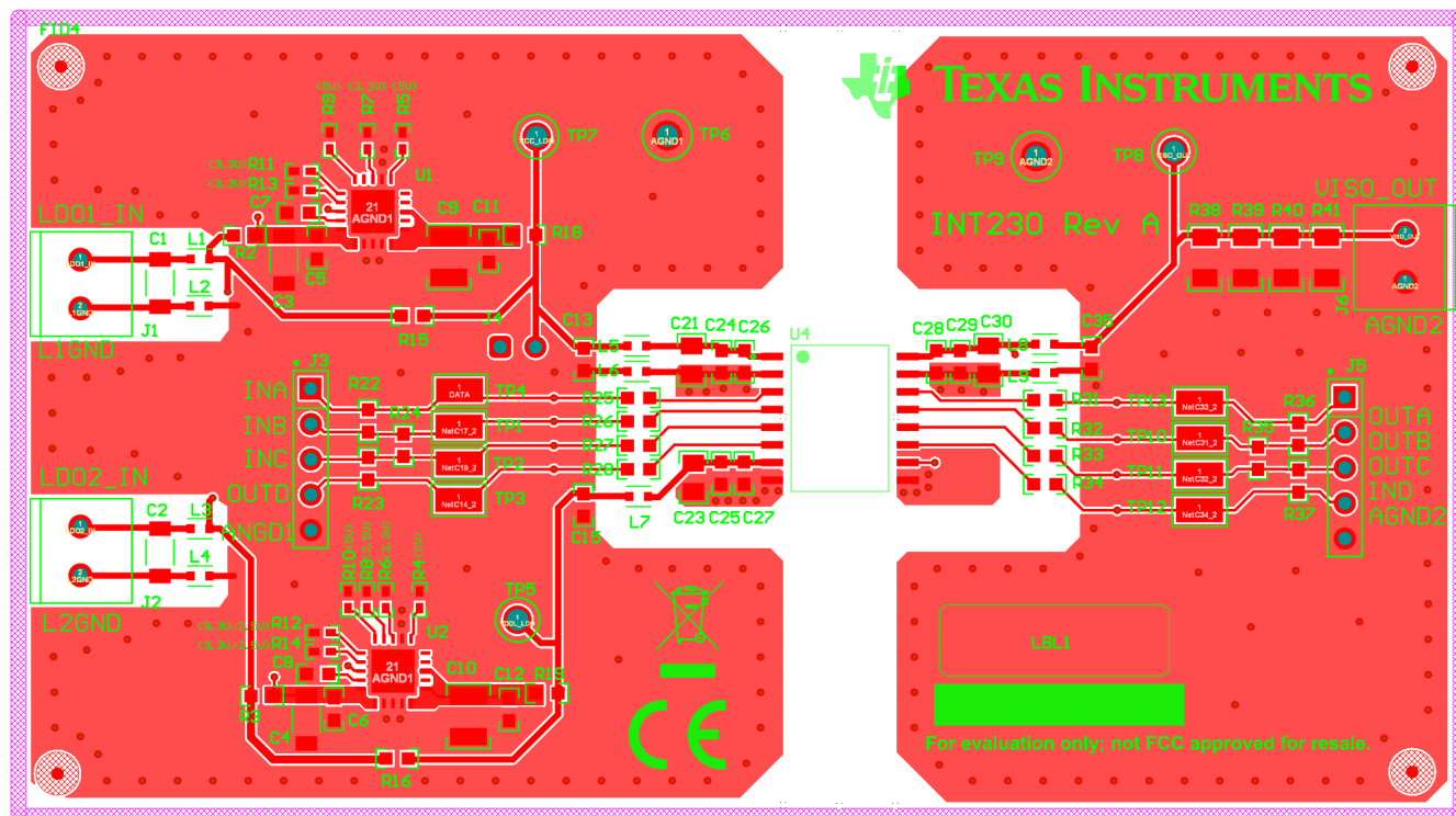
图 3-2. ISOW6441DWEEVM PCB 布局 - 顶层
