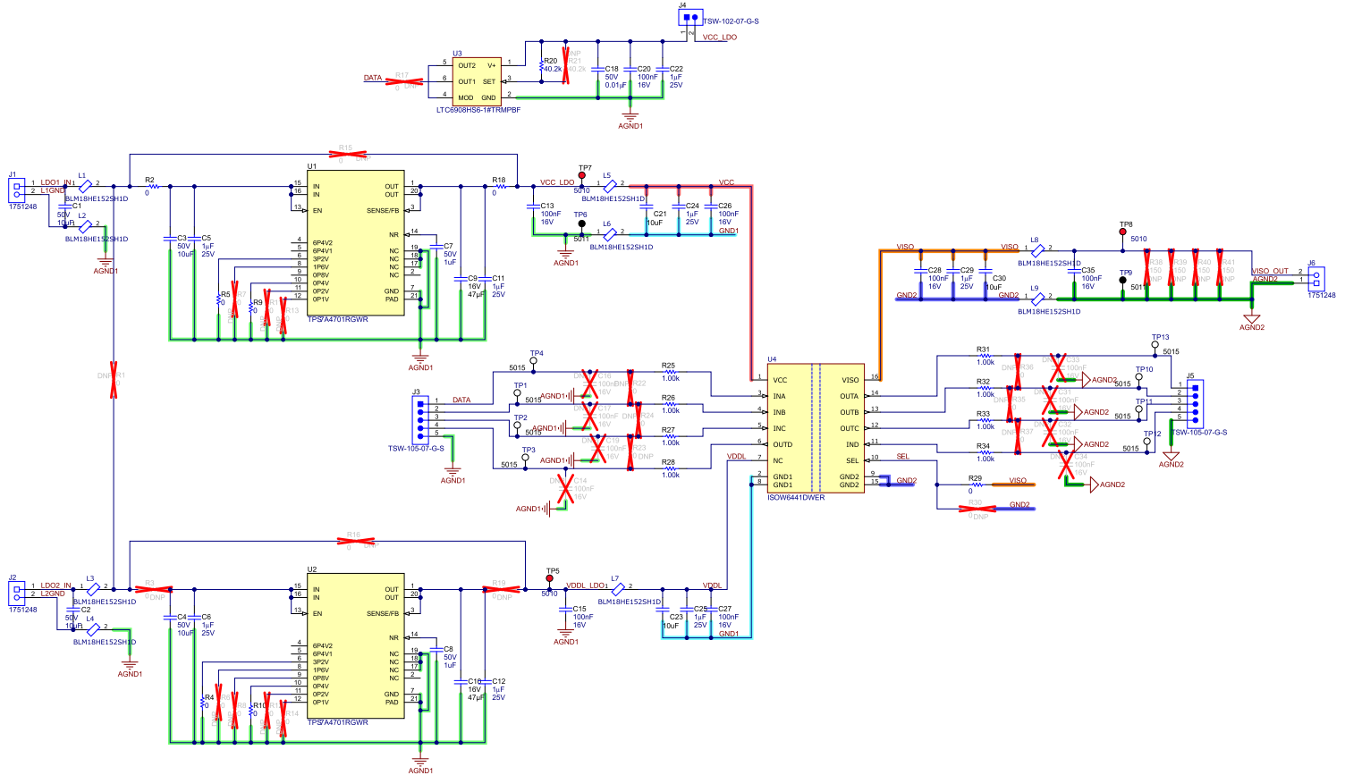
图 3-1. ISOW6441DWEEVM 原理图
