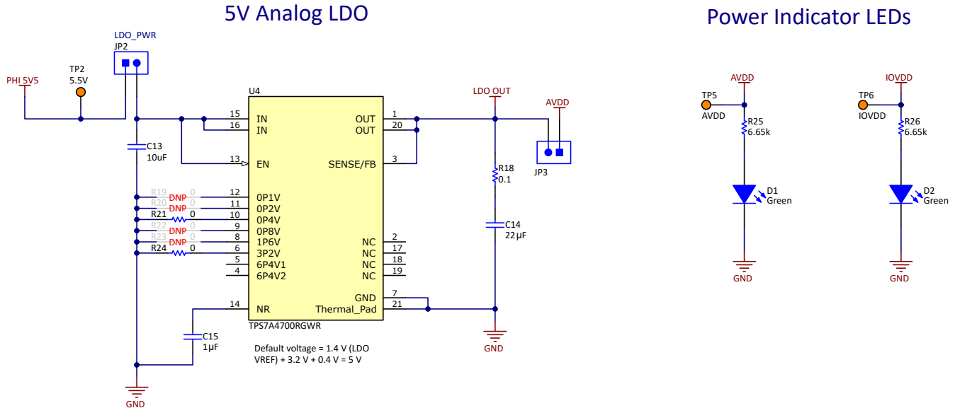
图 2-4. EVM 电源
