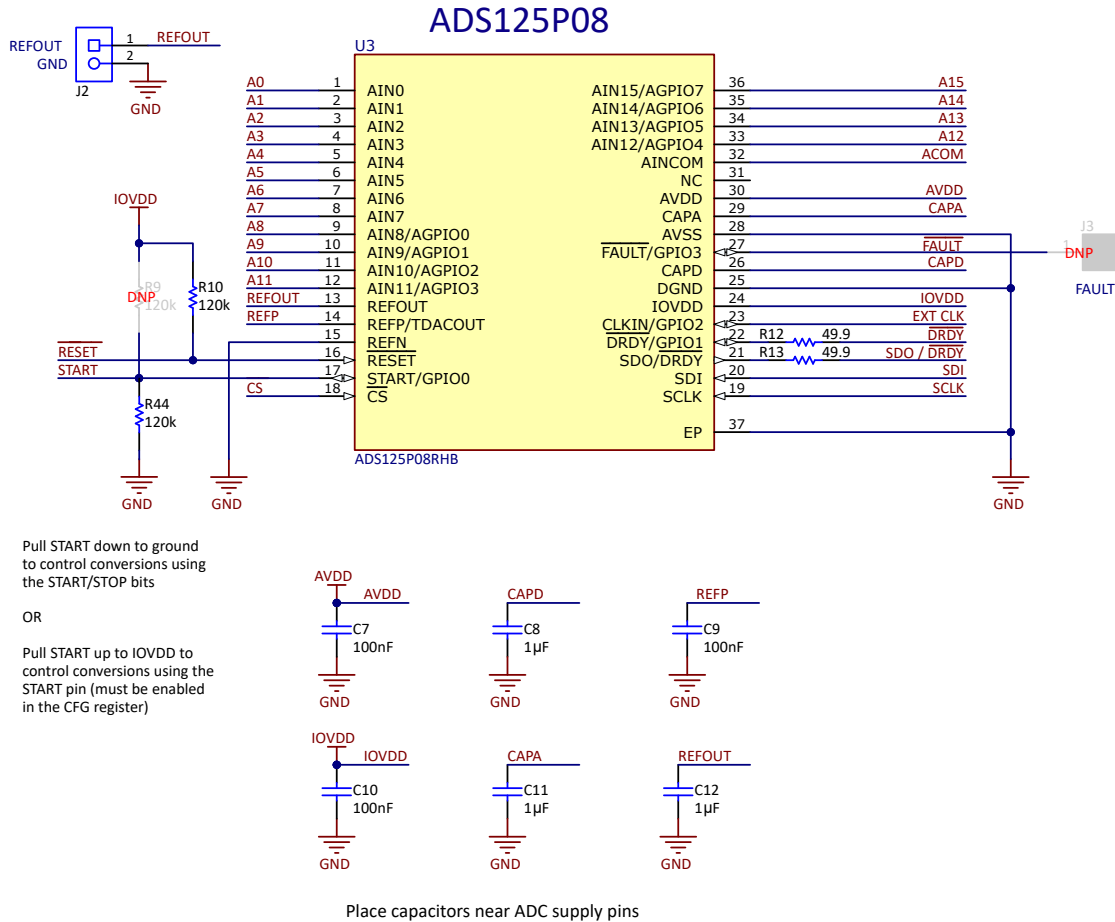
图 2-2. ADC 连接和去耦
