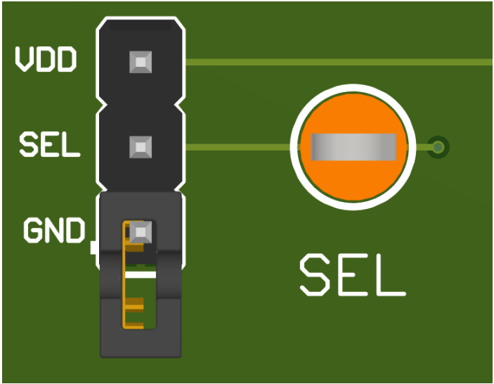
图 2-2. 接头 SEL J : J-1 (VDD)、J-2 ( 连接到器件 SEL )、J-3 (GND)
