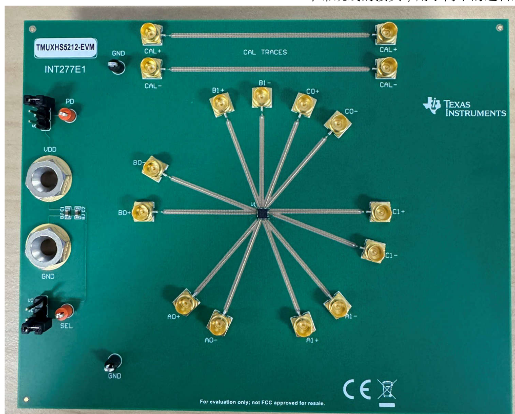
TMUXHS5212-EVM ( 顶视图 )
