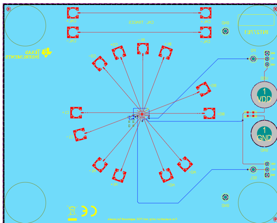
图 3-3. TMUXHS5212-EVM 底层布局
