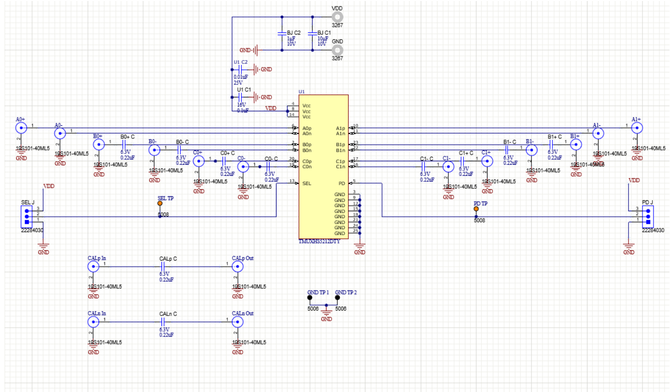
图 3-1. TMUXHS5212-EVM 原理图
