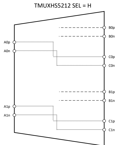
图 1-2. TMUXHS5212 SEL = H 简化电路
