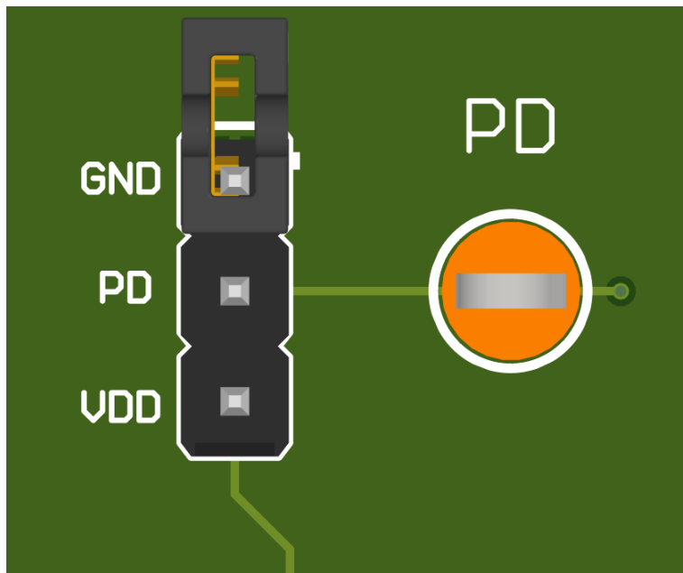
图 2-1. 接头 PD J : J-1 (GND)、J-2 ( 连接到器件 PD )、J-3 (VDD)
