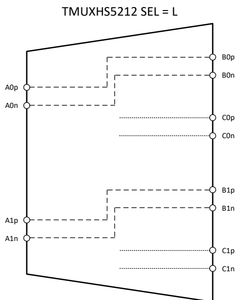
图 1-1. TMUXHS5212 SEL = L 简化电路
