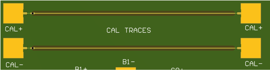
图 2-3. 校准走线
