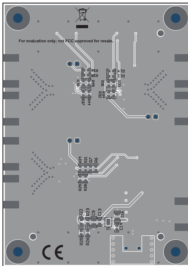
图 5-7. 底视图 (复合)
