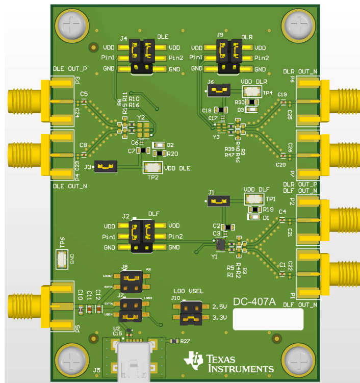
LMK6LEVM 评估板
