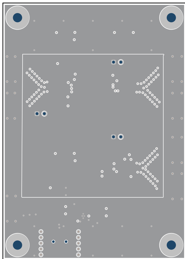
图 5-6. PWR 层
