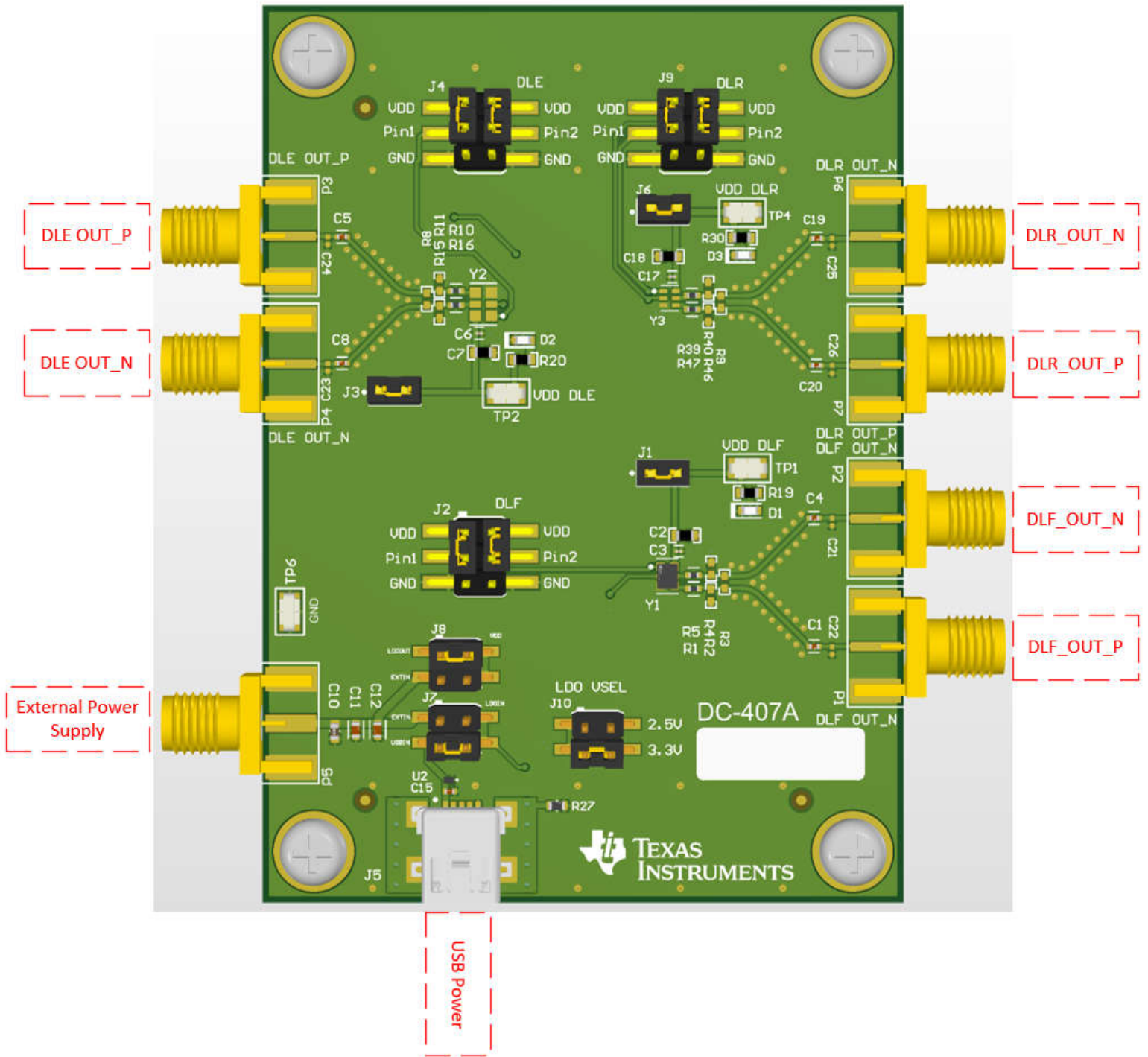
图 4-1. 连接图
