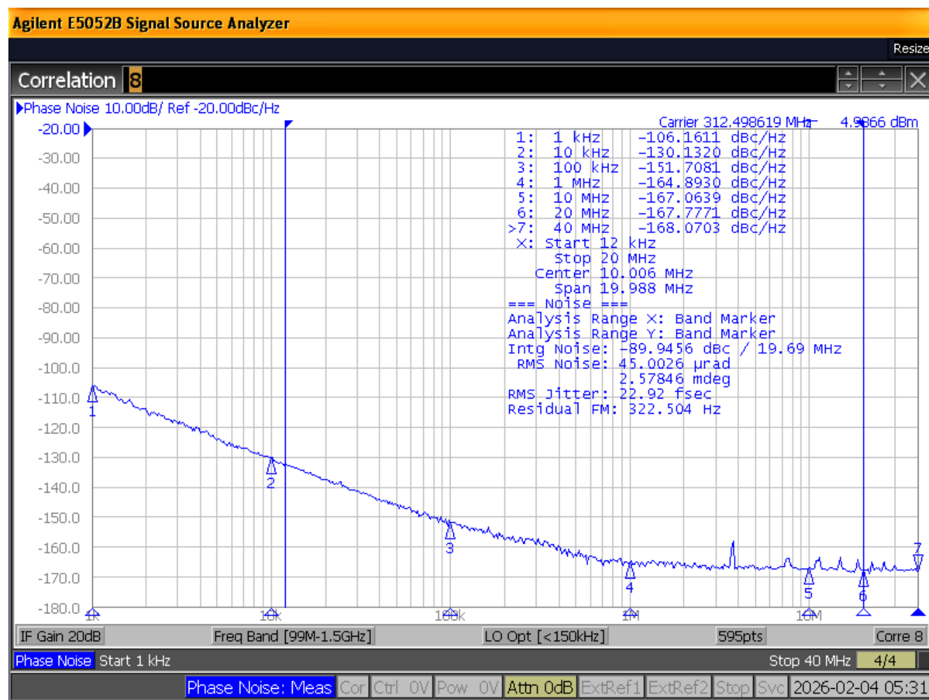
图 4-4. 312.5MHz LMK6L 型号的相位噪声图
