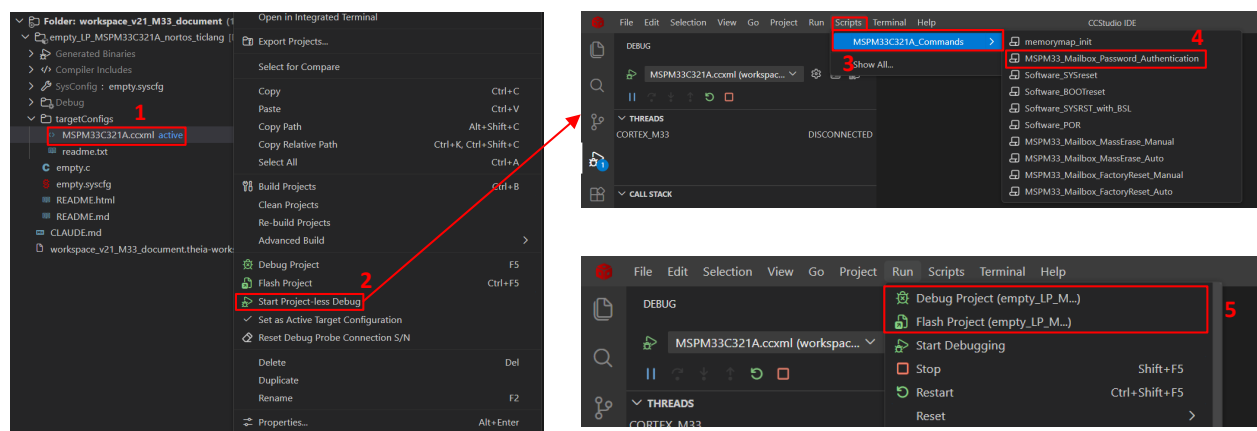
图 6-6. 使用 CCS v21 的 DSSM 命令
