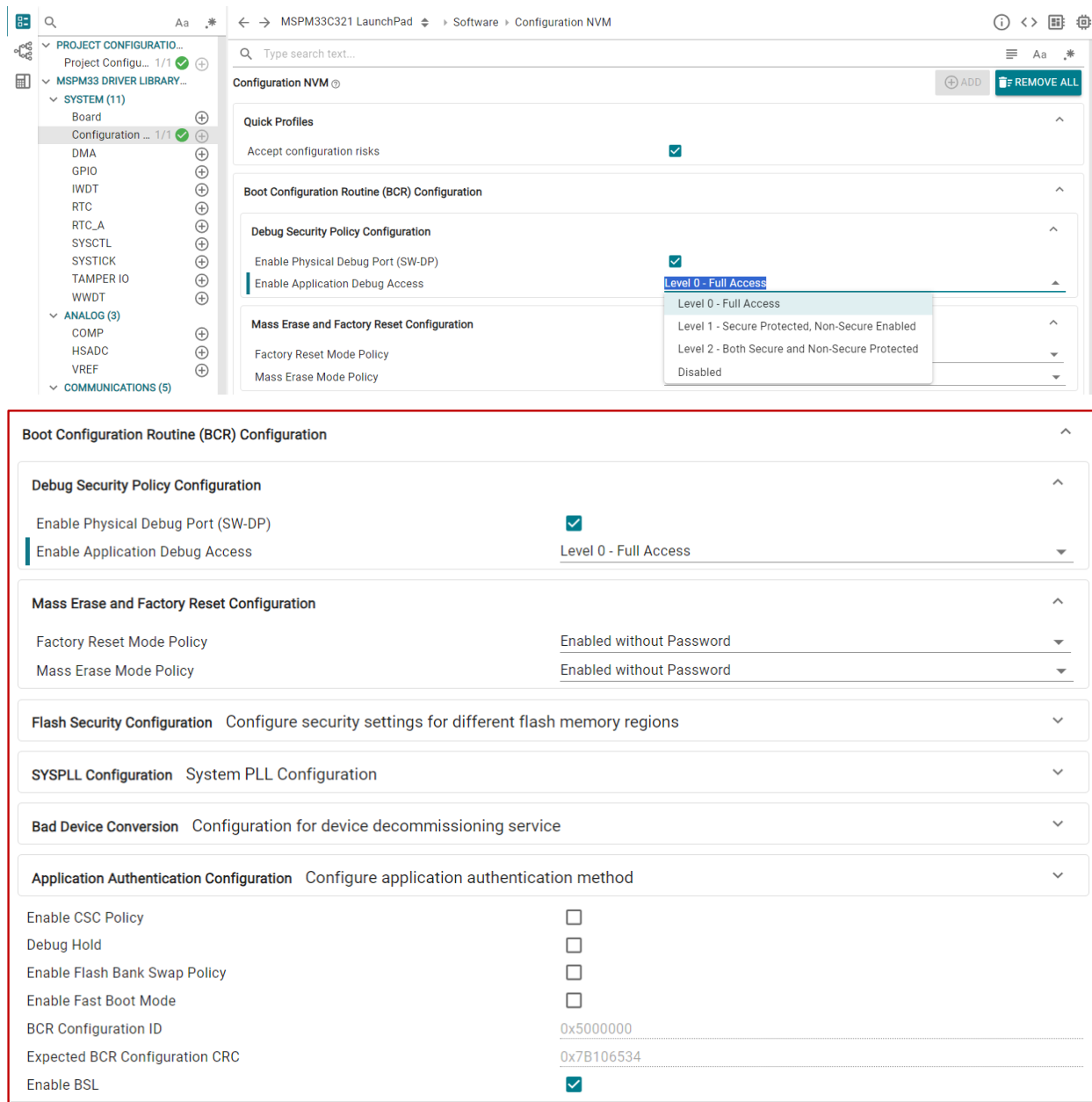
图 4-2. BCR 配置
