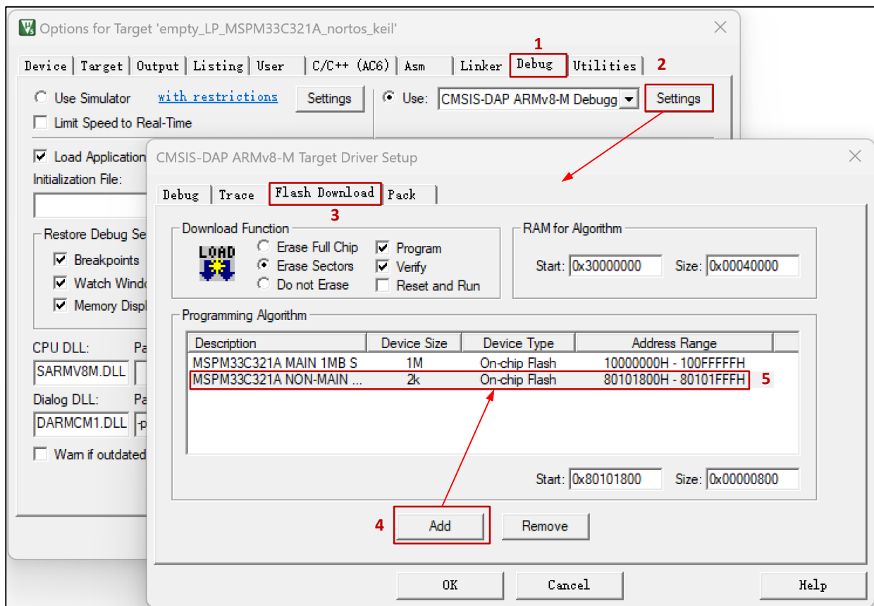
图 6-3. Keil 擦除属性设置
