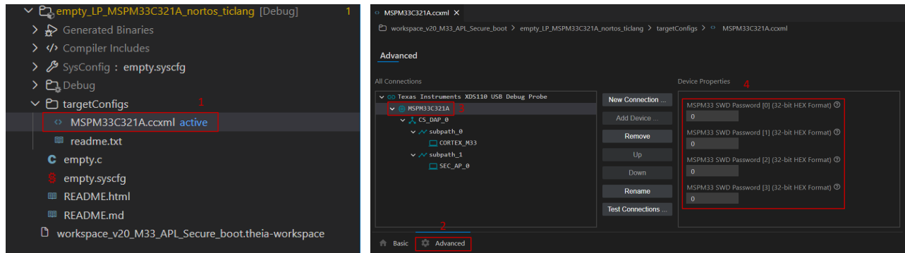
图 6-5. 使用 .ccxml 文件设置密码
