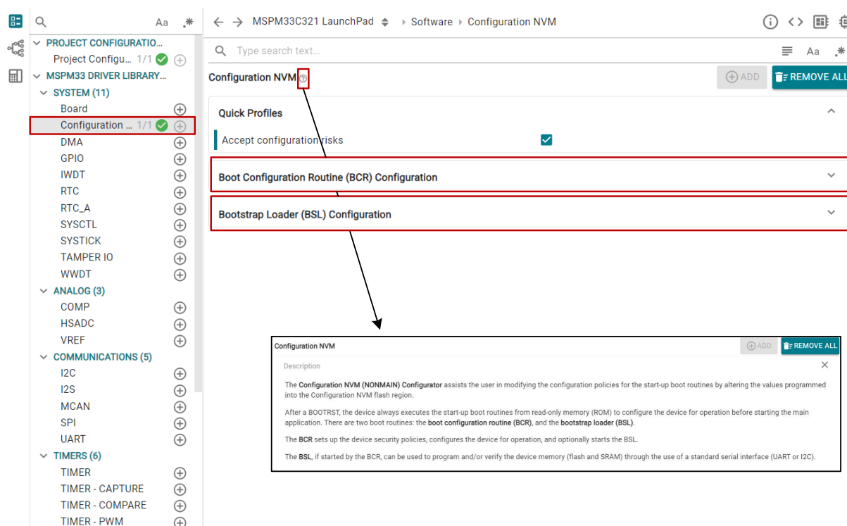
图 4-1. SysConfig 工具：配置 NVM
