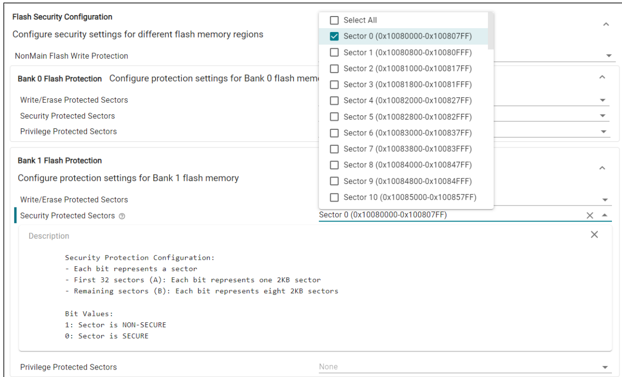
图 4-8. 闪存安全保护
