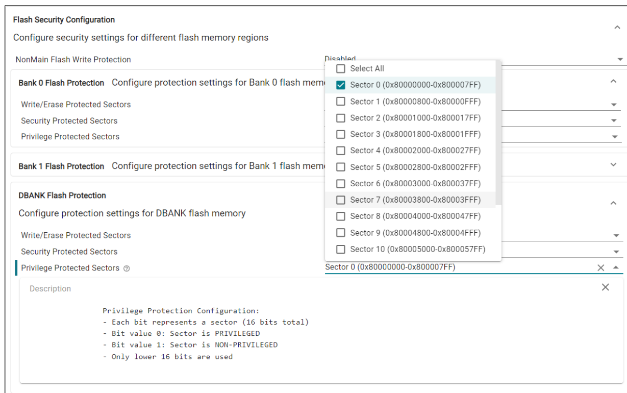
图 4-9. 闪存特权保护
