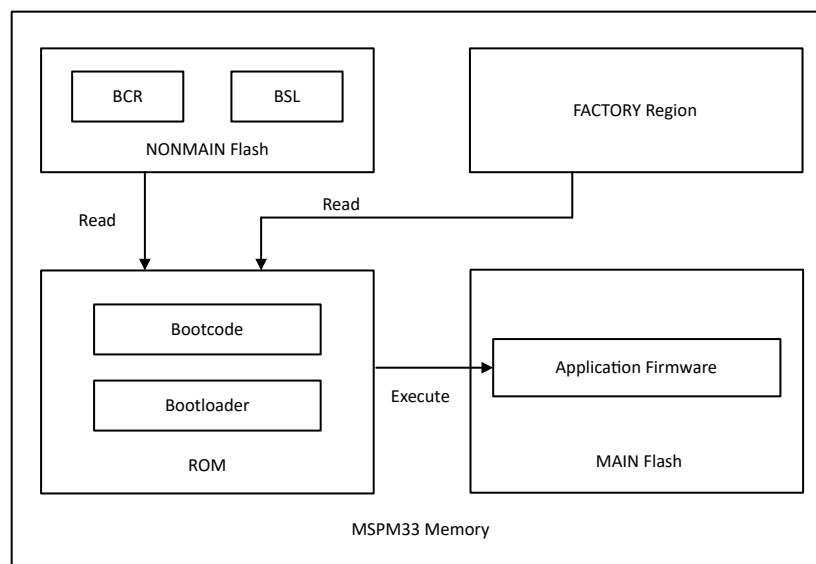
图 1-1. MSPM33 存储器映射
