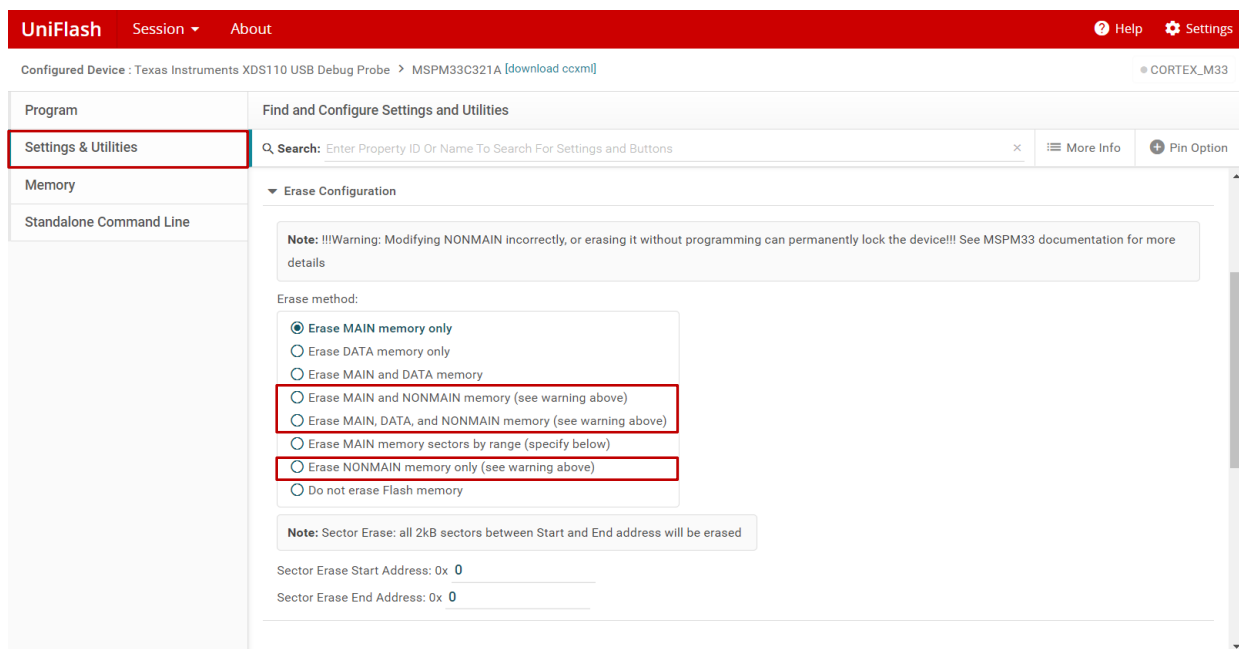
图 7-1. 使用 UniFlash 进行 NONMAIN 操作
