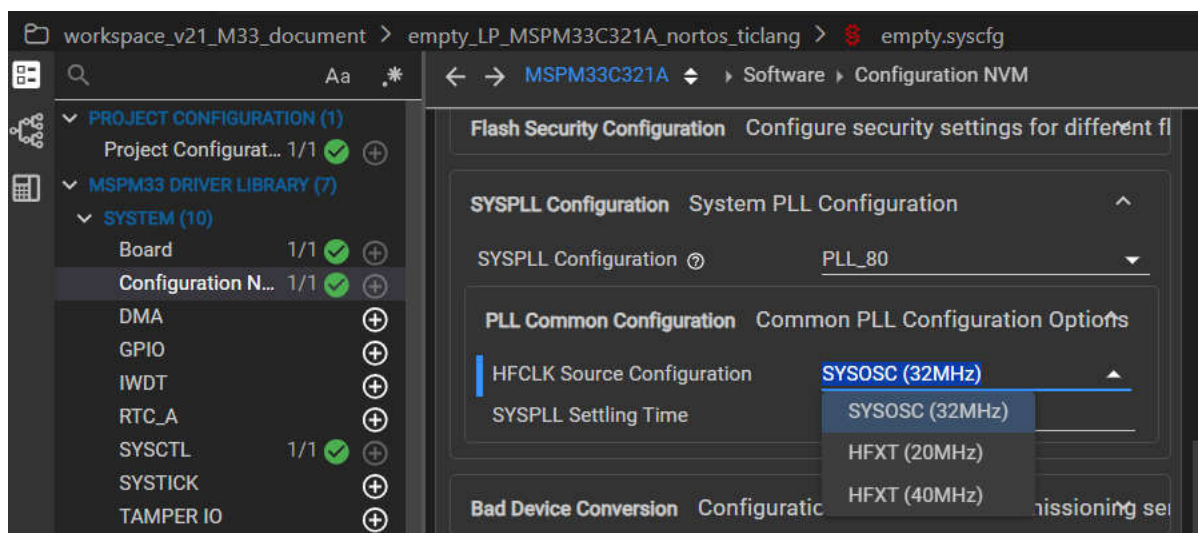
图 4-6. HFCLK 源配置
