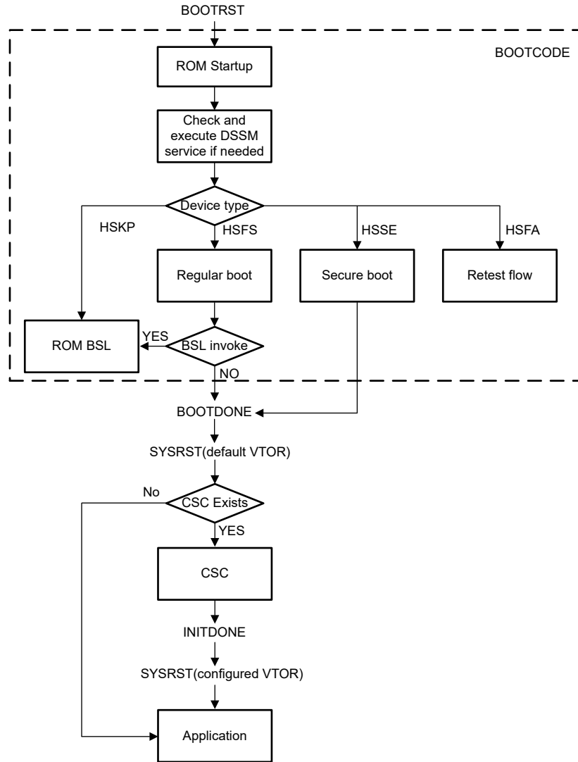
图 3-1. 安全引导和启动序列
