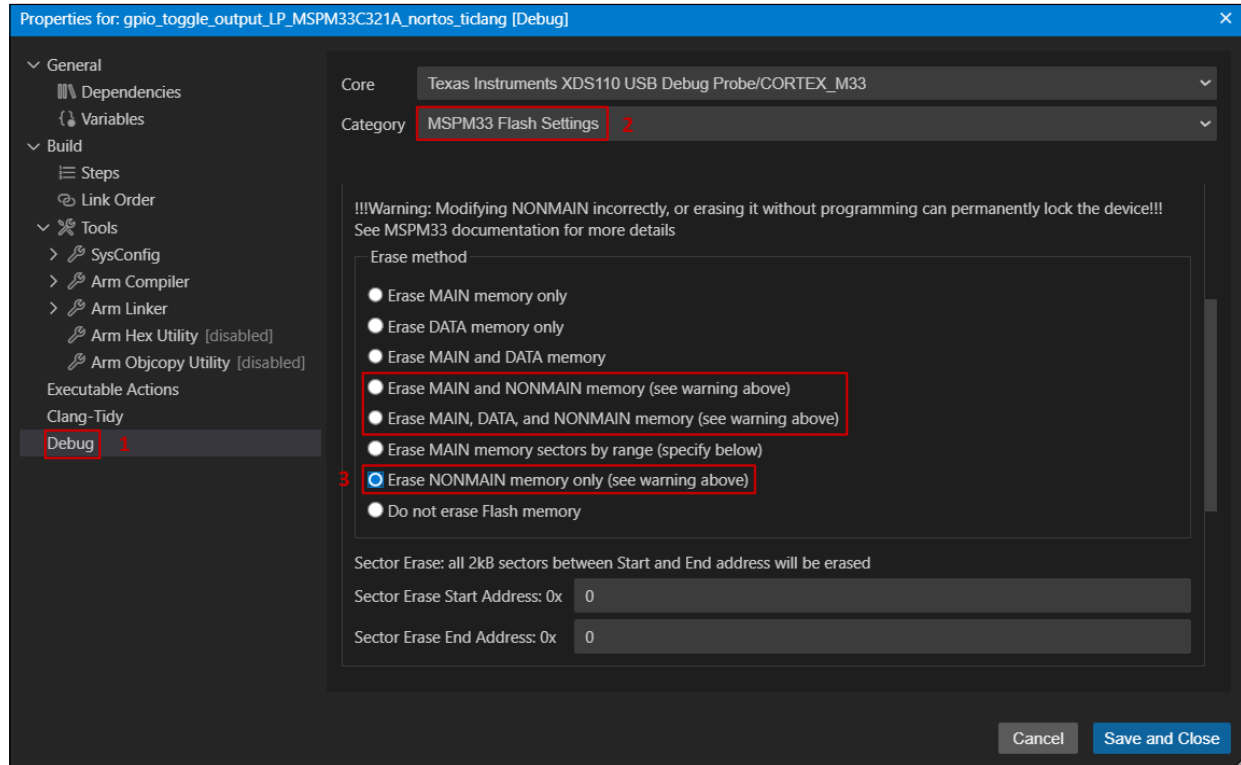
图 6-2. CCS 擦除属性设置
