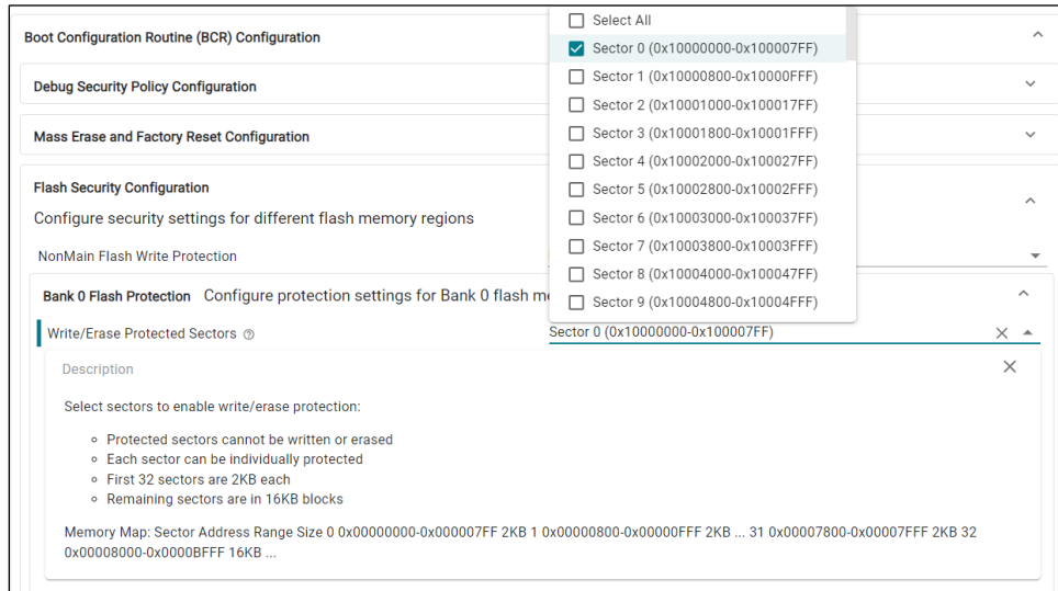
图 4-7. 闪存静态写保护
