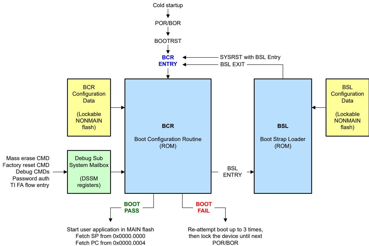
图 1-2. MSPM33 启动流程
