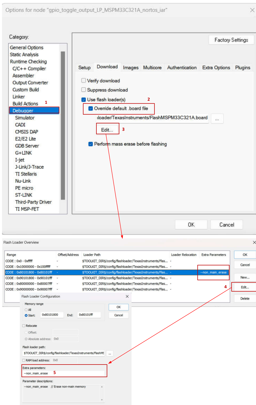
图 6-4. IAR 擦除属性设置
