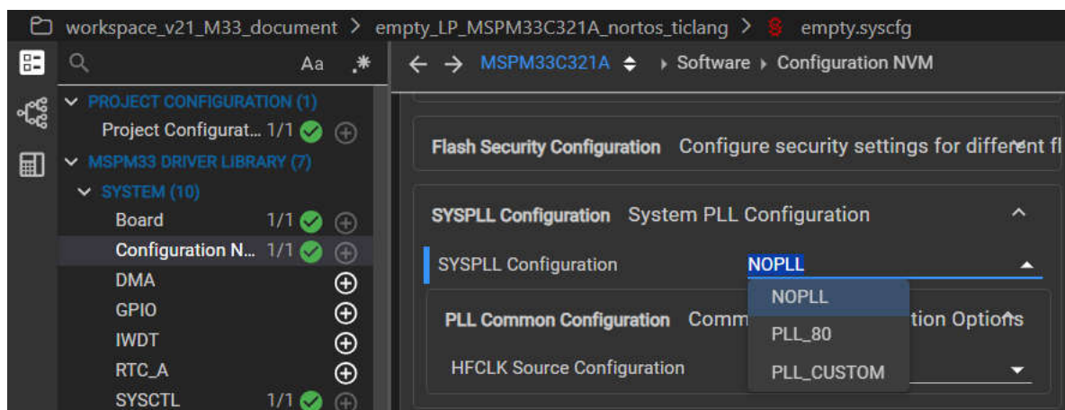
图 4-5. SYSPLL 配置
