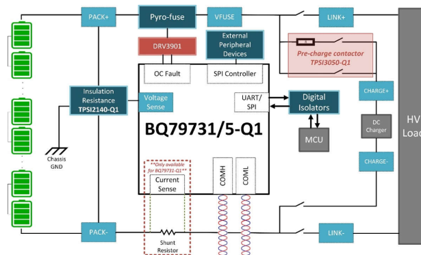
图 5. 简化版 BJB 系统方框图。
