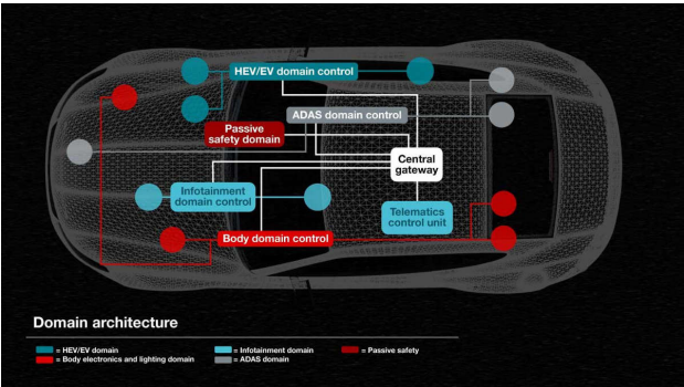
图 1. 域控制架构。
