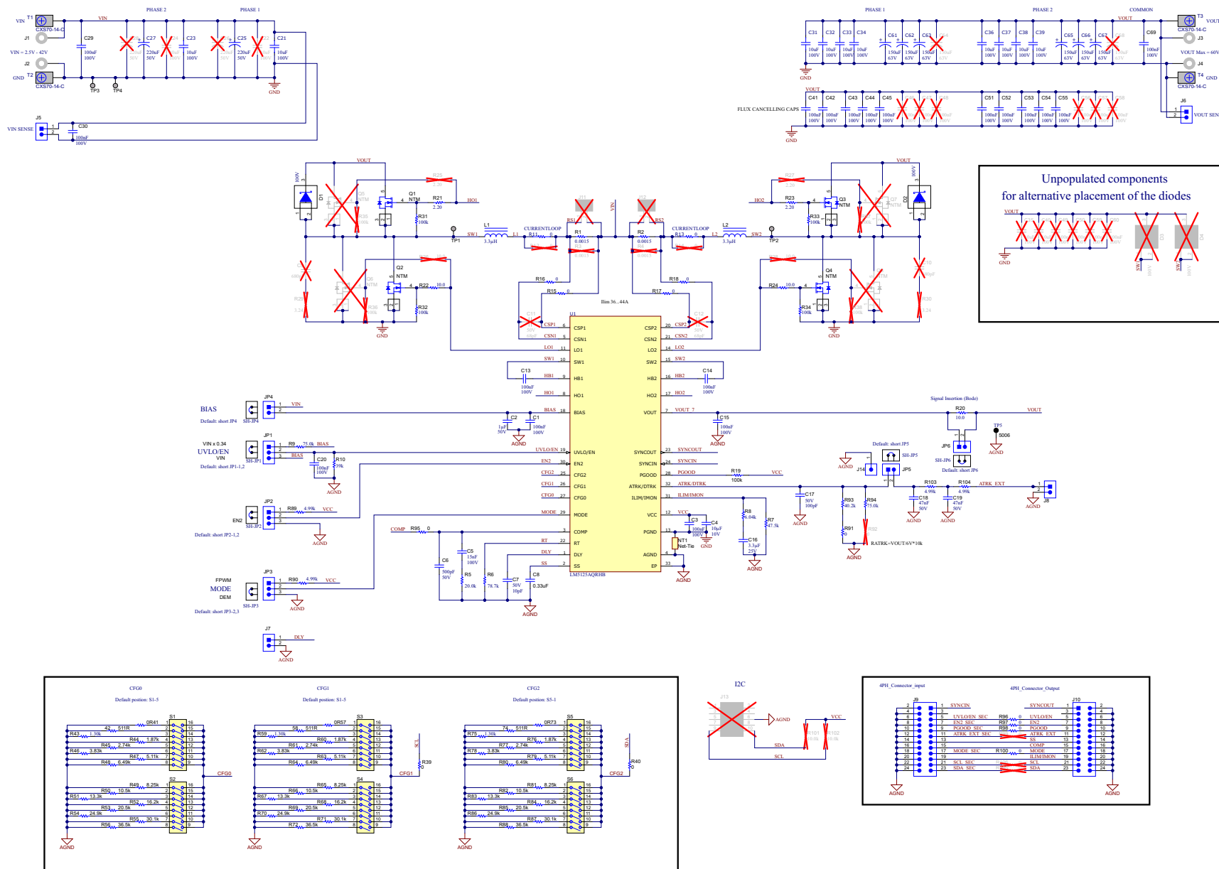
图 4-1. 原理图
