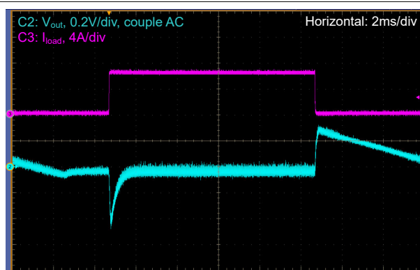
图 3-9. 负载瞬态, V_{in} = 14.4V , V_{out} = 24V , DEM, I_{load} = 0A 至 6.25A , 1A/\mu s
