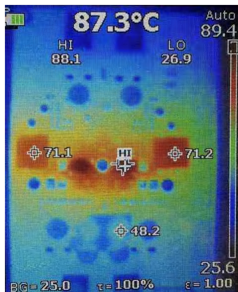
图 3-12. V_{in} = 14.4V , V_{out} = 45V , P_{OUT} = 240W , 自然对流
