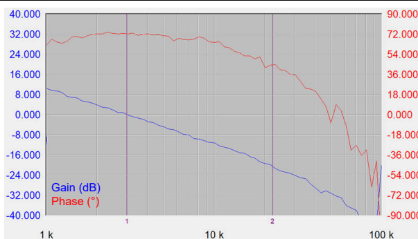
图 3-10. 波特图、 V_{in}=14.4V 、 V_{out}=40V 、 I_{out}=10A (平均电流环路已禁用)
