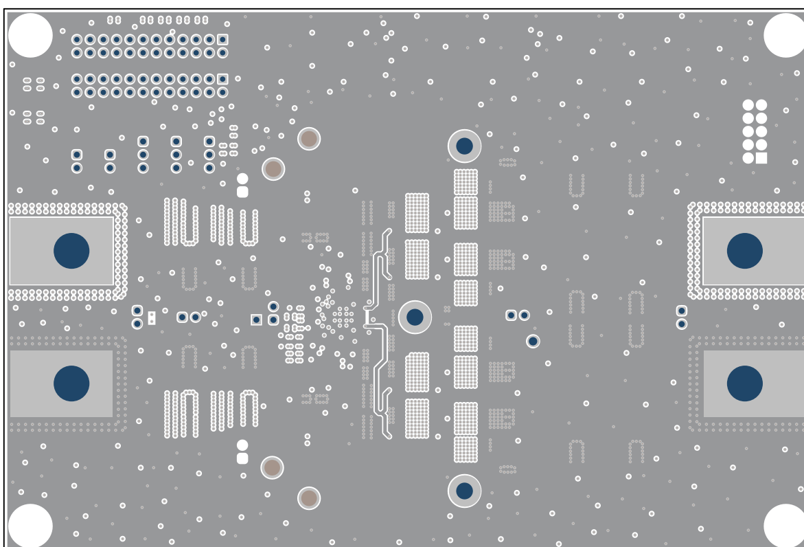
图 4-5. 信号层 1
