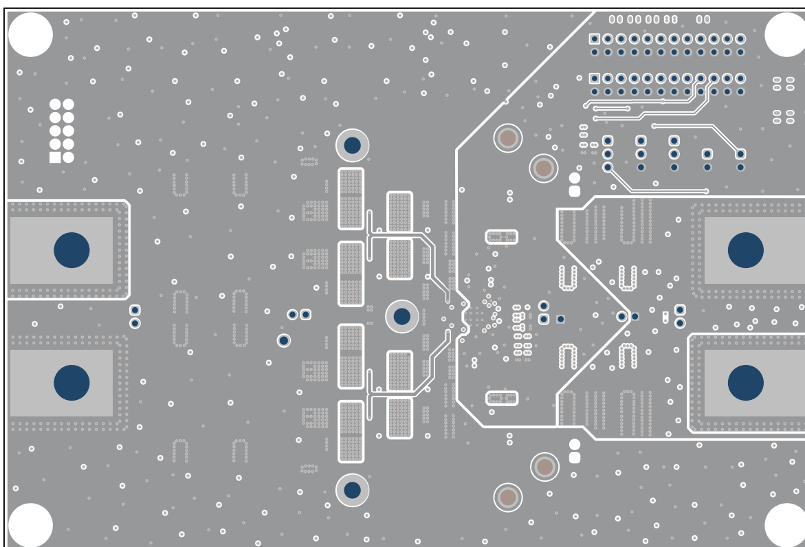
图 4-9. 底层
