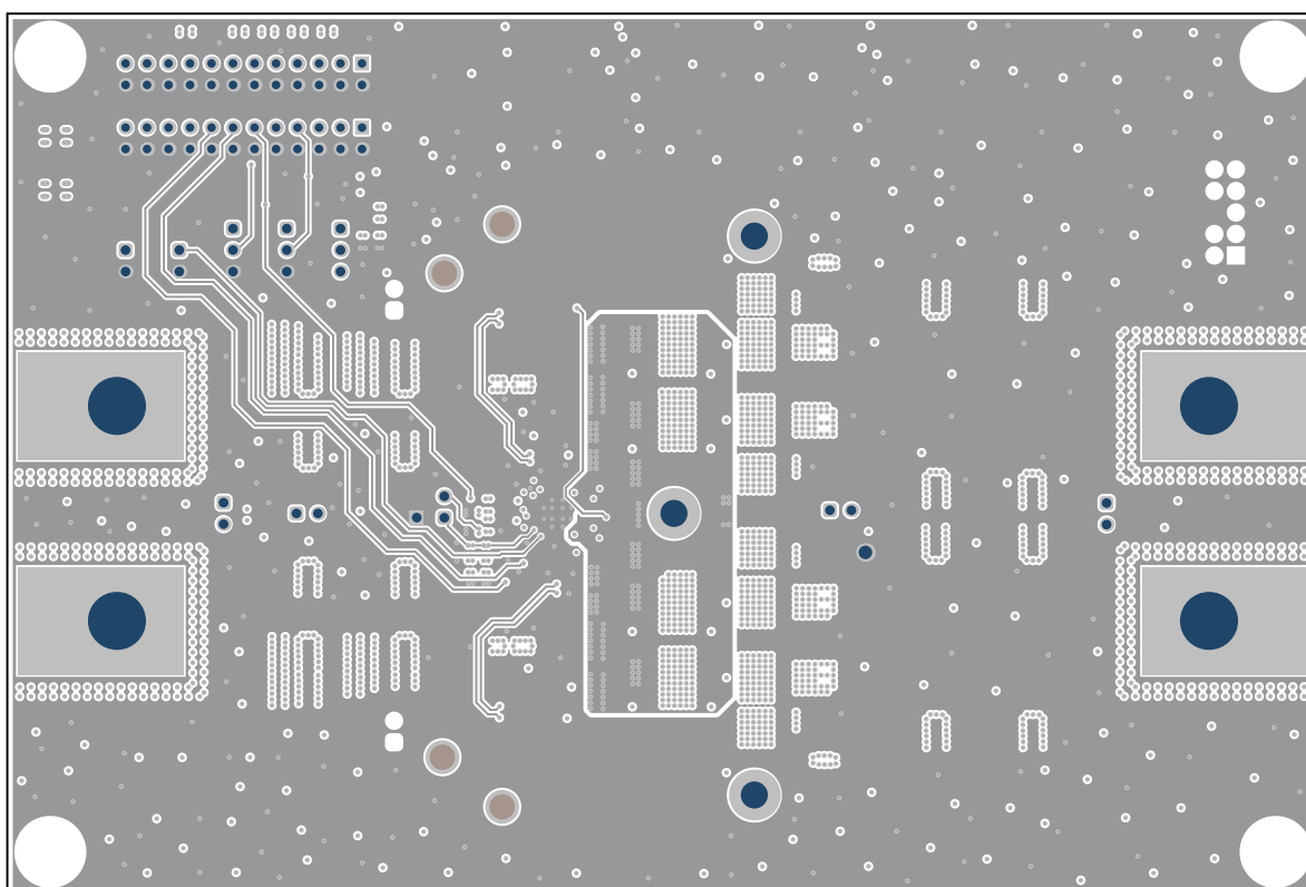
图 4-7. 信号层 3
