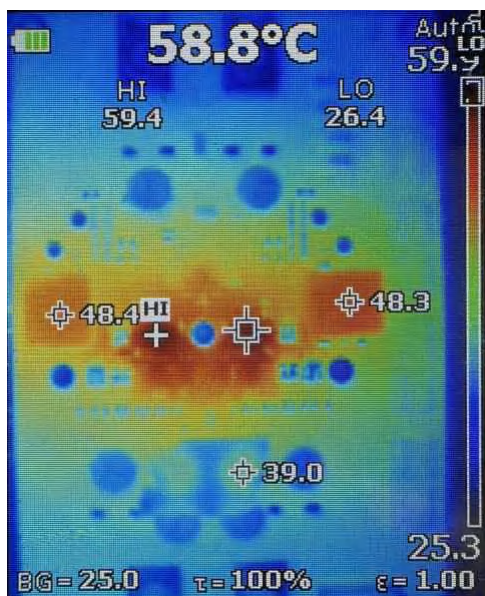
图 3-11. V_{in} = 14.4V , V_{out} = 24V , P_{OUT} = 240W , 自然对流
