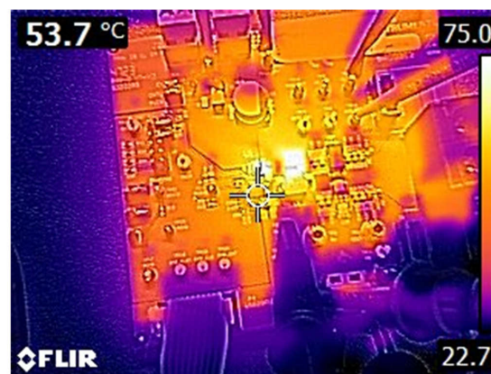
图 4-28. 热特性，1.2MHz，FCCM，外部 5V 辅助电源，20A 负载，无气流，浸泡 10 分钟
