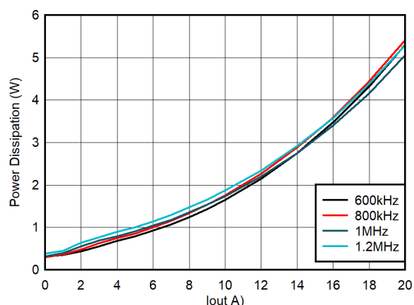
图 4-4. 功率耗散, FCCM, 外部 5V 辅助电源
