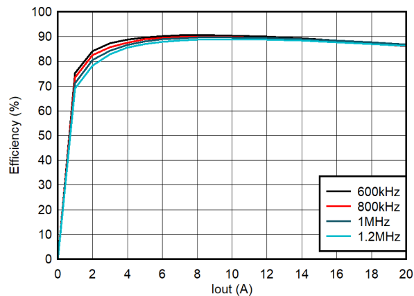
图 4-1. 效率, FCCM, 内部 LDO
