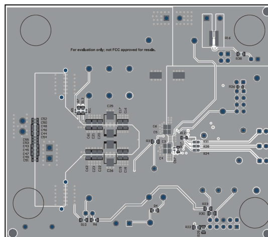
图 5-3. TPS544B27EVM 底部复合视图
