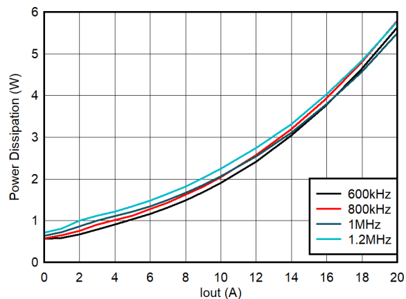
图 4-2. 功率耗散, FCCM, 内部 LDO
