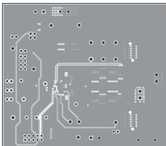
图 5-6. TPS544B27EVM 第 3 层
