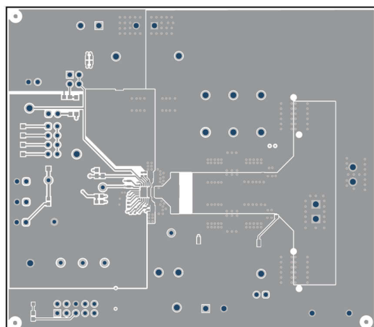
图 5-4. TPS544B27EVM 顶层
