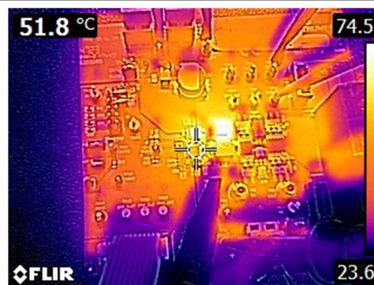
图 4-26. 热特性，1MHz FCCM，外部 5V 辅助电源，20A 负载，无气流，浸泡 10 分钟
