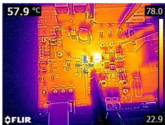
图 4-27. 热特性，1.2MHz，FCCM，内部 LDO，20A 负载，无气流，浸泡 10 分钟
