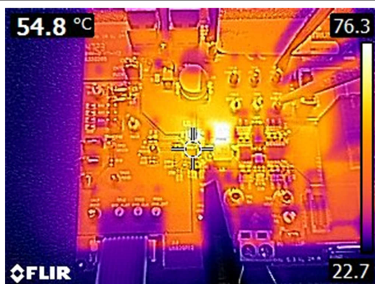
图 4-25. 热特性，1MHz FCCM，内部 LDO，20A 负载，无气流，浸泡 10 分钟
