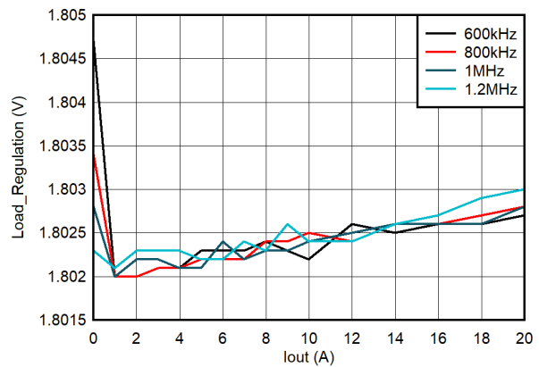
图 4-12. 负载调节，DCM，外部 5V 辅助电源
