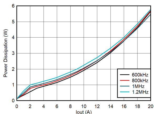
图 4-6. 功率耗散, DCM, 内部 LDO
