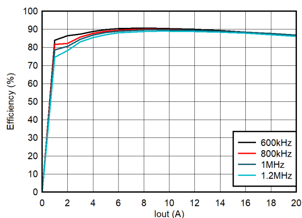
图 4-5. 效率, DCM, 内部 LDO
