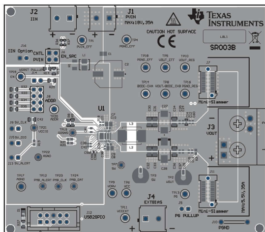
图 5-2. TPS544B27EVM 顶部复合视图
