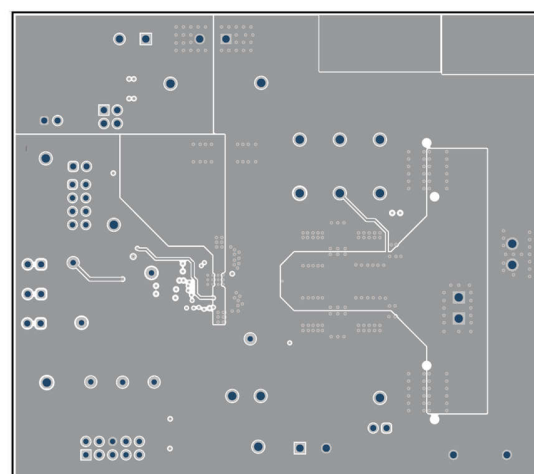
图 5-7. TPS544B27EVM 第 4 层
