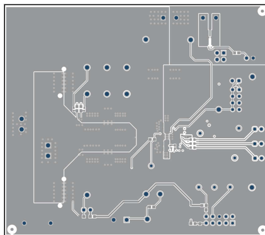
图 5-9. TPS544B27EVM 底层
