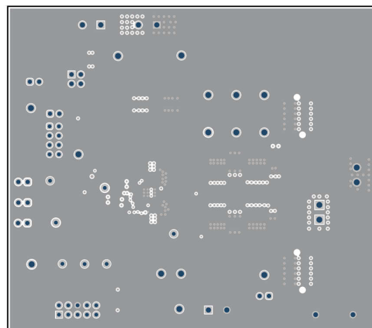
图 5-5. TPS544B27EVM 第 2 层
