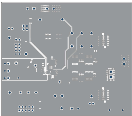
图 5-8. TPS544B27EVM 第 5 层
