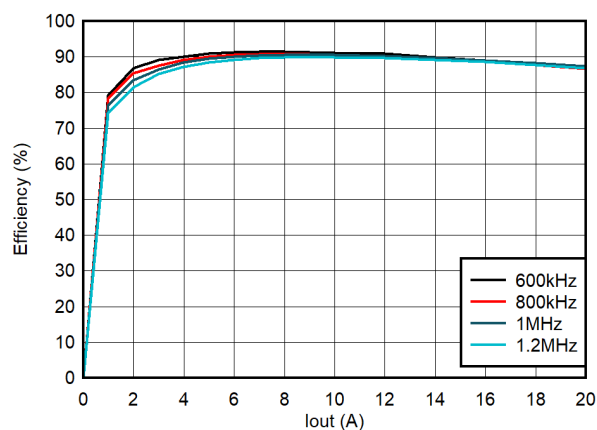
图 4-3. 效率, FCCM, 外部 5V 辅助电源
