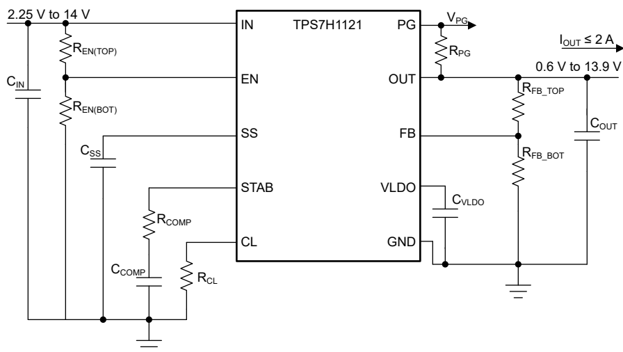
图 1-1. 简化版原理图
