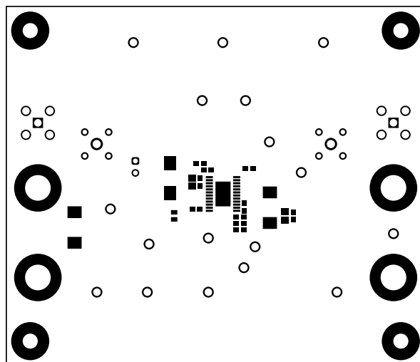
图 4-3. 顶部阻焊层
