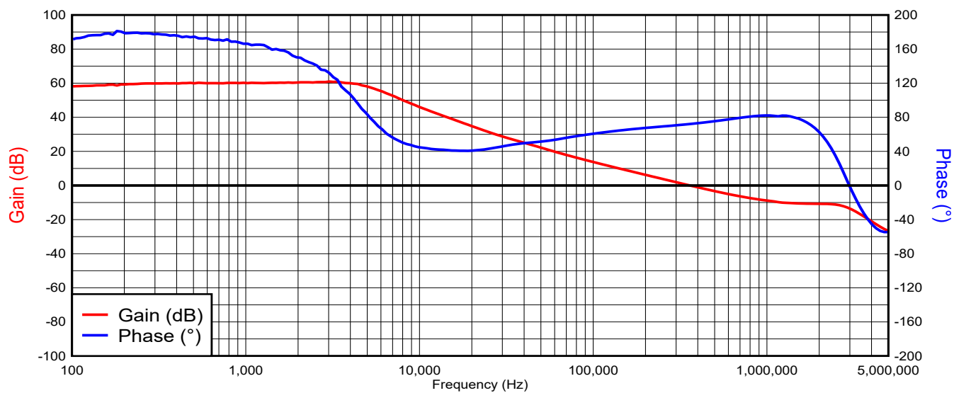
图 3-5. 频率响应 - I_{OUT} = 2\text{ A}
