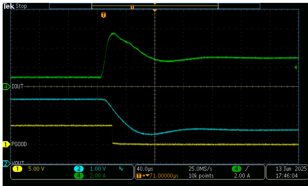
图 3-3. 电流限制生效 - 3.3\ \Omega 至 0.55\ \Omega 阶跃
