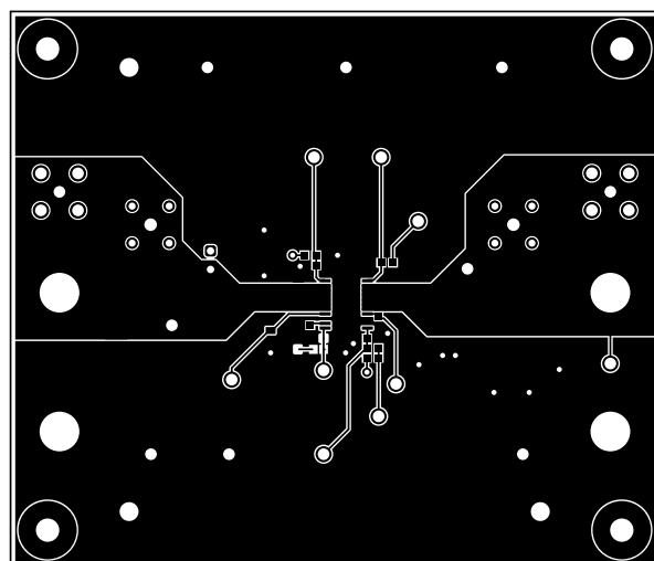
图 4-4. 第 1 层 (顶部)
