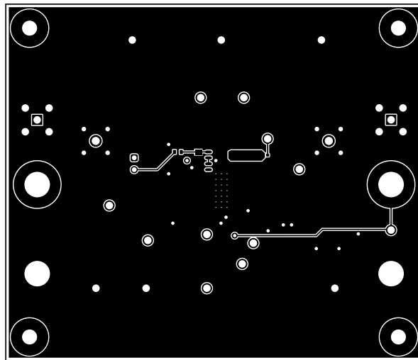
图 4-7. 第 3 层 (底部)
