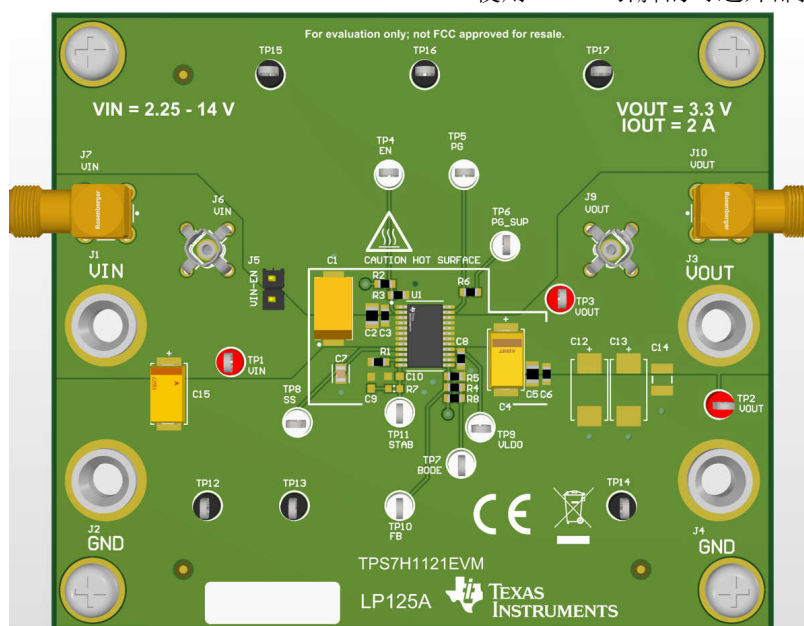
EVM 板
