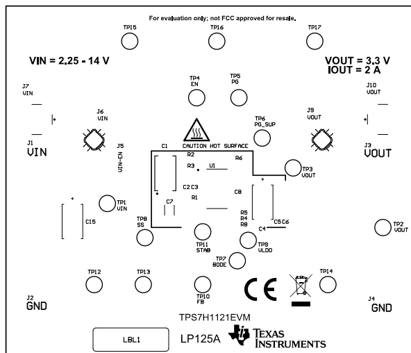
图 4-2. 顶层丝印层
