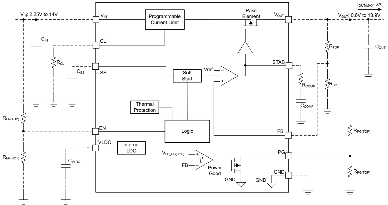
图 1-2. 功能方框图
