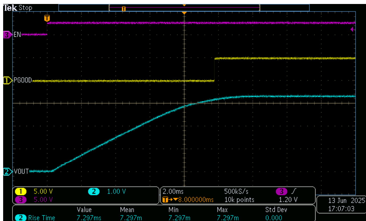
图 3-1. 软启动至 1.65 \Omega 负载
