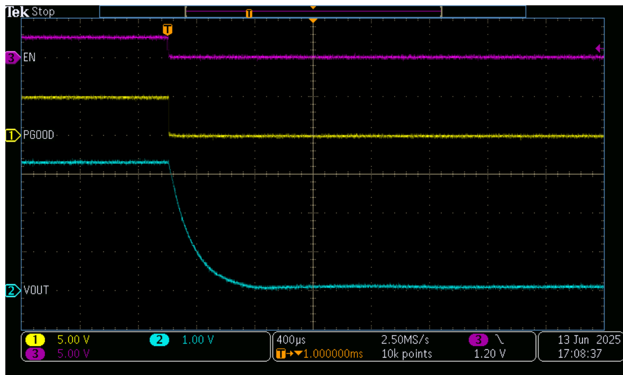
图 3-2. 关断至 3.3\ \Omega 负载
