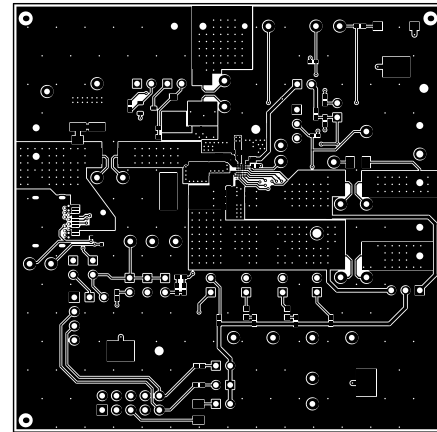
图 4-5. BMS077 顶层
