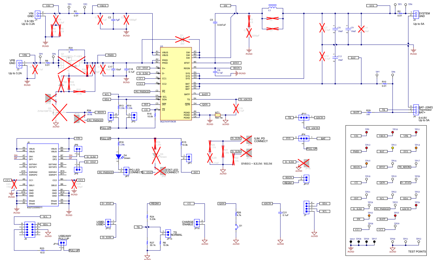
图 4-1. BQ25630EVM 原理图
