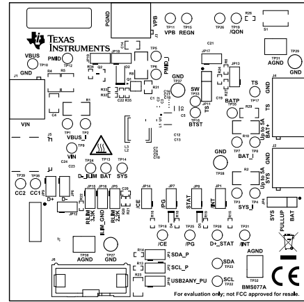
图 4-3. BMS077 顶部丝印
