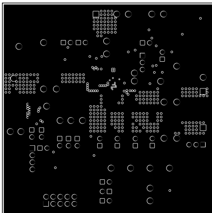
图 4-6. BMS077 信号层 1
