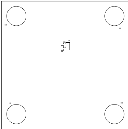
图 4-4. BMS077 底部覆盖层
