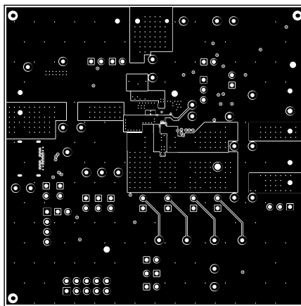
图 4-8. BMS077 底层
