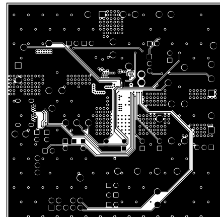
图 4-7. BMS077 信号层 2
