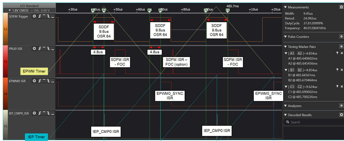
图 4-17. FOC 时序验证
