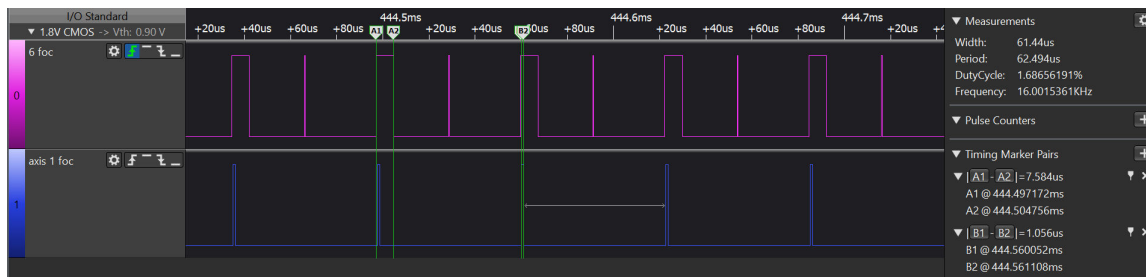
图 4-18. 6 轴 FOC 环路处理时间
