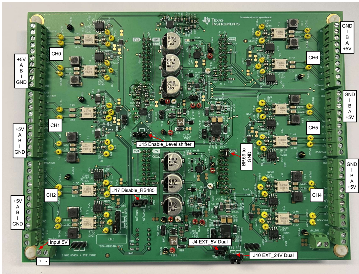
图 4-12. 位置板设置
