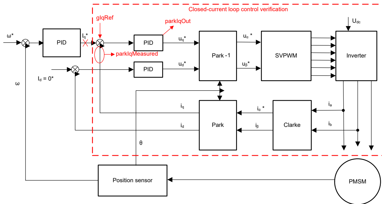
图 4-19. 具有 PI 控制器的闭合电流环路验证图
