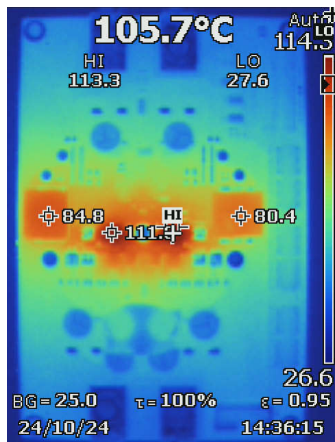
图 3-11. V_{in} = 14.4V , V_{out} = 45V , P_{OUT} = 300W , 自然对流
