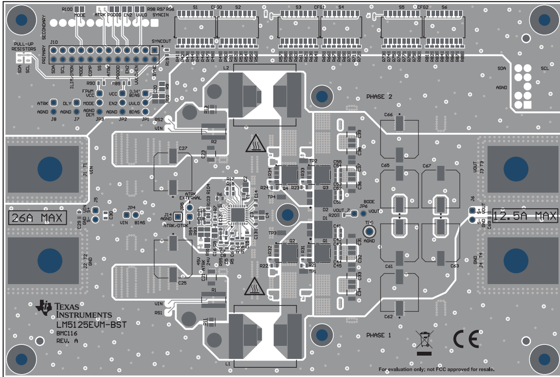
图 4-2. 顶部丝网印刷层
