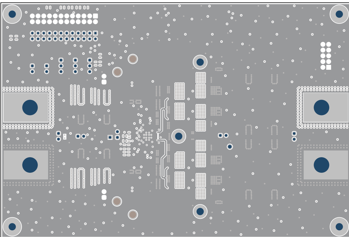
图 4-5. 信号层 1
