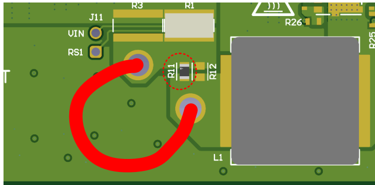
图 2-2. 观测 L1 电感器电流
