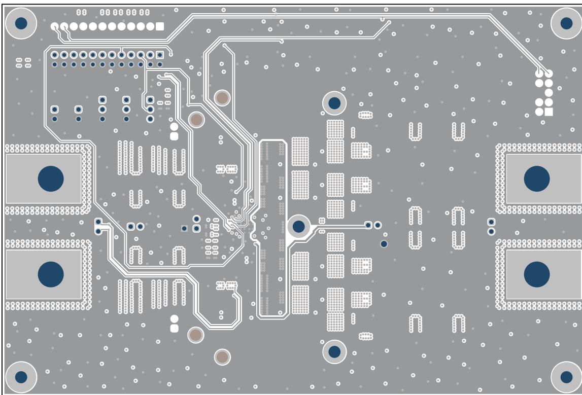
图 4-6. 信号层 2
