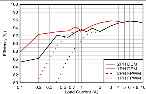
图 3-3. 效率与输出电流间的关系, V_{in} = 14.4V , V_{out} = 45V
