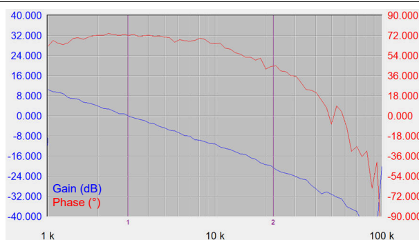
图 3-9. 波特图、 V_{in}=14.4V 、 V_{out}=40V 、 I_{out}=10A (平均电流环路已禁用)
