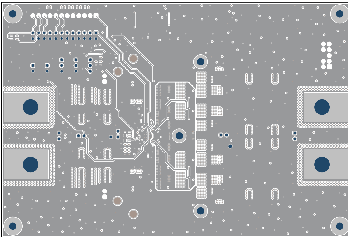
图 4-8. 信号层 4
