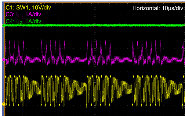
图 3-4. V_{in} = 14.4V , V_{out} = 24V , DEM, I_{load} = 0.1A
