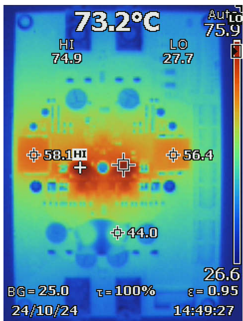
图 3-10. V_{in} = 14.4V , V_{out} = 24V , P_{OUT} = 300W , 自然对流
