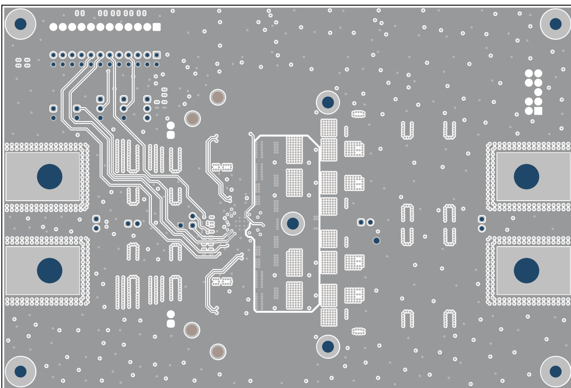
图 4-7. 信号层 3
