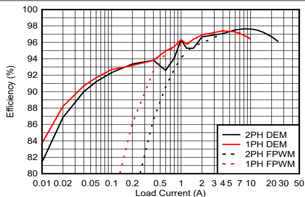
图 3-2. 效率与输出电流间的关系, V_{in} = 14.4V , V_{out} = 24V
