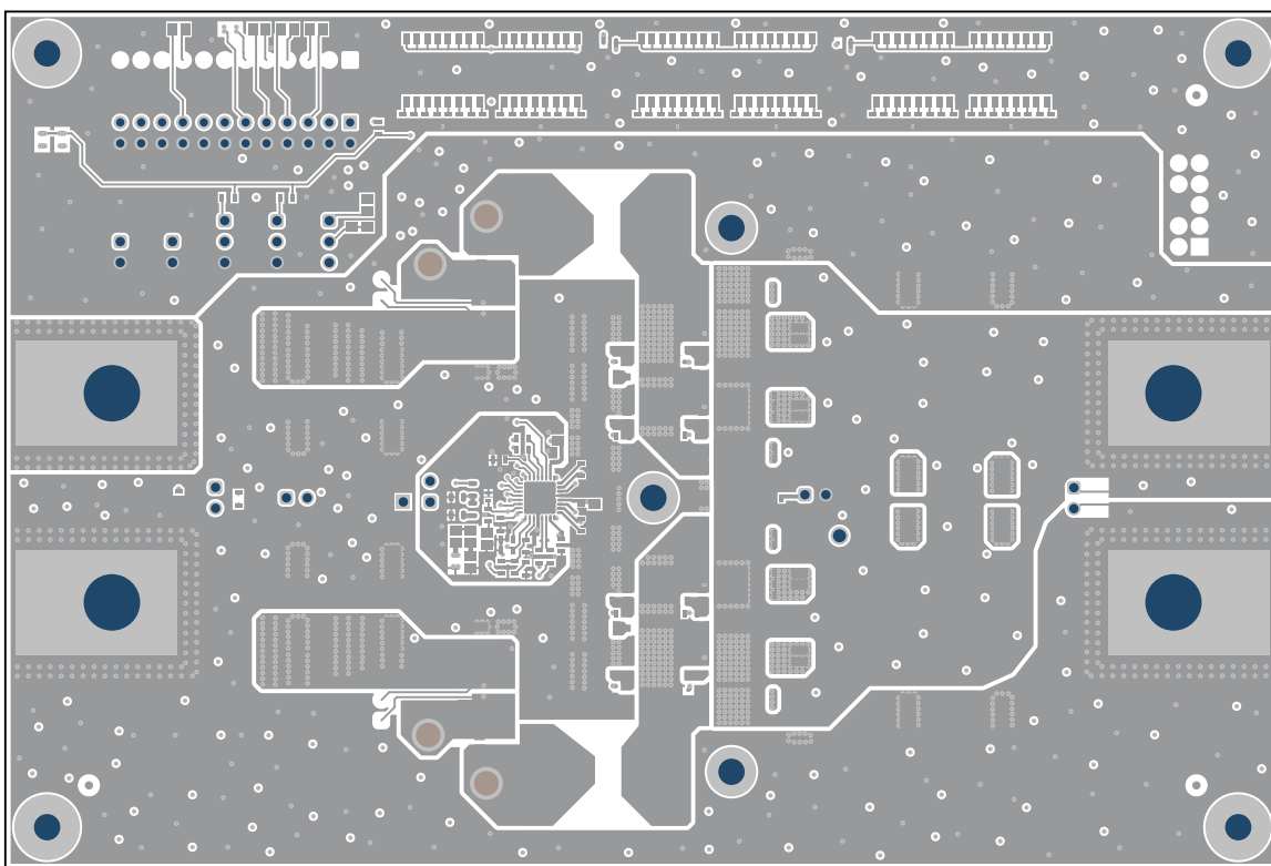
图 4-4. 顶层
