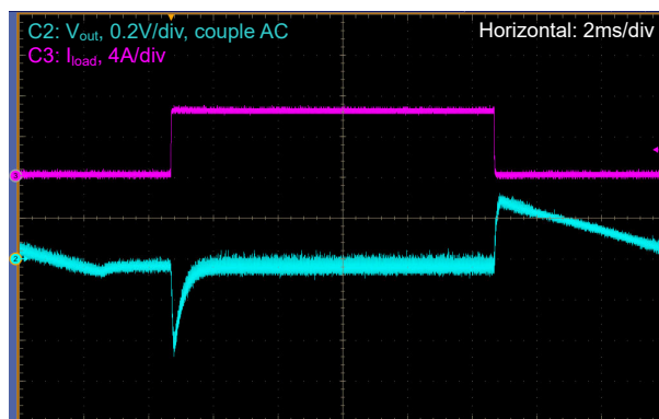
图 3-8. 负载瞬态, V_{in} = 14.4V , V_{out} = 24V , DEM, I_{load} = 0A 至 6.25A , 1A/\mu s
