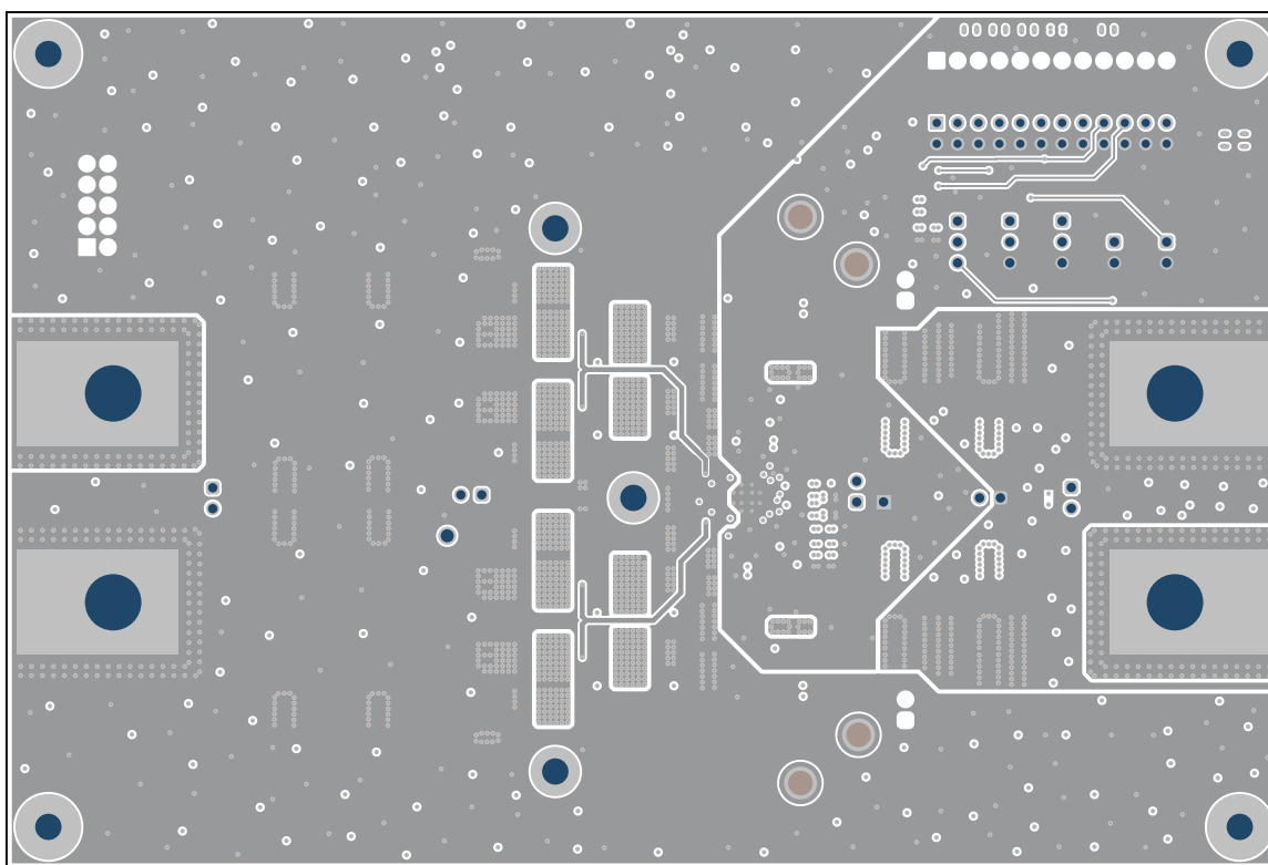
图 4-9. 底层
