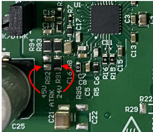
图 2-1. 选择 24V 和 45V 之间的 V_{out}
