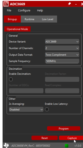
图 3-6. 使用 ADC3669 GUI 采集 ADC 数据
