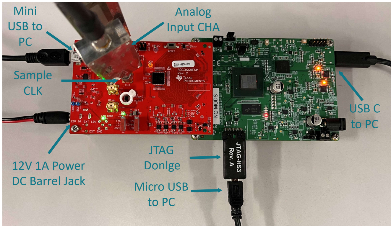
图 2-3. ADC3669EVM 的组装设置
