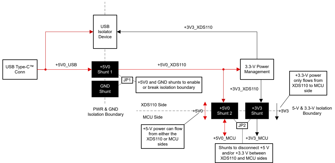
图 2-2. LaunchPad 配电图
