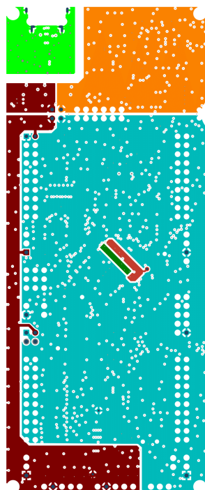
图 4-3. PWR - 第 3 层
