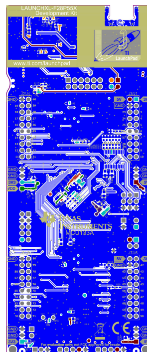
图 4-4. 底部信号 - 第 4 层
