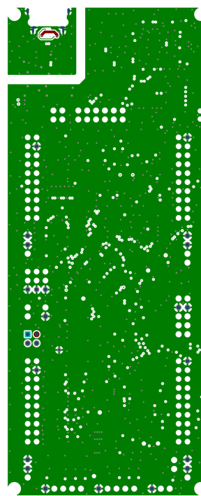
图 4-2. GND - 第 2 层
