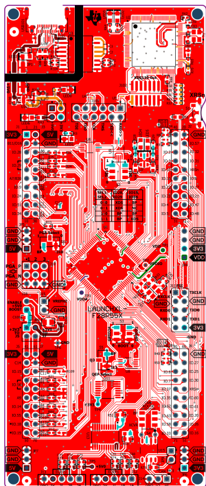
图 4-1. 顶部信号 - 第 1 层
