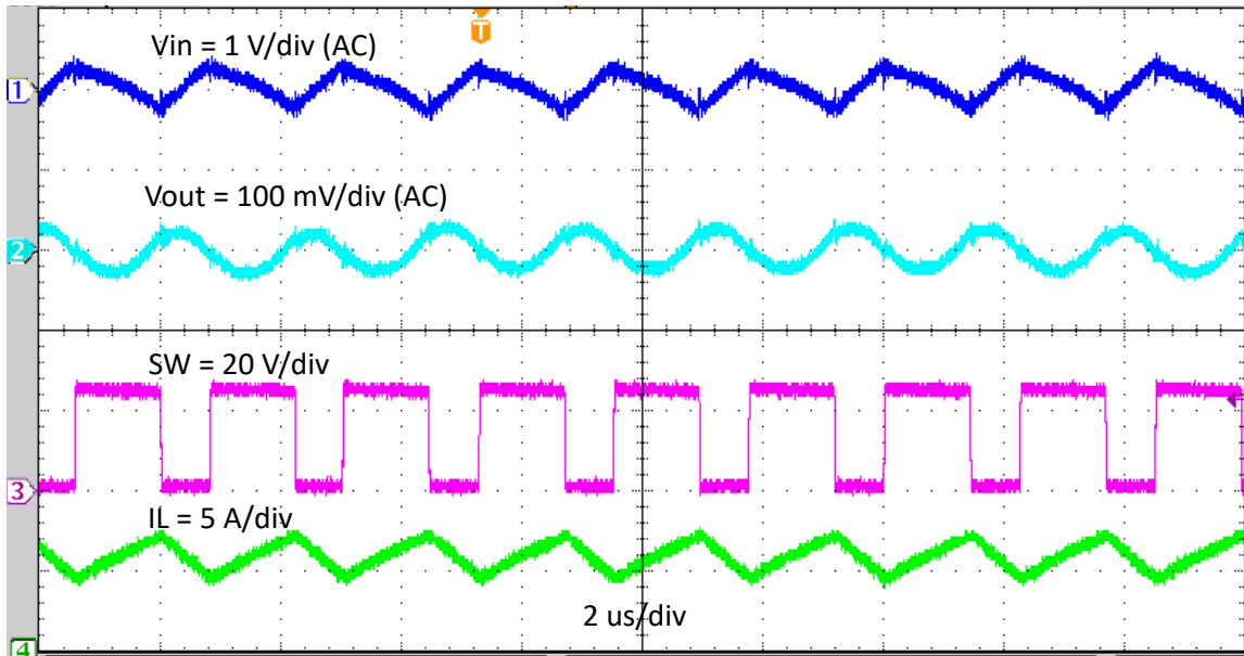
图 3-2. TPS56837HEVM 输出电压纹波 ( V_{IN} = 24V , I_{OUT} = 8A )
