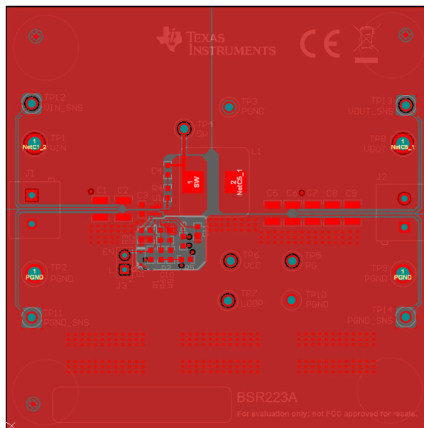
图 4-5. 顶层
