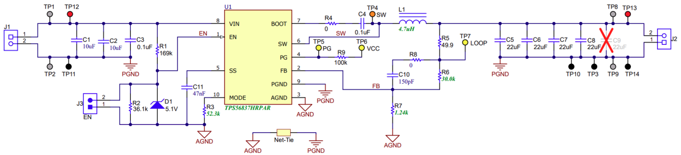
图 4-1. TPS56837HEVM 原理图
