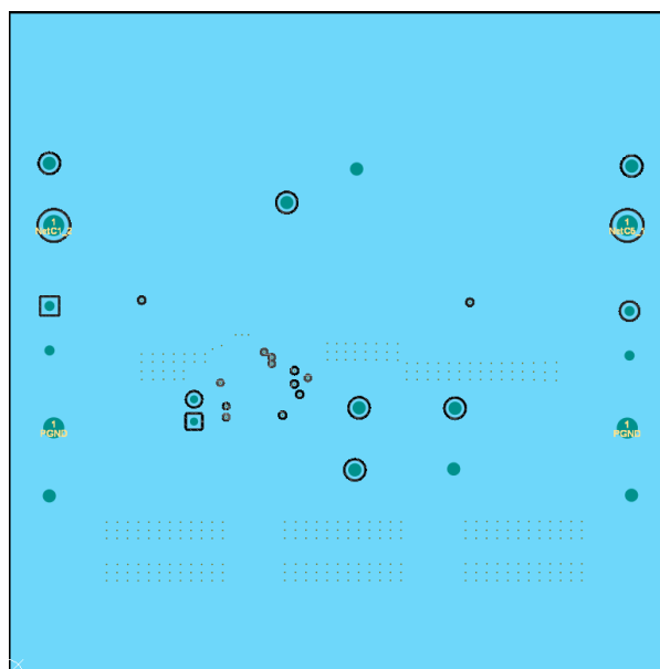
图 4-7. 中间层 2
