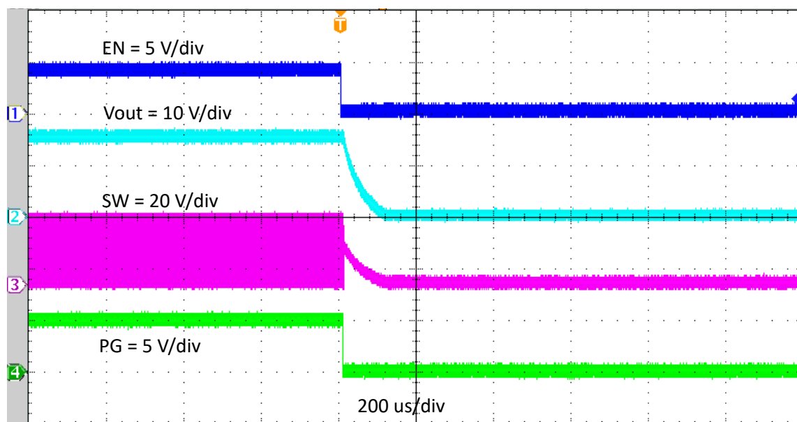
图 3-4. TPS56837HEVM 相对于 EN 的关断, I_{OUT} = 8A
