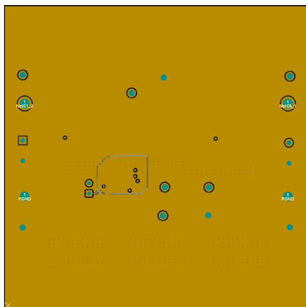
图 4-6. 中间层 1
