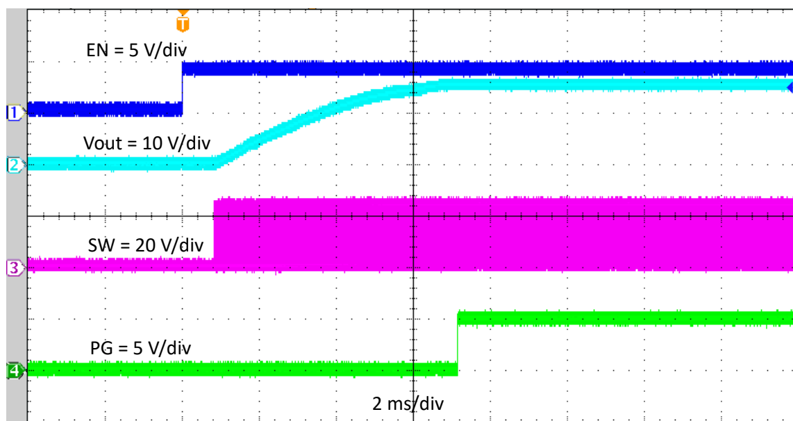
图 3-3. TPS56837HEVM 相对于 EN 的启动, I_{OUT} = 8A
