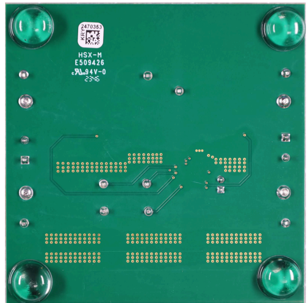
图 4-3. TPS56837HEVM 背面图
