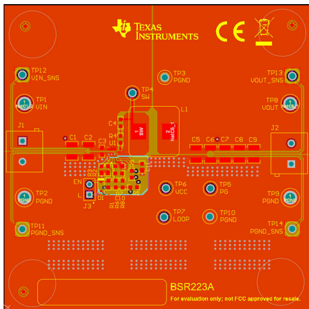
图 4-4. 顶层装配图
