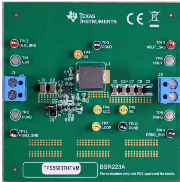
图 4-2. TPS56837HEVM 正面图
