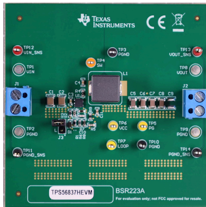
图 1-1. TPS56837HEVM (顶视图)
